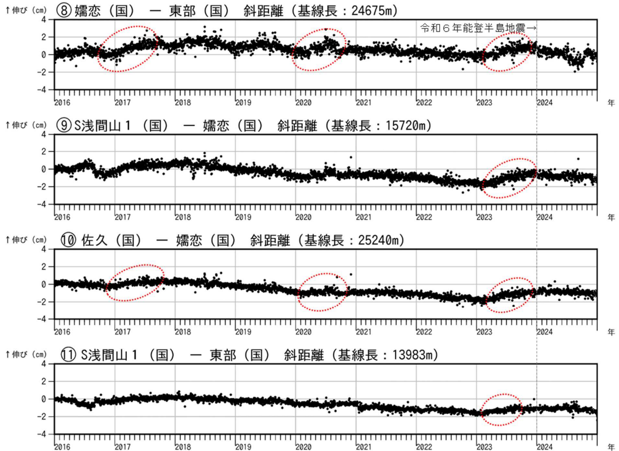
図7-2 浅間山 GNSS 連続観測結果(2016年1月1日～2024年12月31日)
