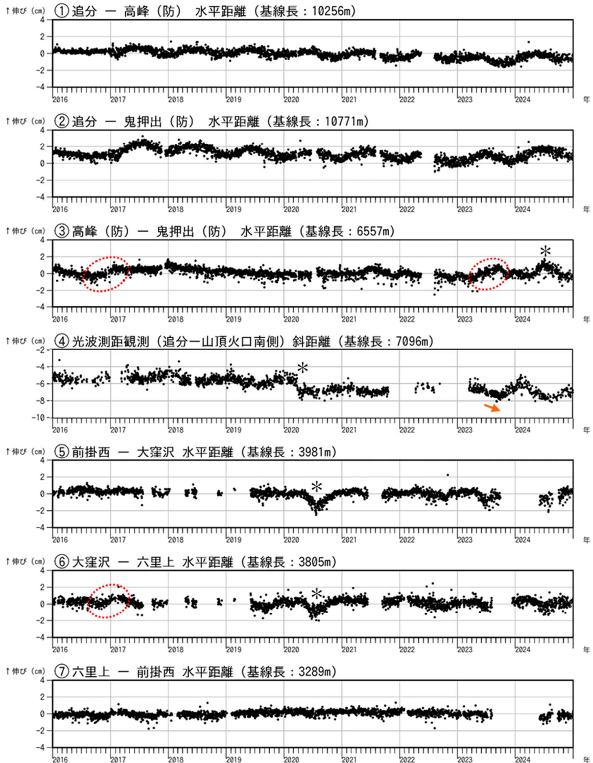
図7-1 浅間山 GNSS 連続観測及び光波測距観測結果(2016年1月1日~2024年12月31日)
