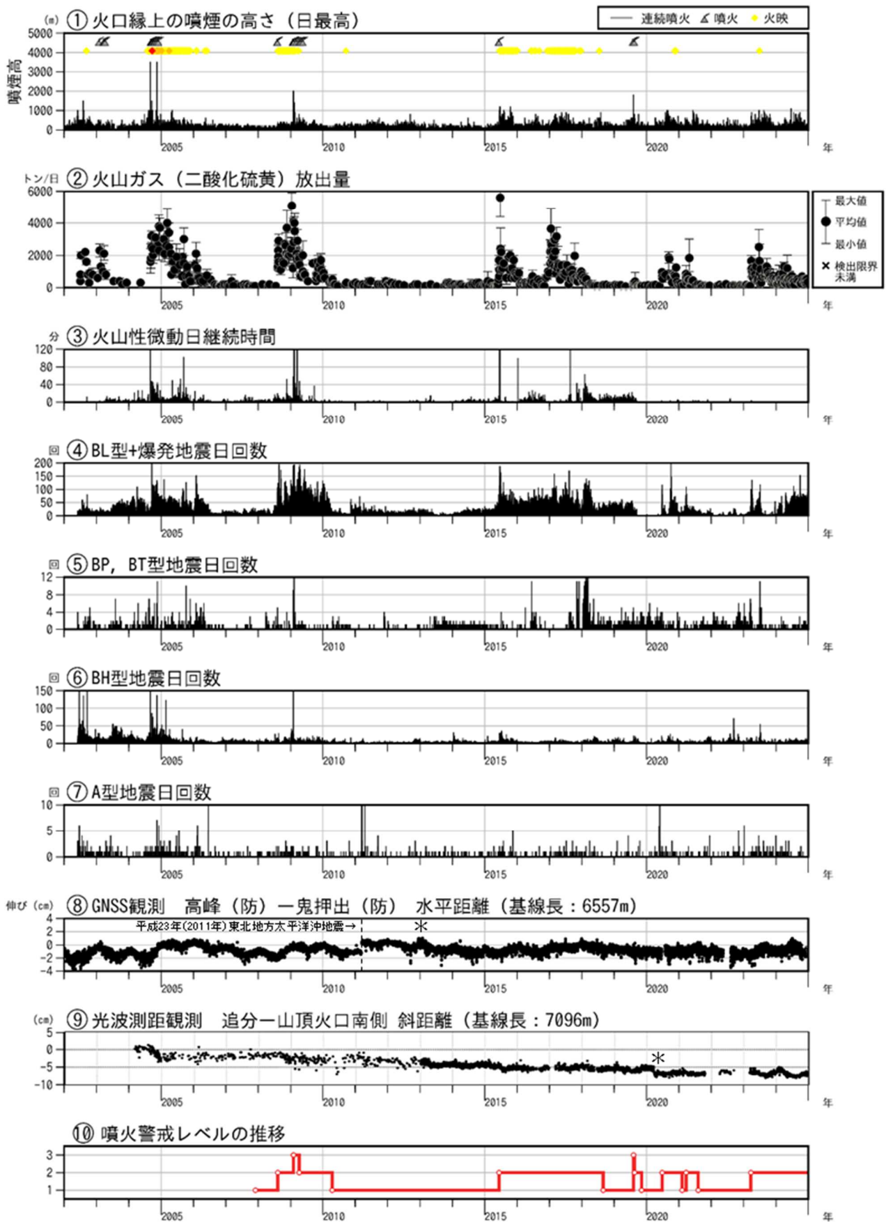
図3 浅間山 長期火山活動経過図（2002年1月1日～2024年12月31日）
