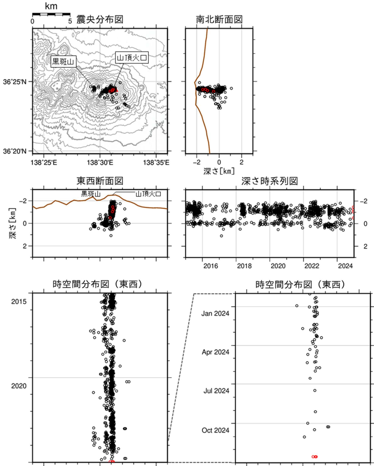
図5 浅間山 震源分布図（2015年1月1日～2024年12月31日）
