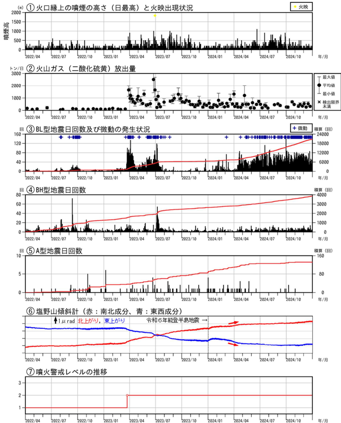
図2 浅間山 短期火山活動経過図（2022年4月1日～2024年12月31日）
