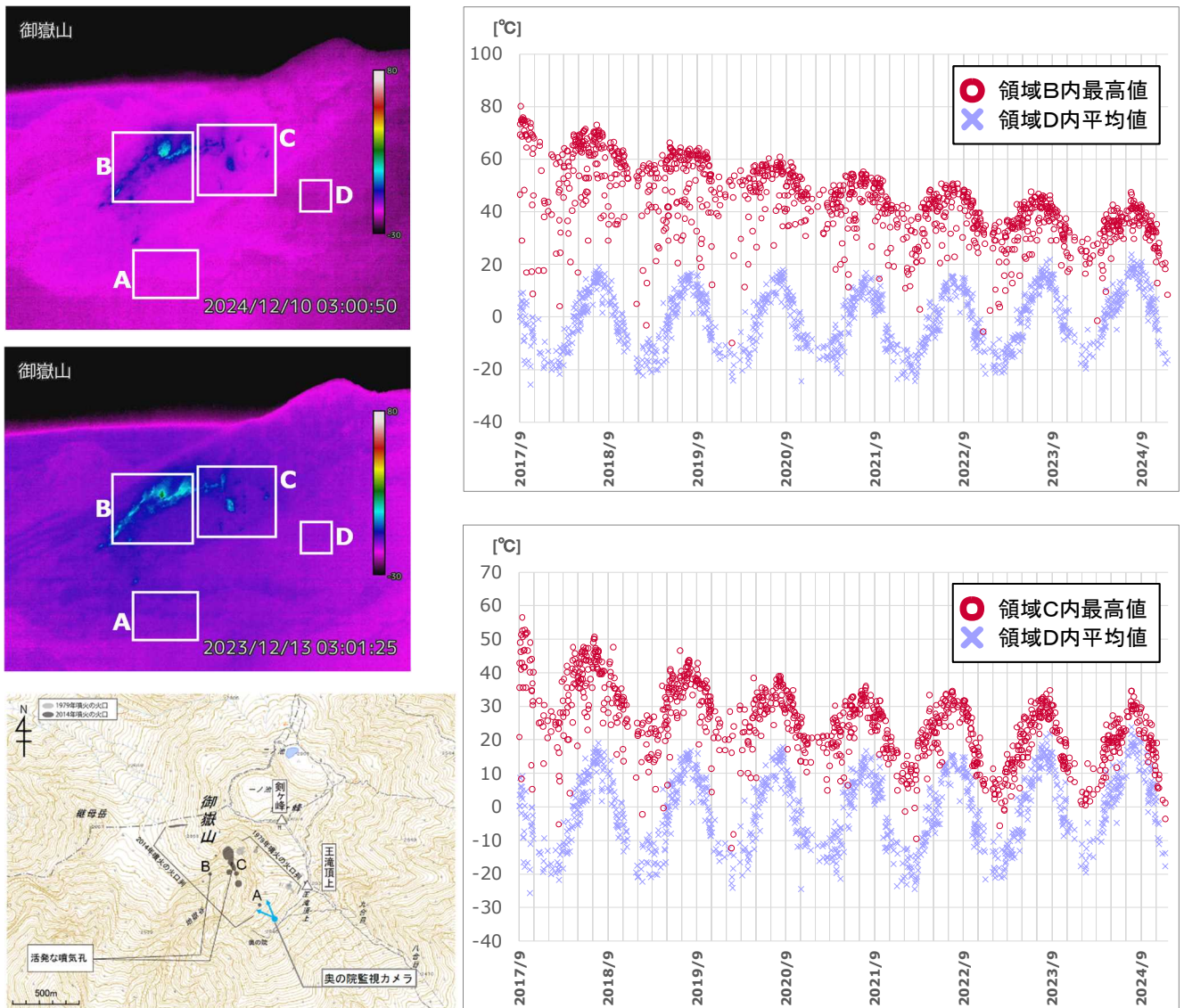
図5 御嶽山 奥の院赤外熱映像カメラによる剣ヶ峰南西側における最高温度の推移 (2017年9月13日～2024年12月31日)
