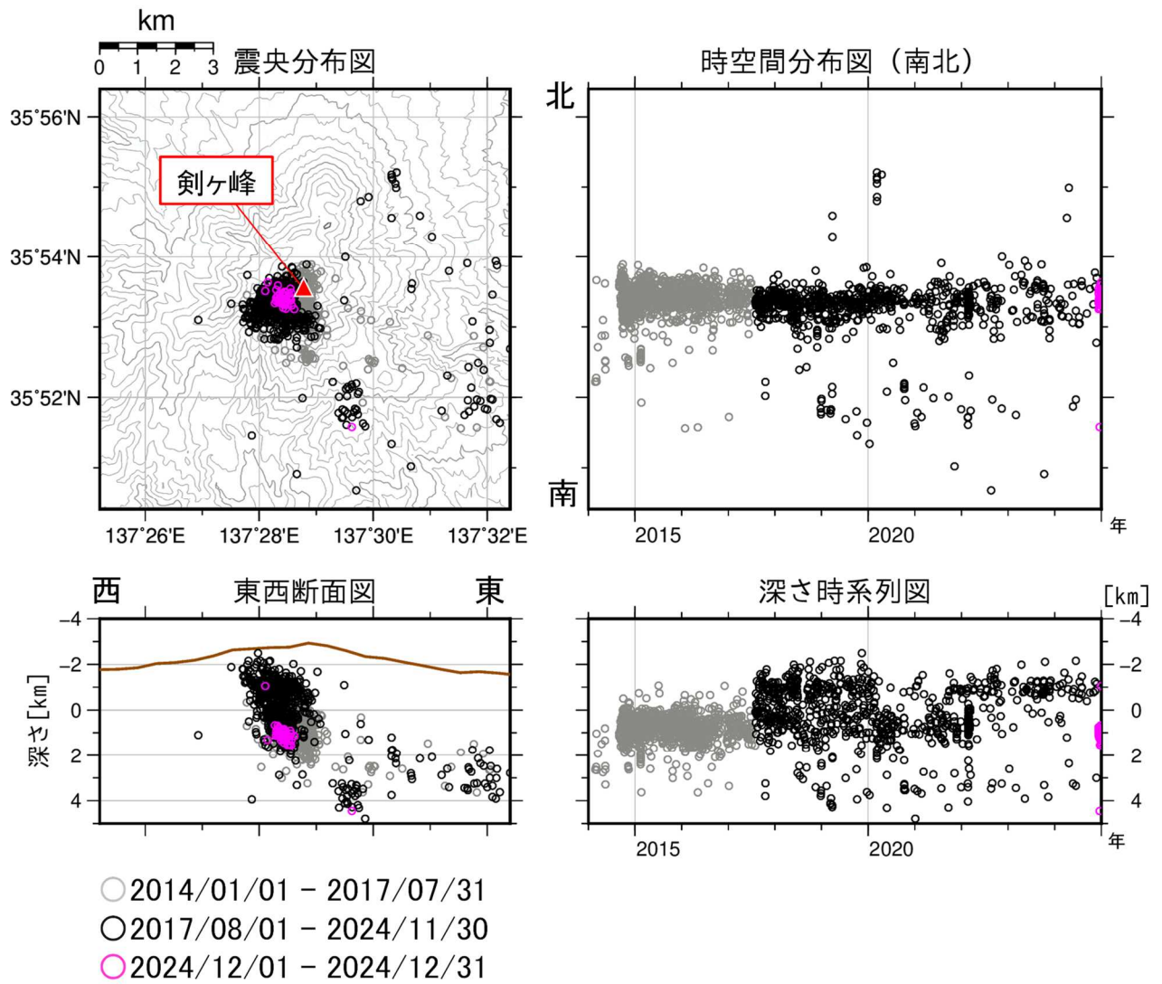
図6 御嶽山 震源分布図（2014年1月1日～2024年12月31日）
