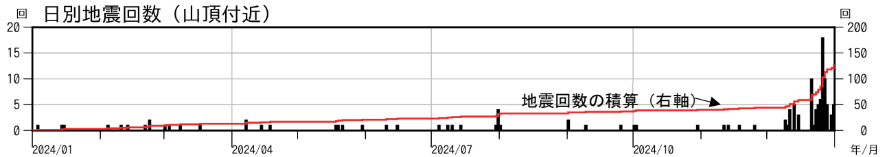
図2 御嶽山 山頂付近の直下を震源とする地震の日別回数（2024年1月1日～2024年12月31日）
