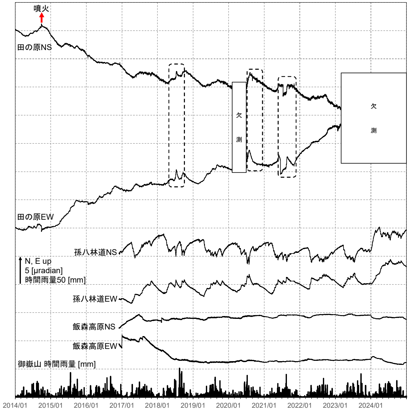
図8 御嶽山 傾斜変動（2014年1月1日～2024年12月31日）
