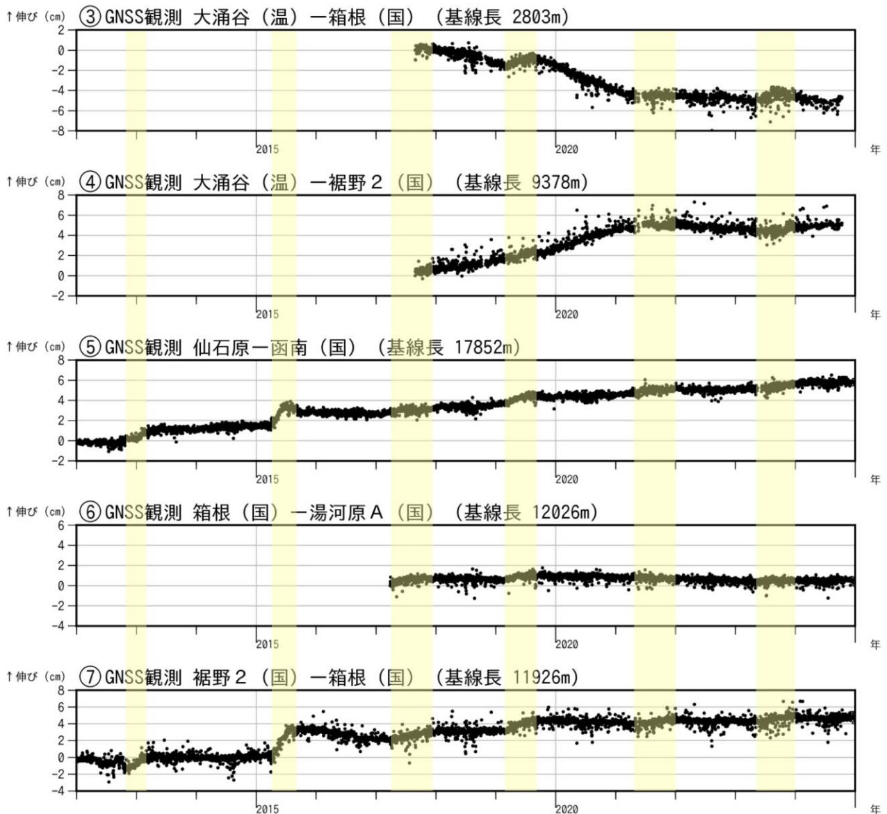
図3-2 箱根山 GNSS連続観測による 基線長変化及び観測点配置図 (2012年1月1日～2024年12月31日) (国): 国土地理院 (温): 神奈川県温泉地学研究所 空白部分は欠測を示します。 システム更新に伴う調整中のため、一部の 過去データにステップ状の変化がみ られています。
