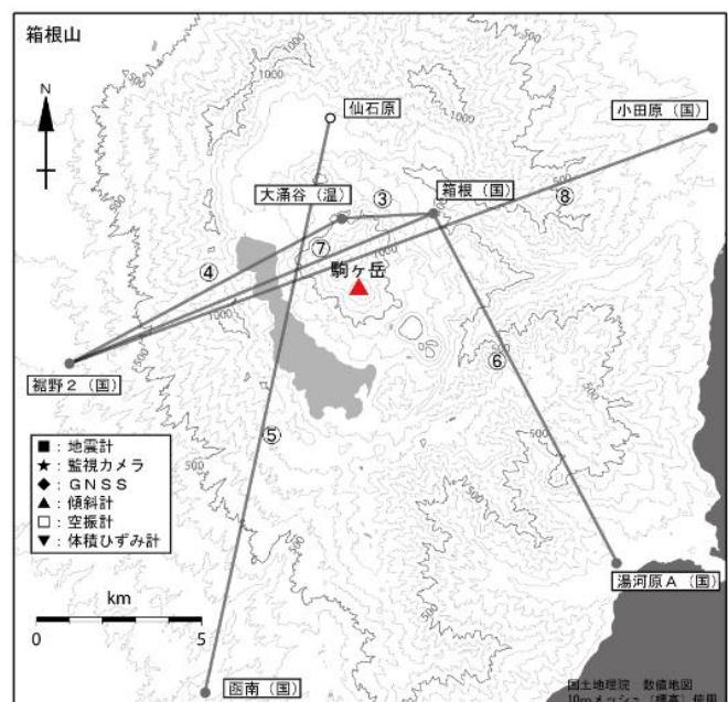
図3-2 箱根山 GNSS連続観測による 基線長変化及び観測点配置図 (2012年1月1日～2024年12月31日) (国): 国土地理院 (温): 神奈川県温泉地学研究所 空白部分は欠測を示します。 システム更新に伴う調整中のため、一部の 過去データにステップ状の変化がみ られています。
