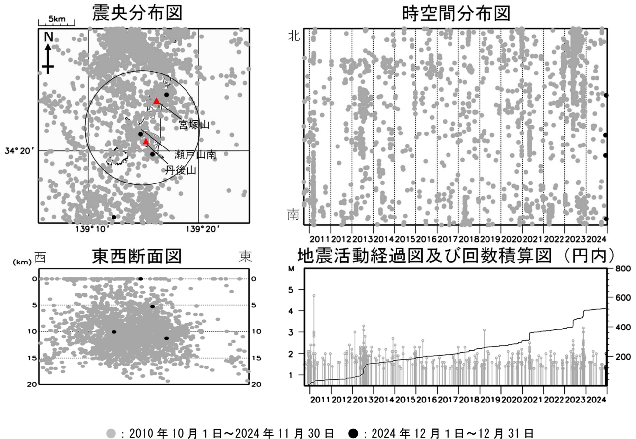
図3 新島 広域地震観測網による山体・周辺の地震活動
