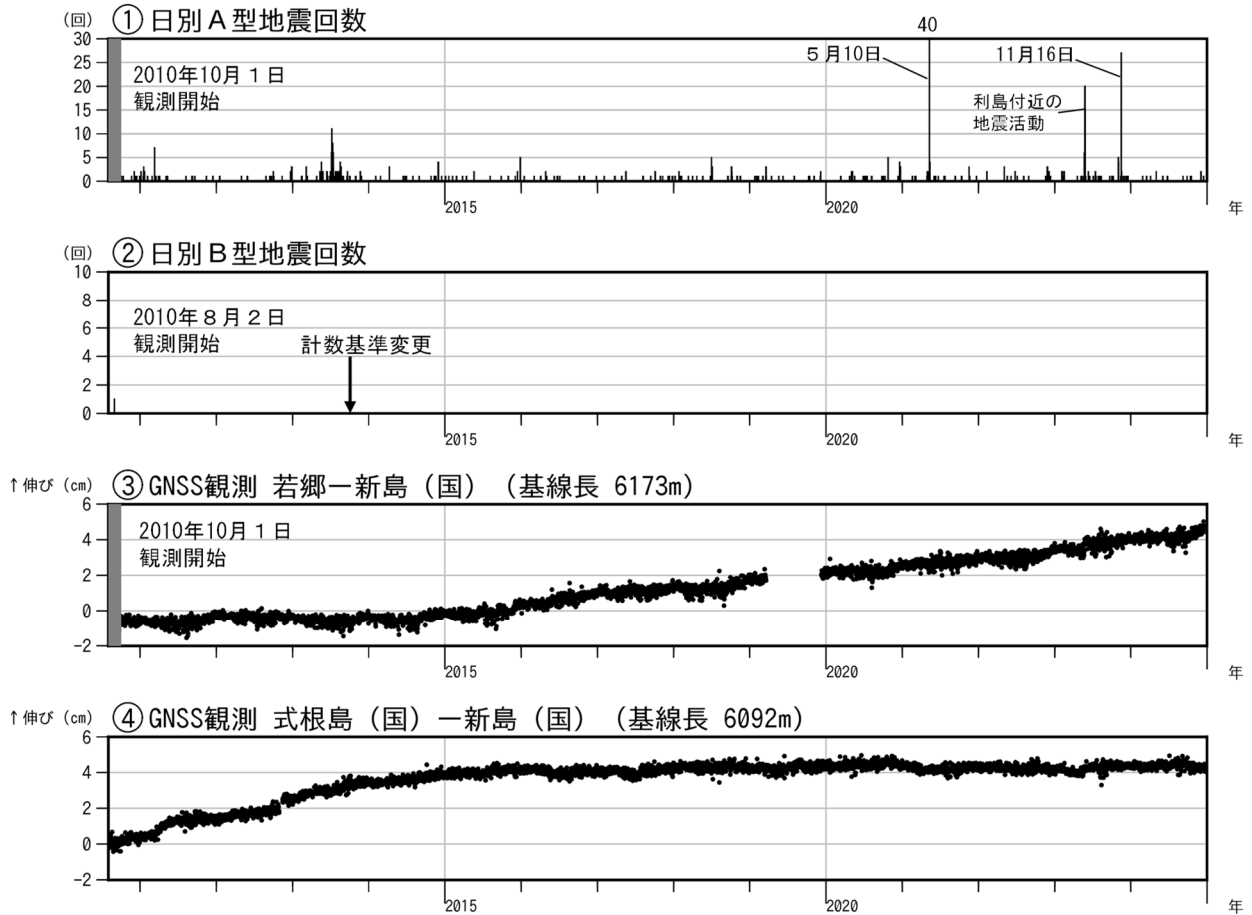
図2 新島 火山活動経過図(2010年8月2日～2024年12月31日)
