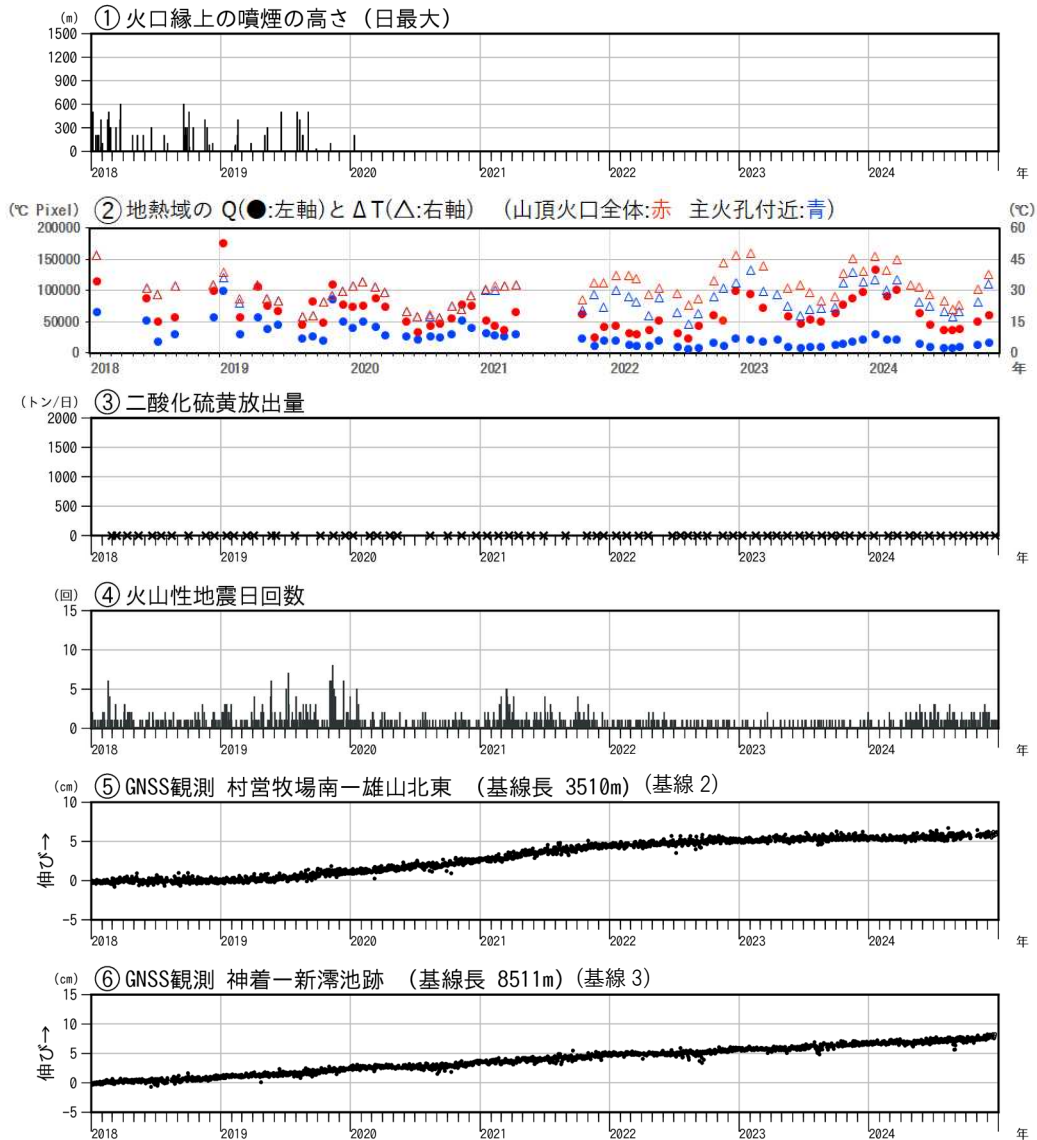
図6 三宅島 火山活動経過図（2018年1月1日～2024年12月31日）
