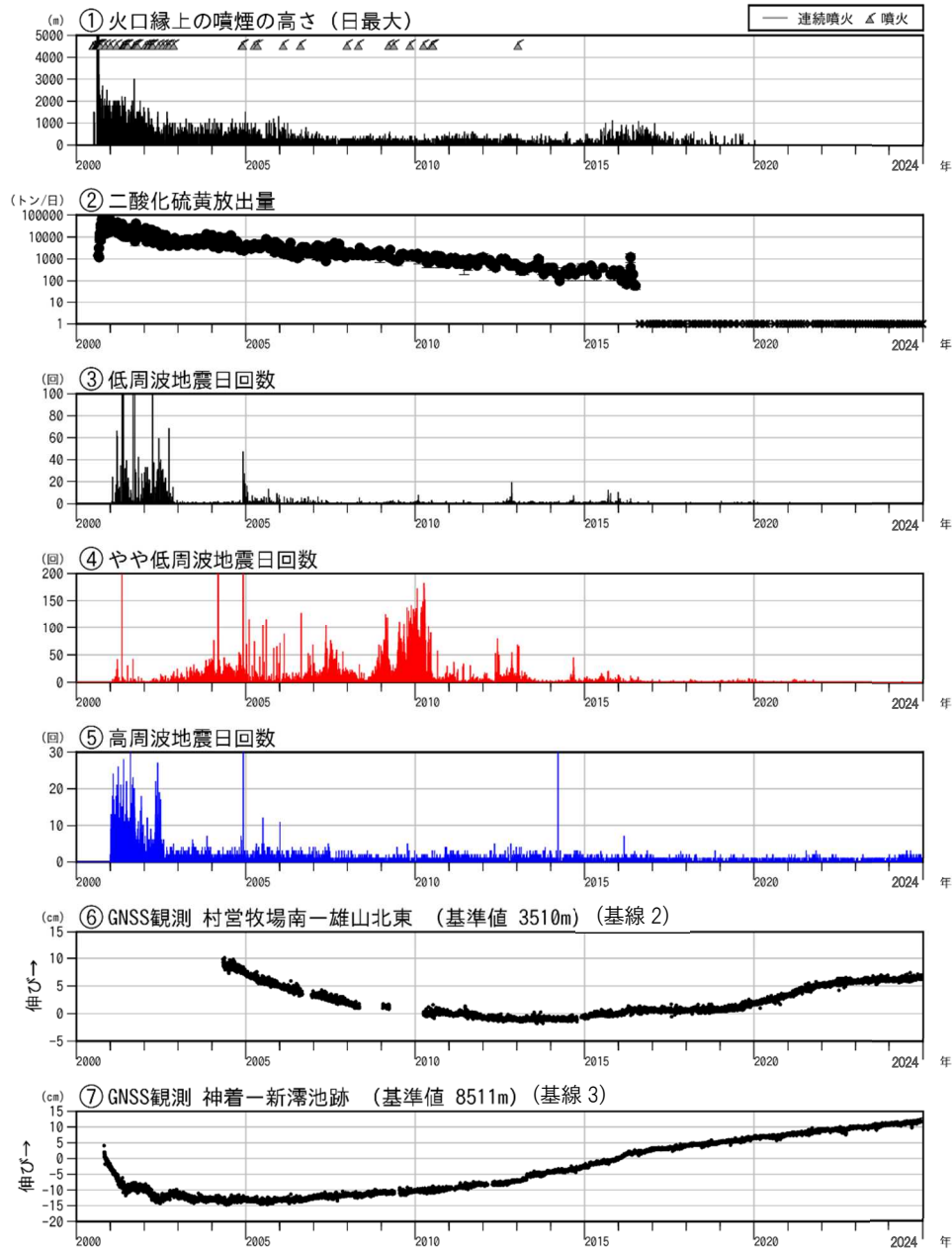
図7 三宅島 長期の火山活動経過図（2000年1月1日～2024年12月31日）
