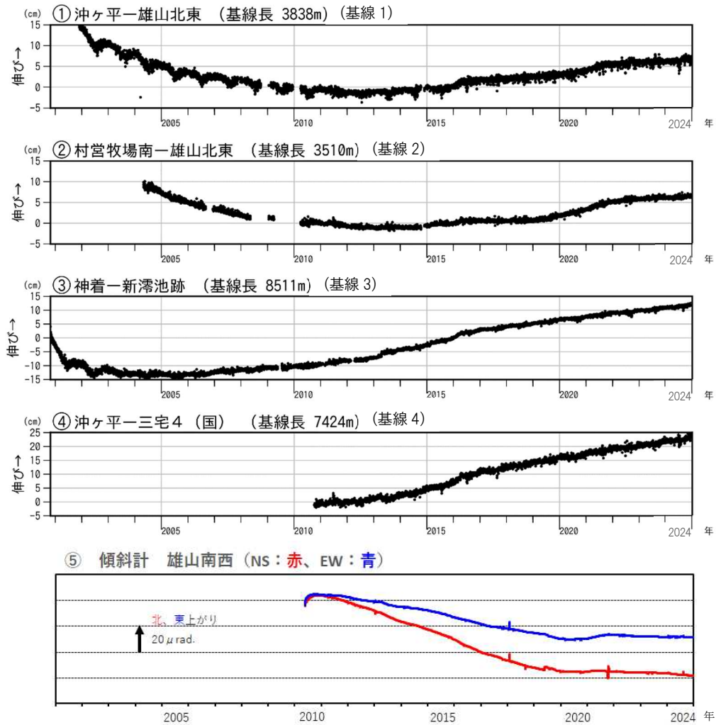
図8 三宅島 GNSS 連続観測及び傾斜計観測結果（2000 年 10 月 26 日～2024 年 12 月 31 日）
