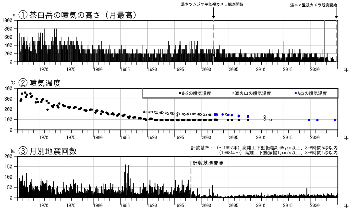
図3-1 那須岳 火山活動経過図（1966年6月～2025年1月）
