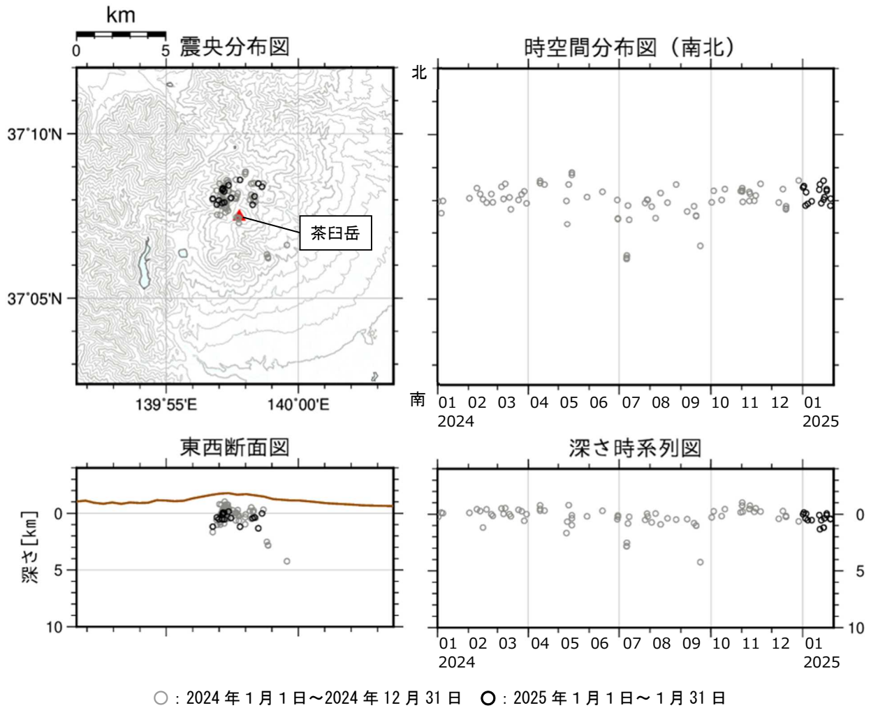
図5 那須岳 震源分布図（2024 年 1 月 1 日～2025 年 1 月 31 日）
