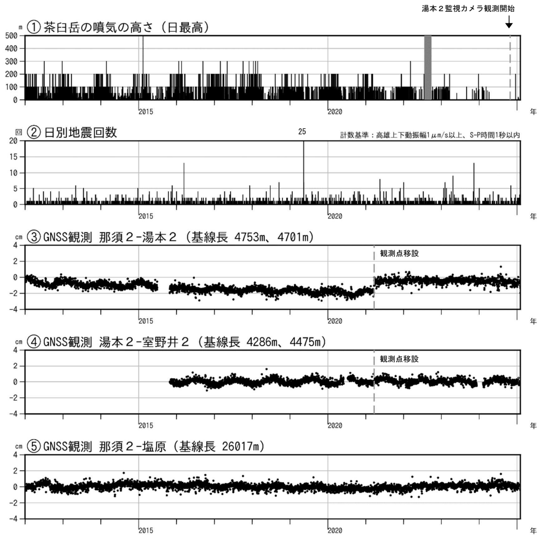
図4 那須岳 火山活動経過図（2012年1月1日～2025年1月31日）
