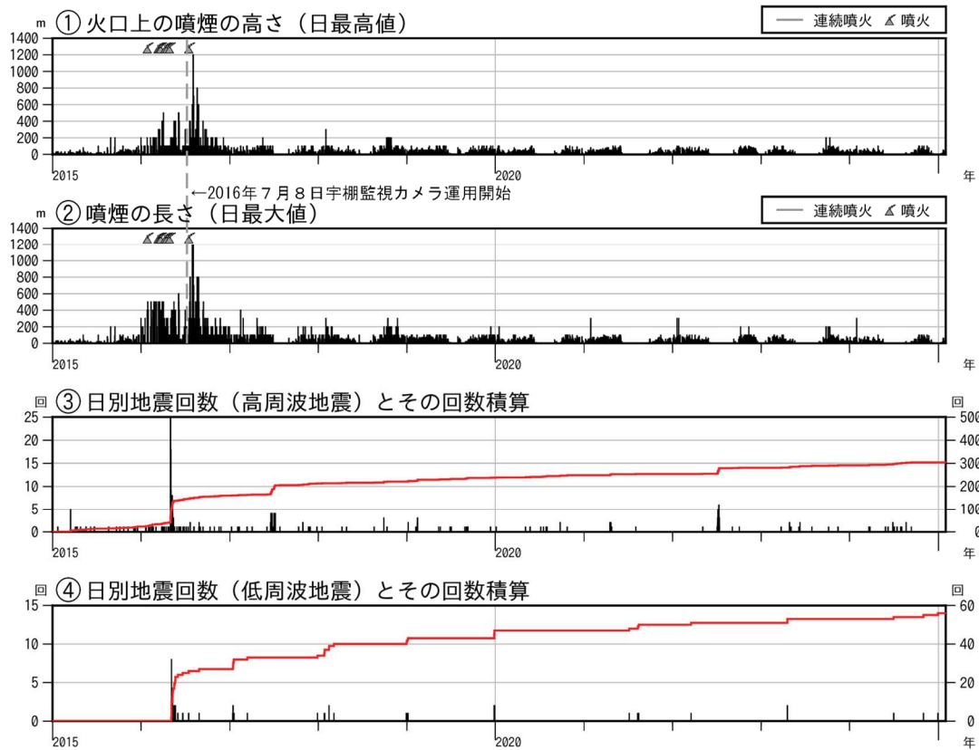
図 3 新潟焼山 火山活動経過図（短期）（2015 年 1 月 1 日～2025 年 1 月 31 日）
