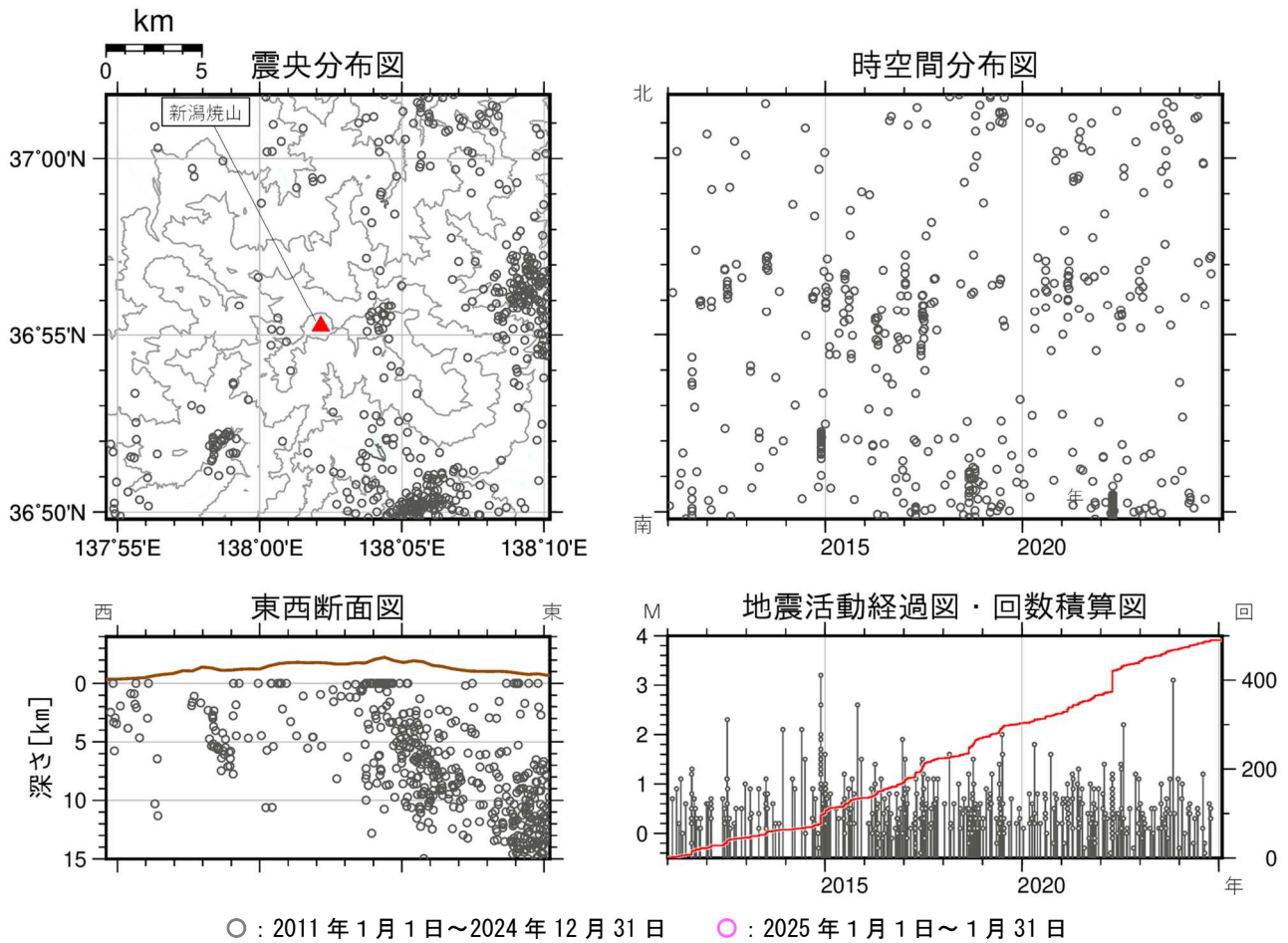
図4 新潟焼山 広域地震観測網による山体・周辺の地震活動（2011 年 1 月 1 日～2025 年 1 月 31 日）
