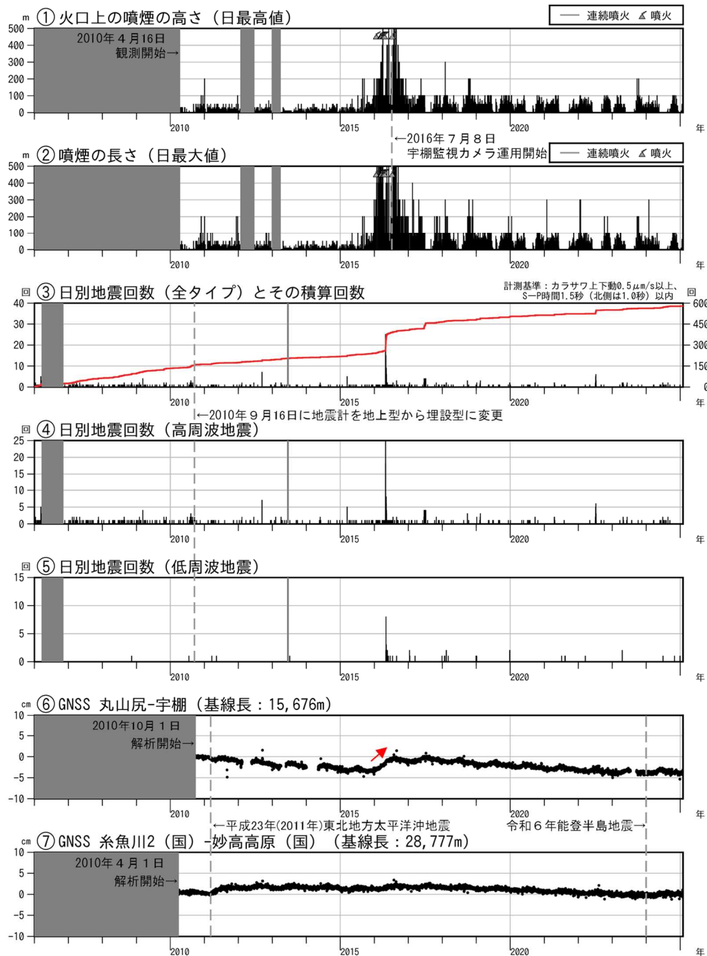
図2 新潟焼山 火山活動経過図（2006年1月1日～2025年1月31日）
