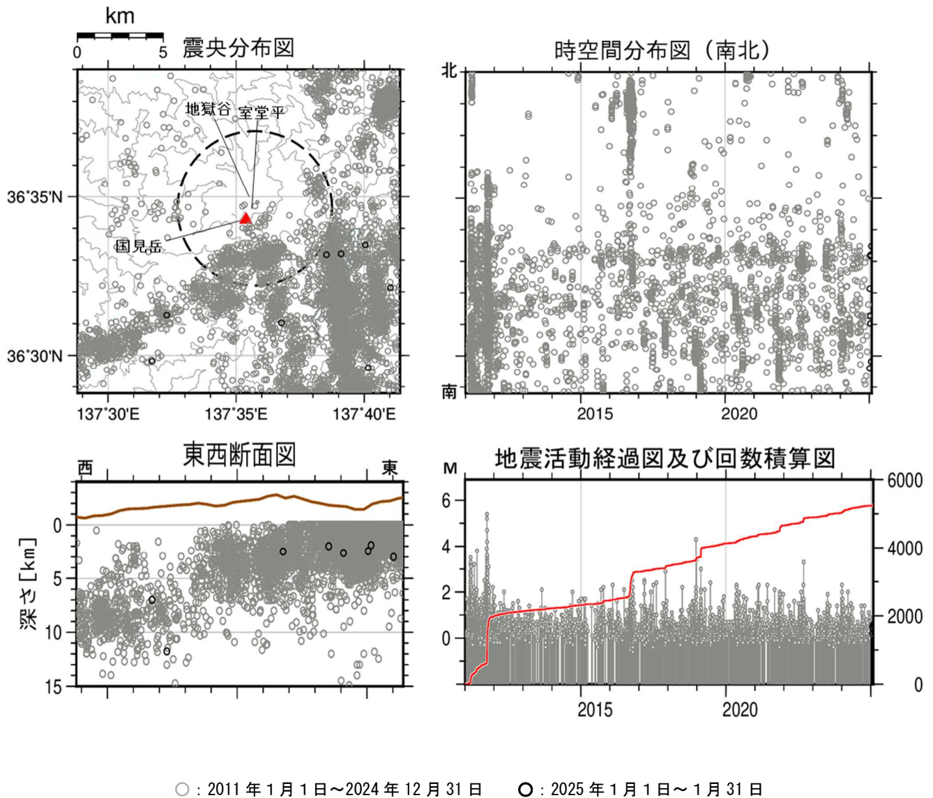
図2 弥陀ヶ原 広域地震観測網による山体・周辺の地震活動（2011 年 1 月 1 日～2025 年 1 月 31 日） 震央分布図中の円は弥陀ヶ原の計数対象地震（室堂平で S-P 時間 1 秒以内）のおよその範囲を示しています。 広域地震観測網により震源決定したもので、深さは全て海面以下として決定しています。なお、2020 年 9 月以降については、地震観測点の標高を考慮する等、震源決定の手法を変更しております。 図中の震源要素は一部暫定値が含まれており、後日変更することがあります。
