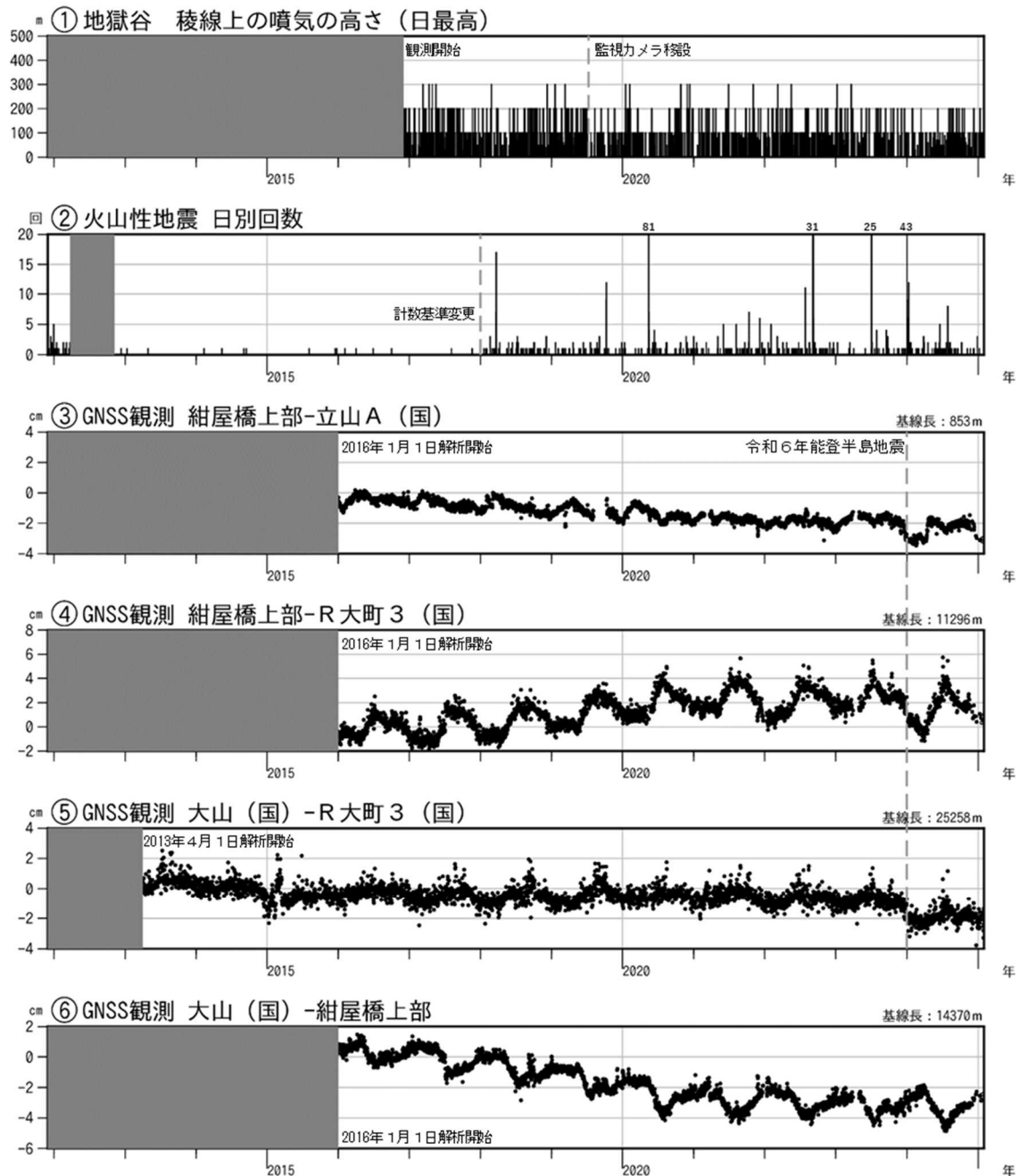
図3 弥陀ヶ原 火山活動経過図（2011年12月1日～2025年1月31日）
