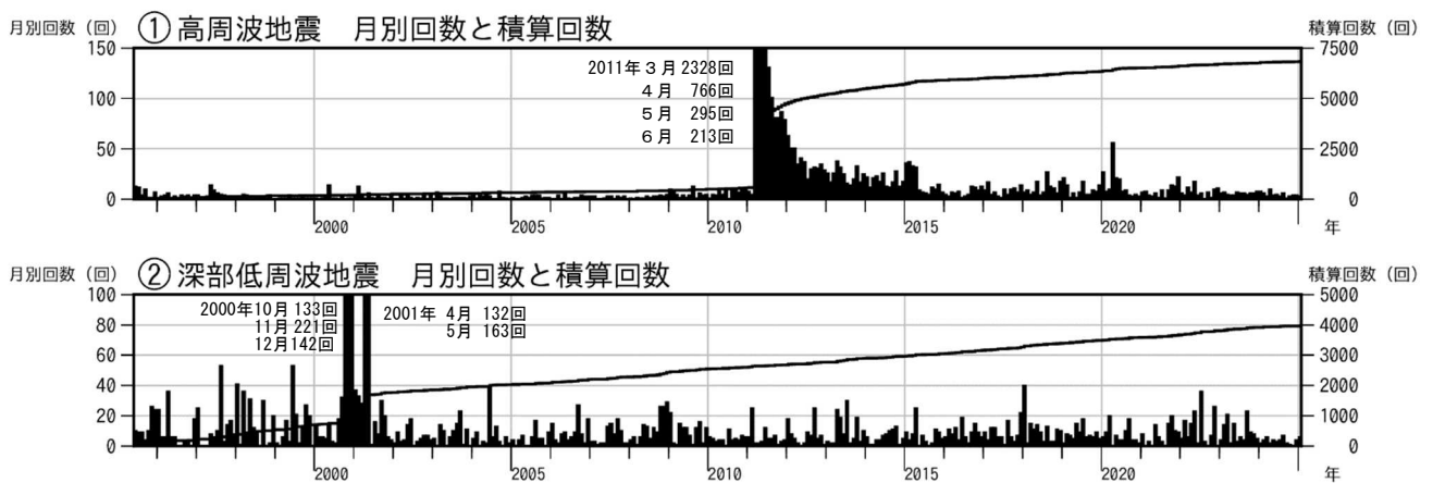
図2 富士山 月別地震回数（1995年6月1日～2025年1月31日）
