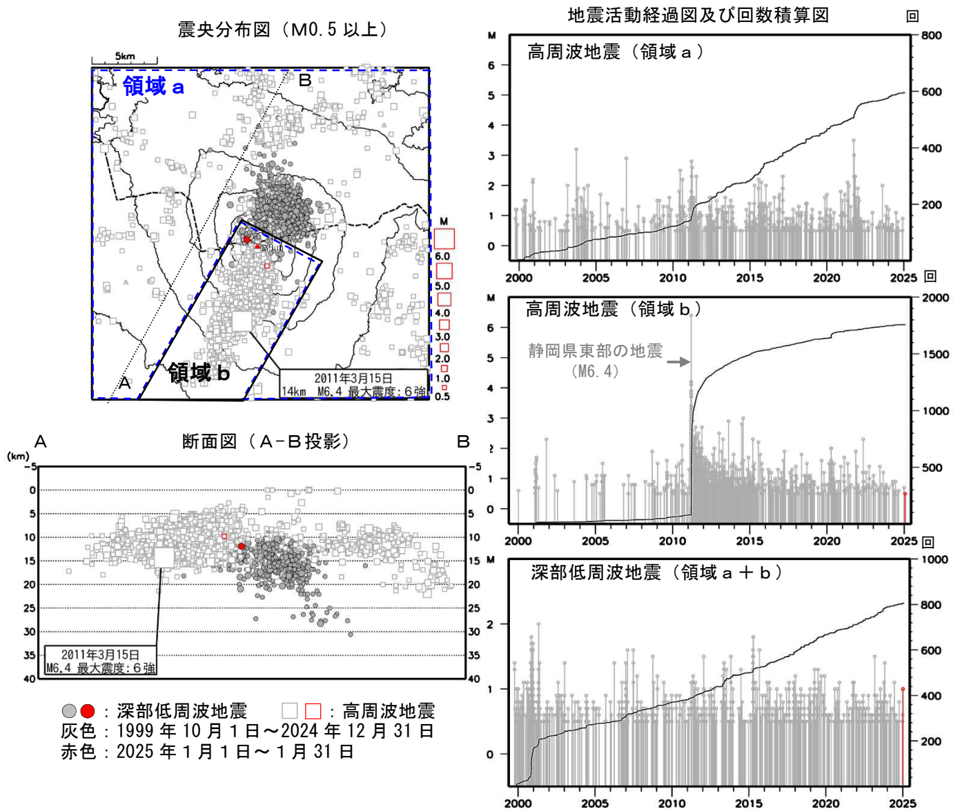
図3 富士山 広域地震観測網による山体及び周辺の地震活動（1999年10月1日～2025年1月31日）
