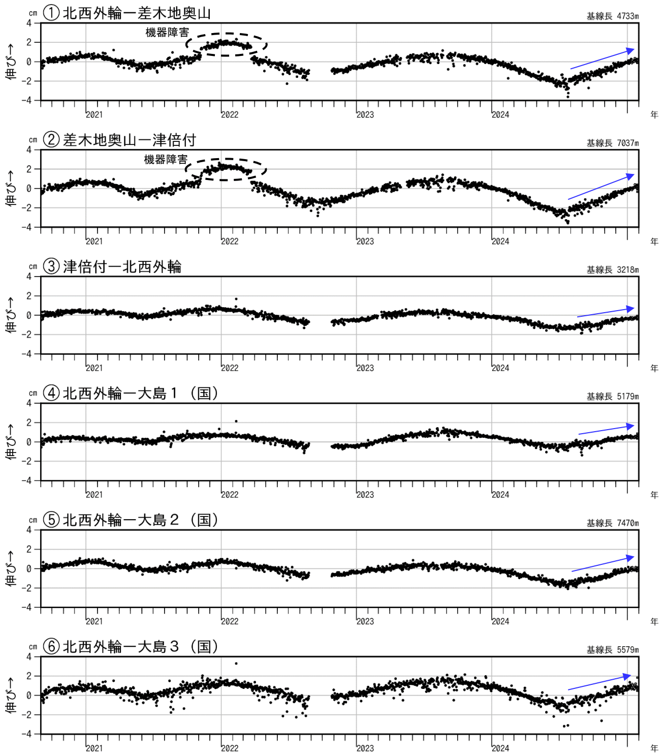
図 3-2 伊豆大島 GNSS 連続観測による基線長変化(2020 年 9 月～2025 年 1 月 31 日)
