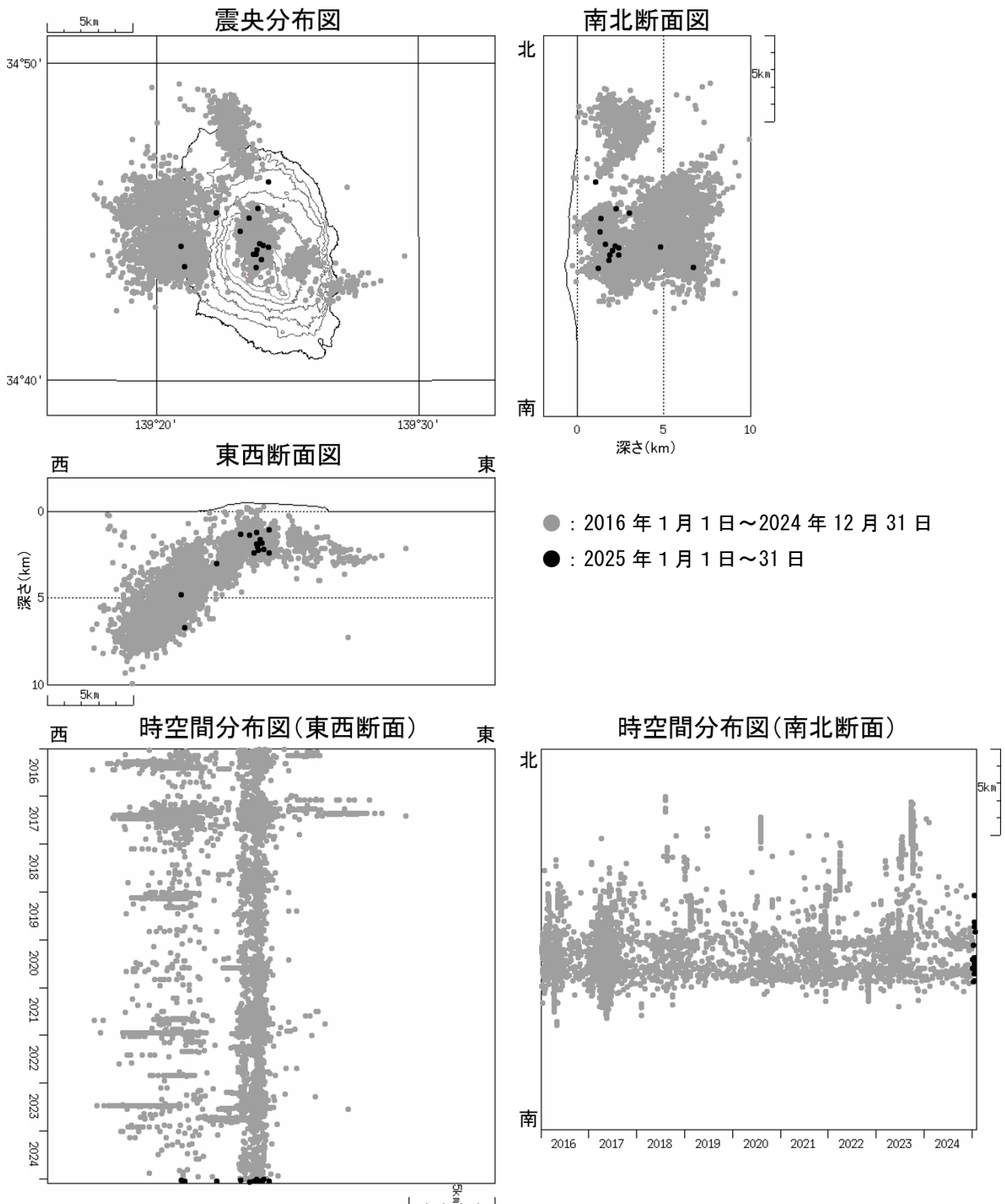
図4 伊豆大島 震源分布図（2016 年 1 月 1 日～2025 年 1 月 31 日）
