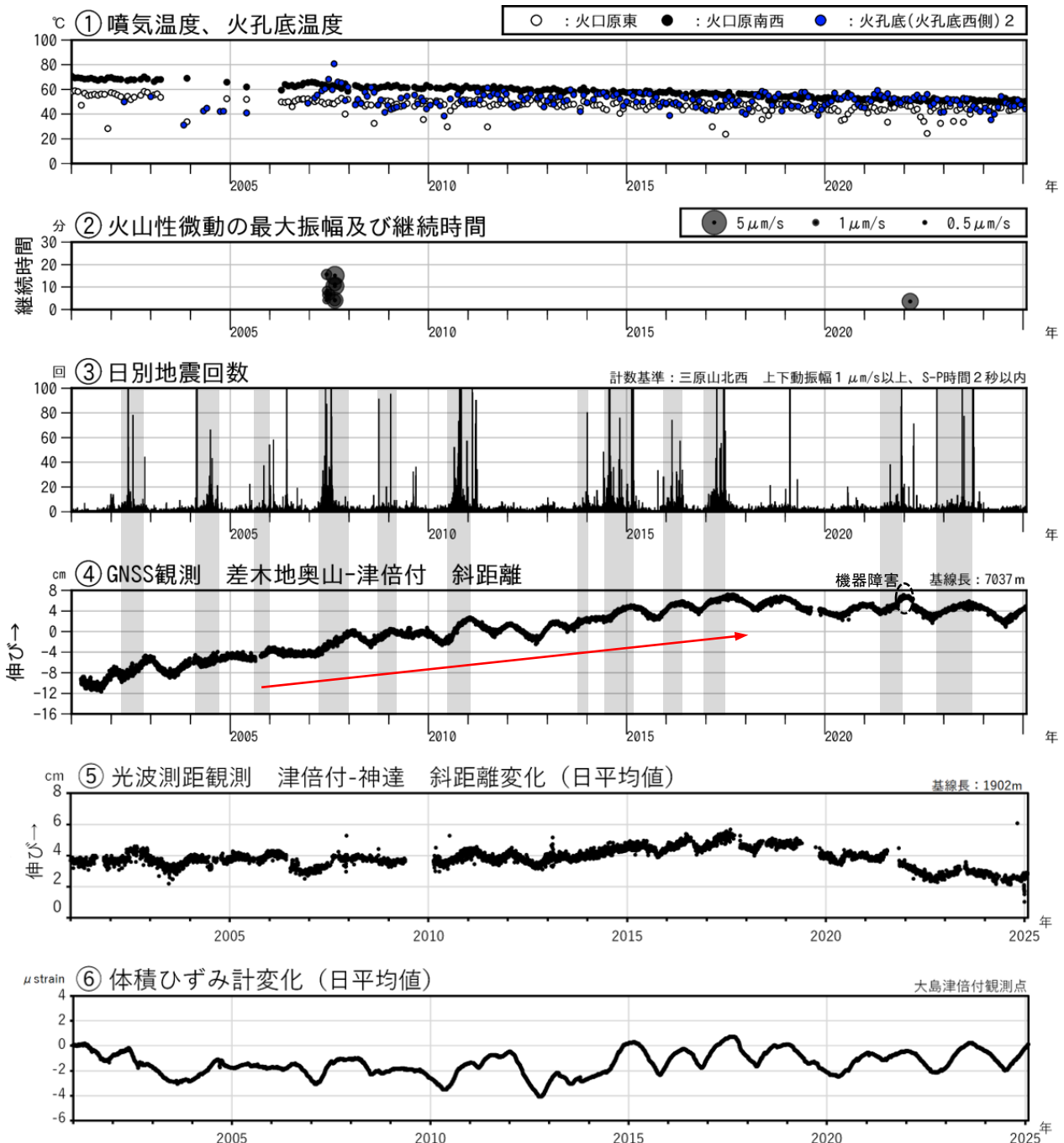
図2 伊豆大島 最近の火山活動経過図（2001年1月～2025年1月31日）
