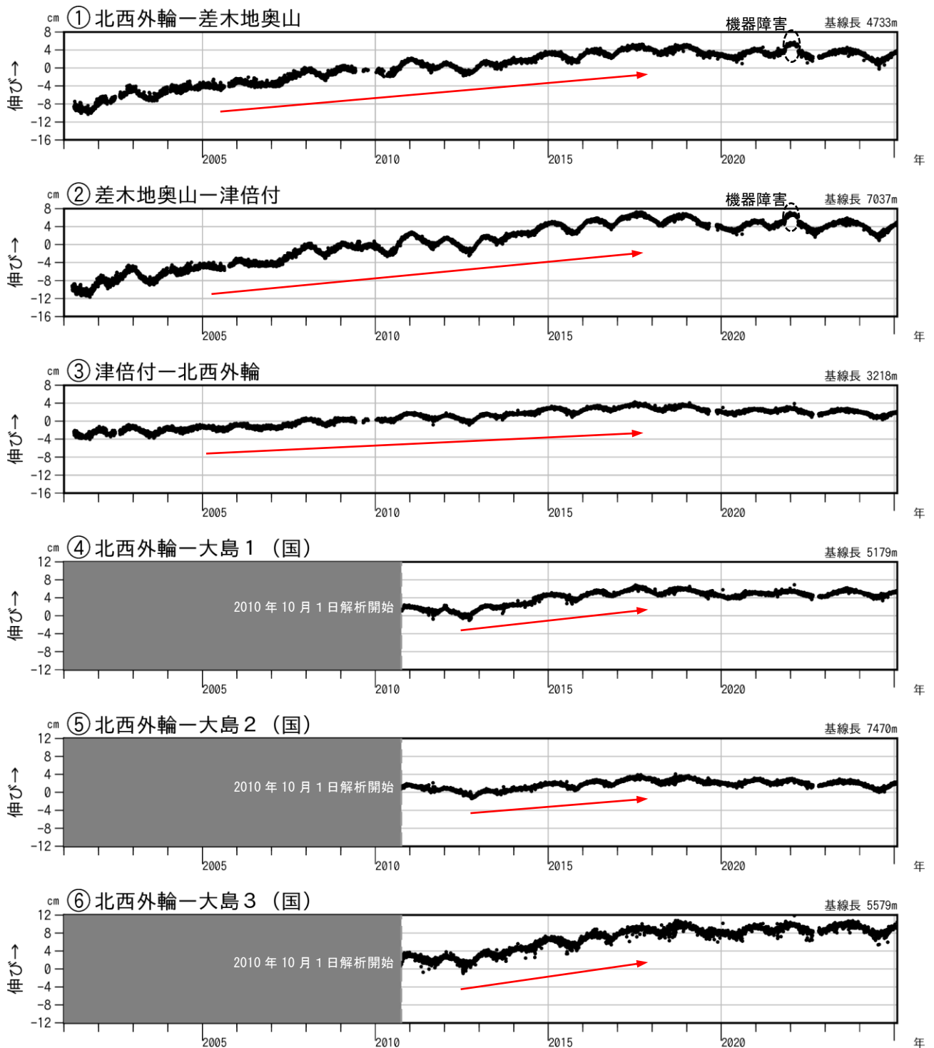
図 3-1 伊豆大島 GNSS 連続観測による基線長変化(2001 年 1 月～2025 年 1 月 31 日)
