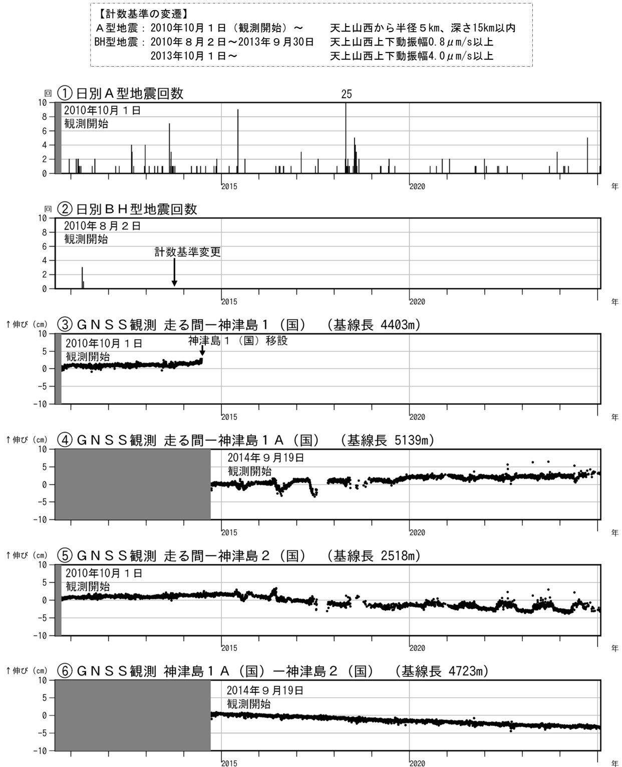
図2 神津島 火山活動経過図(2010年8月2日～2025年1月31日)
