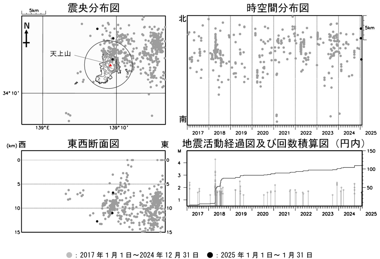
図3 神津島 広域地震観測網による山体・周辺の地震活動（2017年1月1日～2025年1月31日）
