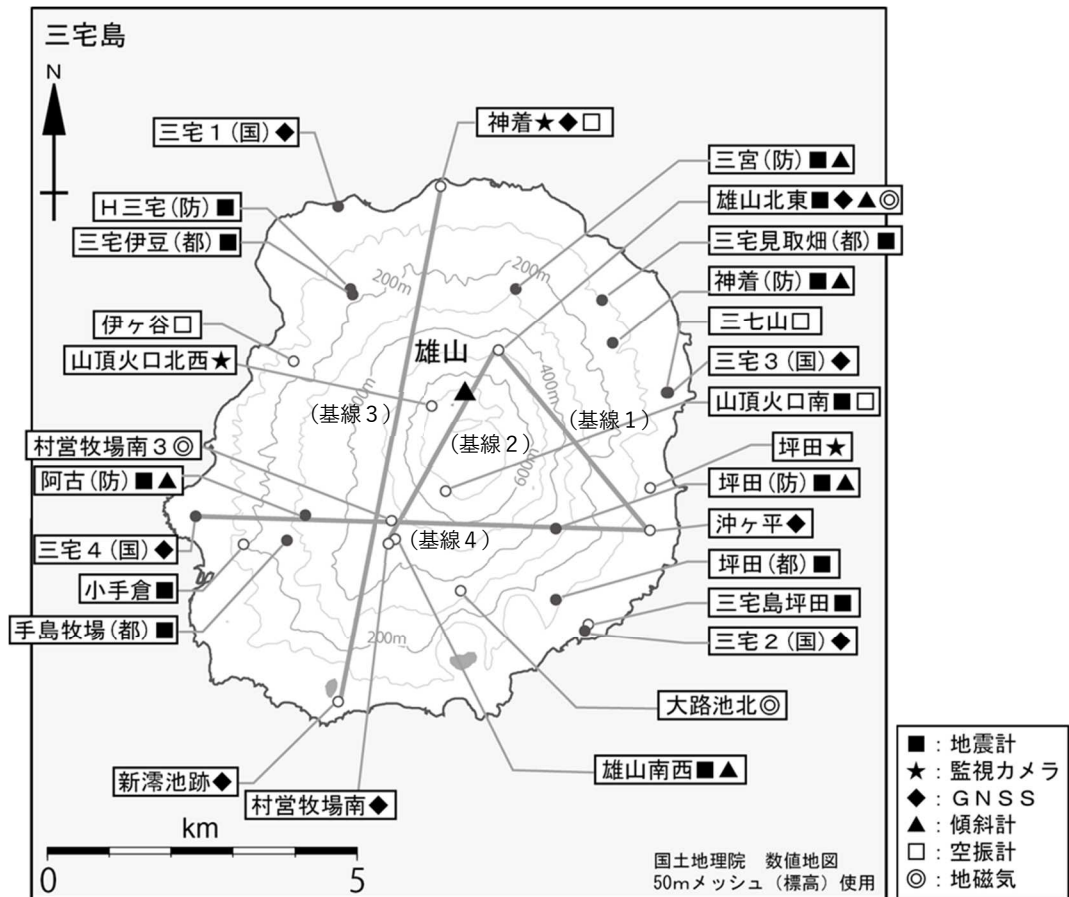
図 11 三宅島 観測点配置図
