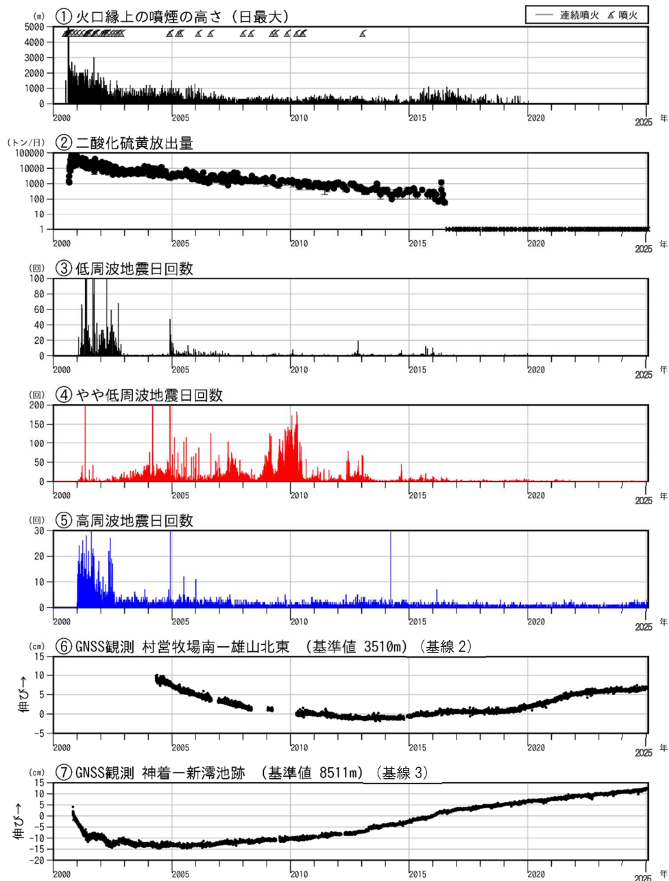
図7 三宅島 長期の火山活動経過図（2000年1月1日～2025年1月31日）
