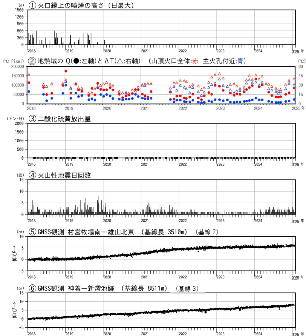
図6 三宅島 火山活動経過図（2018年1月1日～2025年1月31日）
