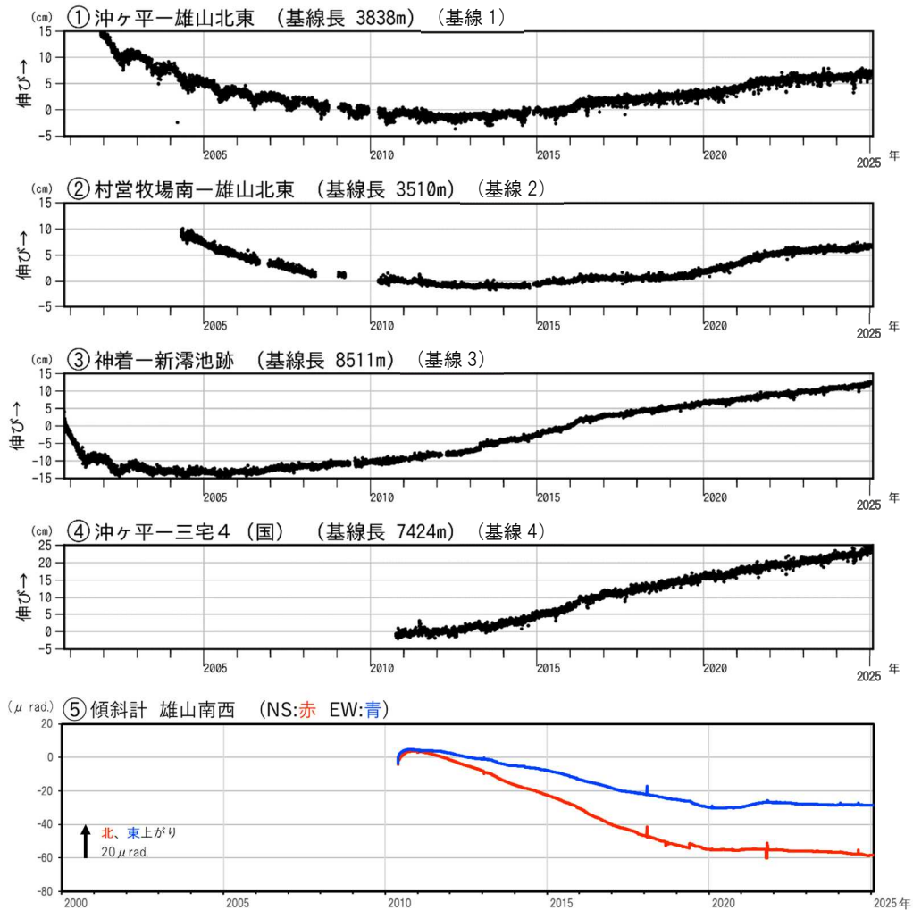
図8 三宅島 GNSS 連続観測及び傾斜計観測結果（2000年10月26日～2025年1月31日）
