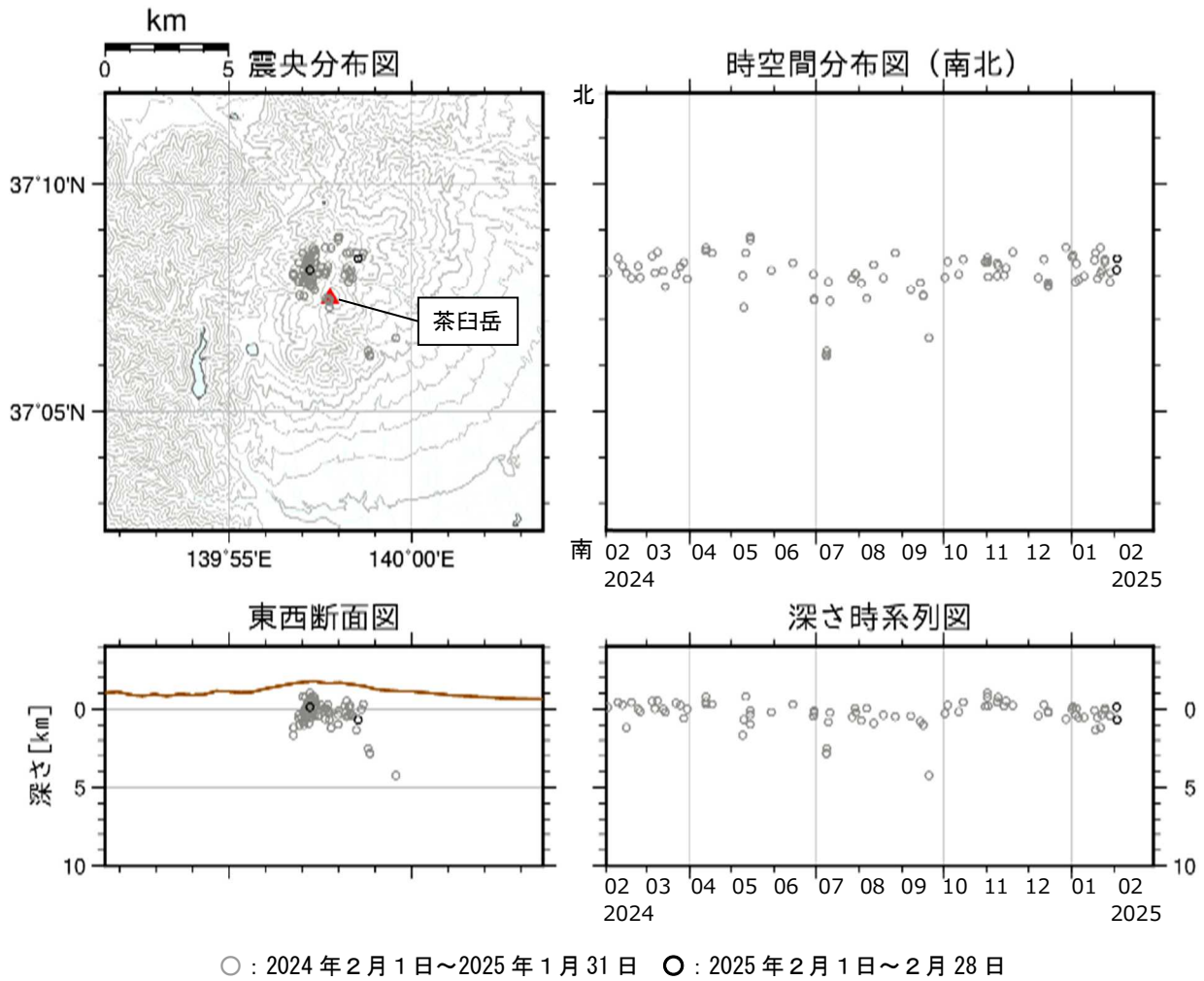
図5 那須岳 震源分布図（2024 年 2 月 1 日～2025 年 2 月 28 日）
