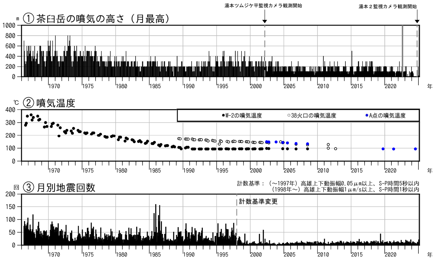
図3-1 那須岳 火山活動経過図（1966年6月～2025年2月）
