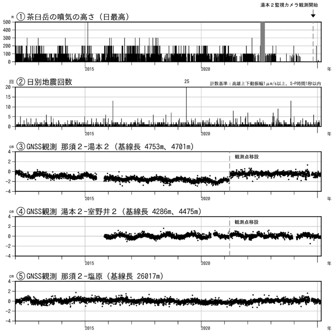
図4 那須岳 火山活動経過図（2012年1月1日～2025年2月28日）
