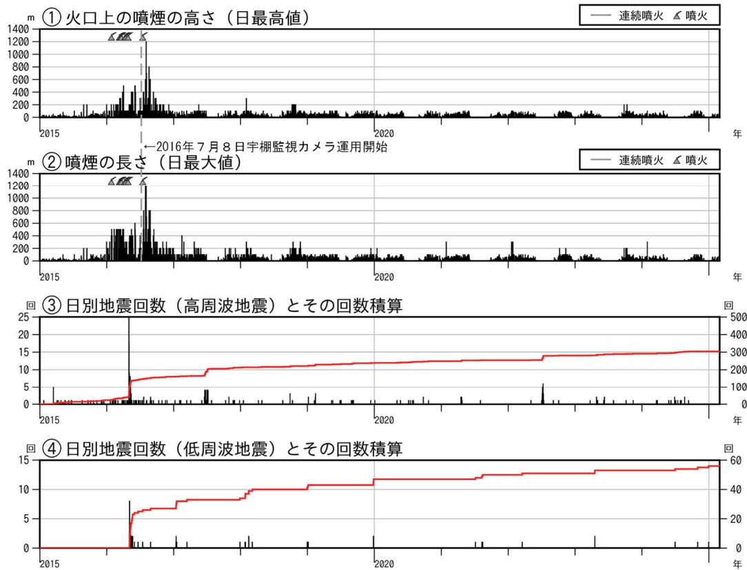
図 3 新潟焼山 火山活動経過図（短期）（2015 年 1 月 1 日～2025 年 2 月 28 日）
