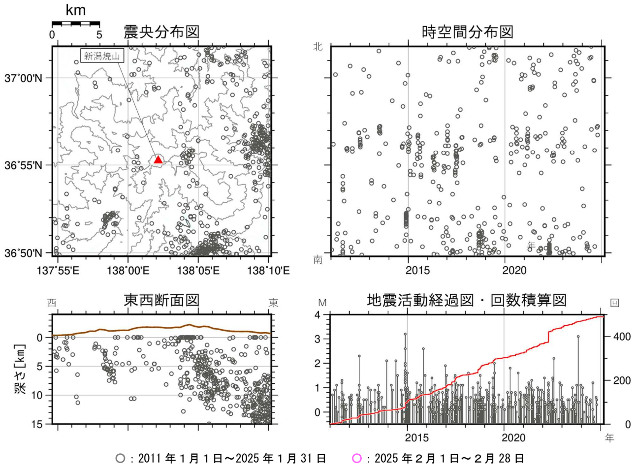
図 4 新潟焼山 広域地震観測網による山体・周辺の地震活動（2011 年 1 月 1 日～2025 年 2 月 28 日）
