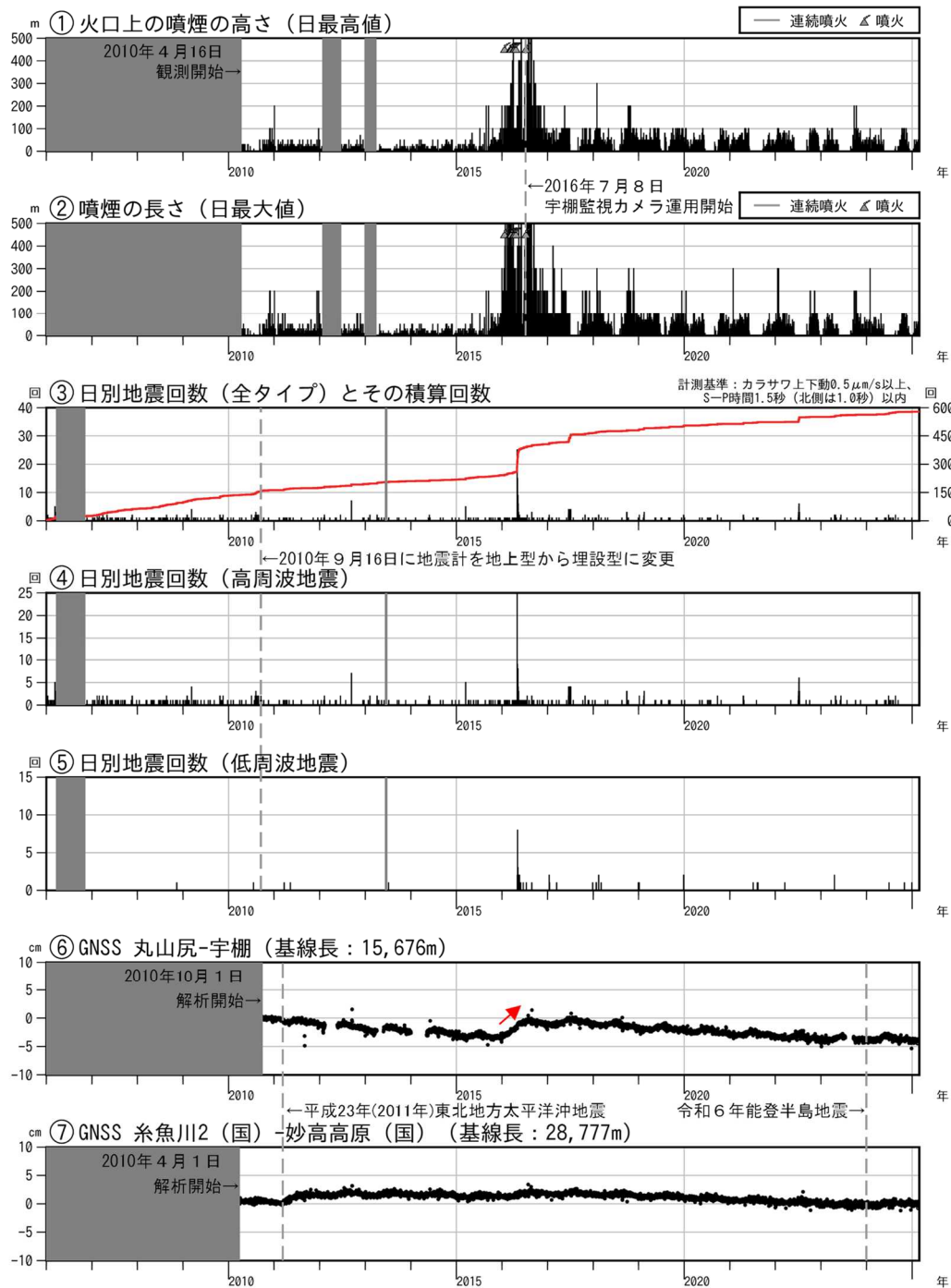
図2 新潟焼山 火山活動経過図（2006年1月1日～2025年2月28日）
