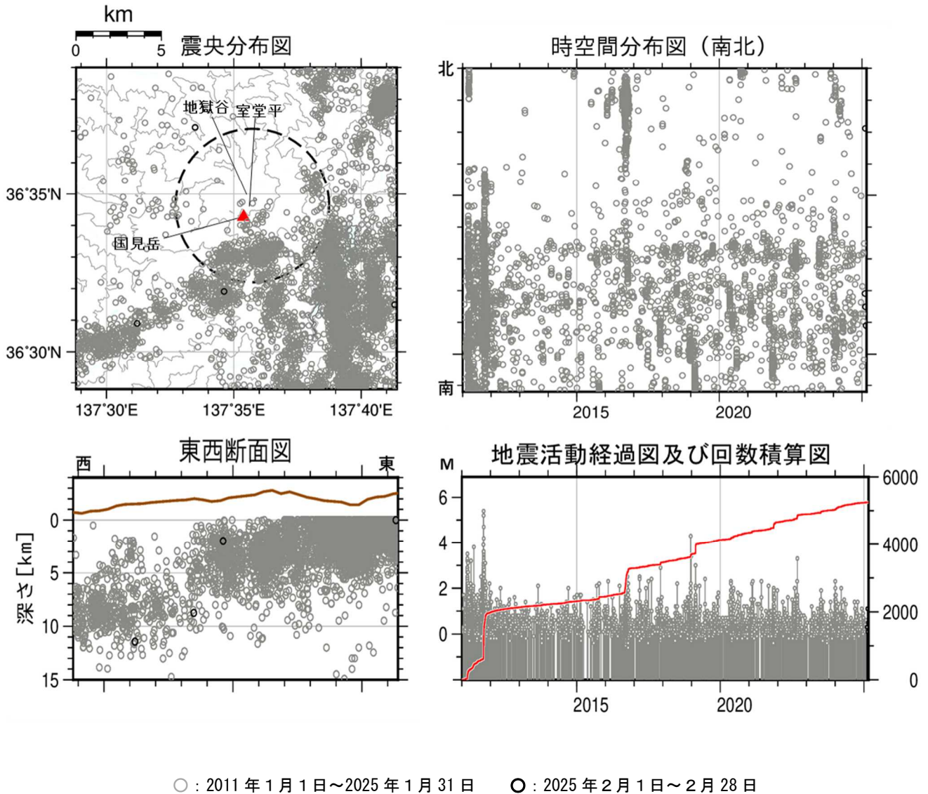
図2 弥陀ヶ原 広域地震観測網による山体・周辺の地震活動（2011 年 1 月 1 日～2025 年 2 月 28 日） 震央分布図中の円は弥陀ヶ原の計数対象地震（室堂平で S-P 時間 1 秒以内）のおよその範囲を示しています。 広域地震観測網により震源決定したもので、深さは全て海面以下として決定しています。なお、2020 年 9 月以降については、地震観測点の標高を考慮する等、震源決定の手法を変更しております。 図中の震源要素は一部暫定値が含まれており、後日変更することがあります。
