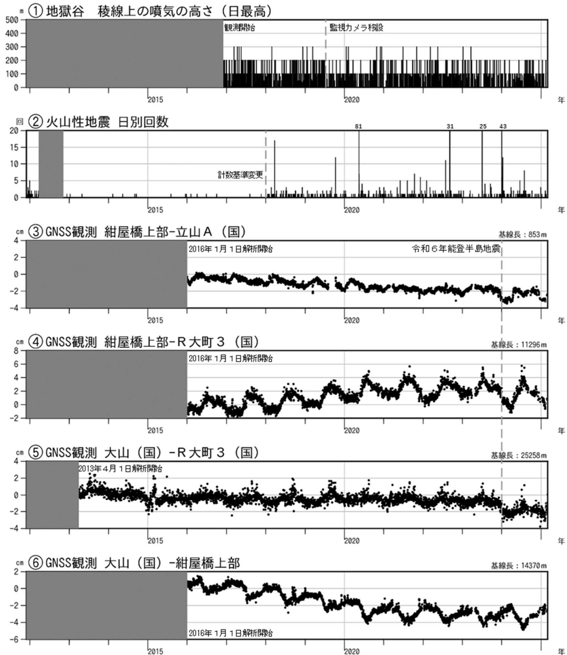
図3 弥陀ヶ原 火山活動経過図（2011年12月1日～2025年2月28日）
