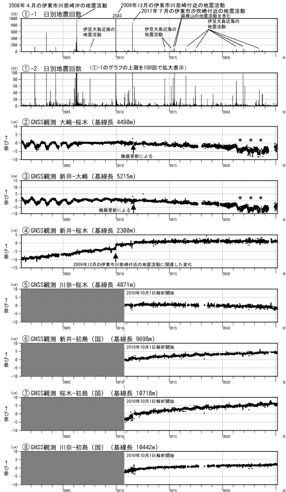
図3 伊豆東部火山群 火山活動経過図 (2001年2月1日~2025年2月28日)
