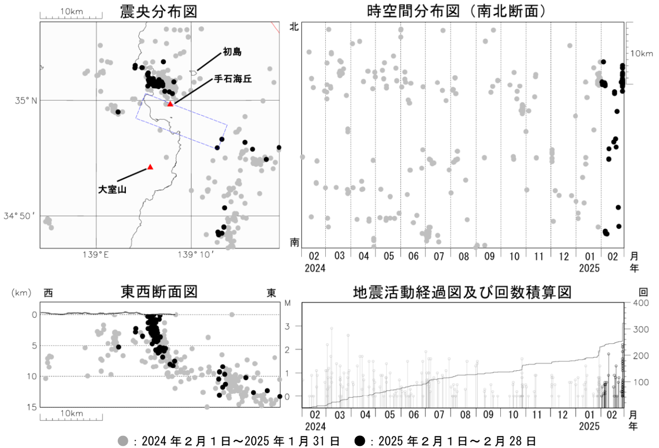
図2 伊豆東部火山群 広域地震観測網による震源分布図（2024 年 2 月 1 日～2025 年 2 月 28 日） □ の領域は群発地震活動の発生する可能性がある範囲（火口が出現する可能性のある範囲）を示しています。 https://www.data.jma.go.jp/vois/data/filing/level/PDF/level_316.pdf 広域地震観測網により震源決定したもので、深さは全て海面以下として決定しています。 M（マグニチュード）は地震の規模を表し、M0.0 以上を表示しています。 図中の震源要素は一部暫定値が含まれており、後日変更することがあります。 この図では、関係機関の地震波形を一元的に処理し、地震観測点の標高を考慮する等した手法で得られた震源を用いています。
