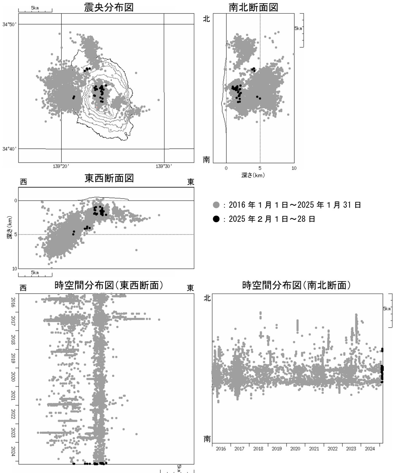
図4 伊豆大島 震源分布図（2016 年 1 月 1 日～2025 年 2 月 28 日）
