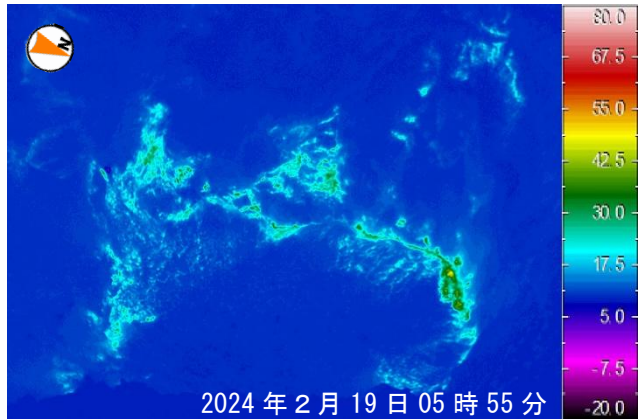
中央火孔東カメラ位置からの熱画像 （2024年2月19日 現地調査時に撮影）
