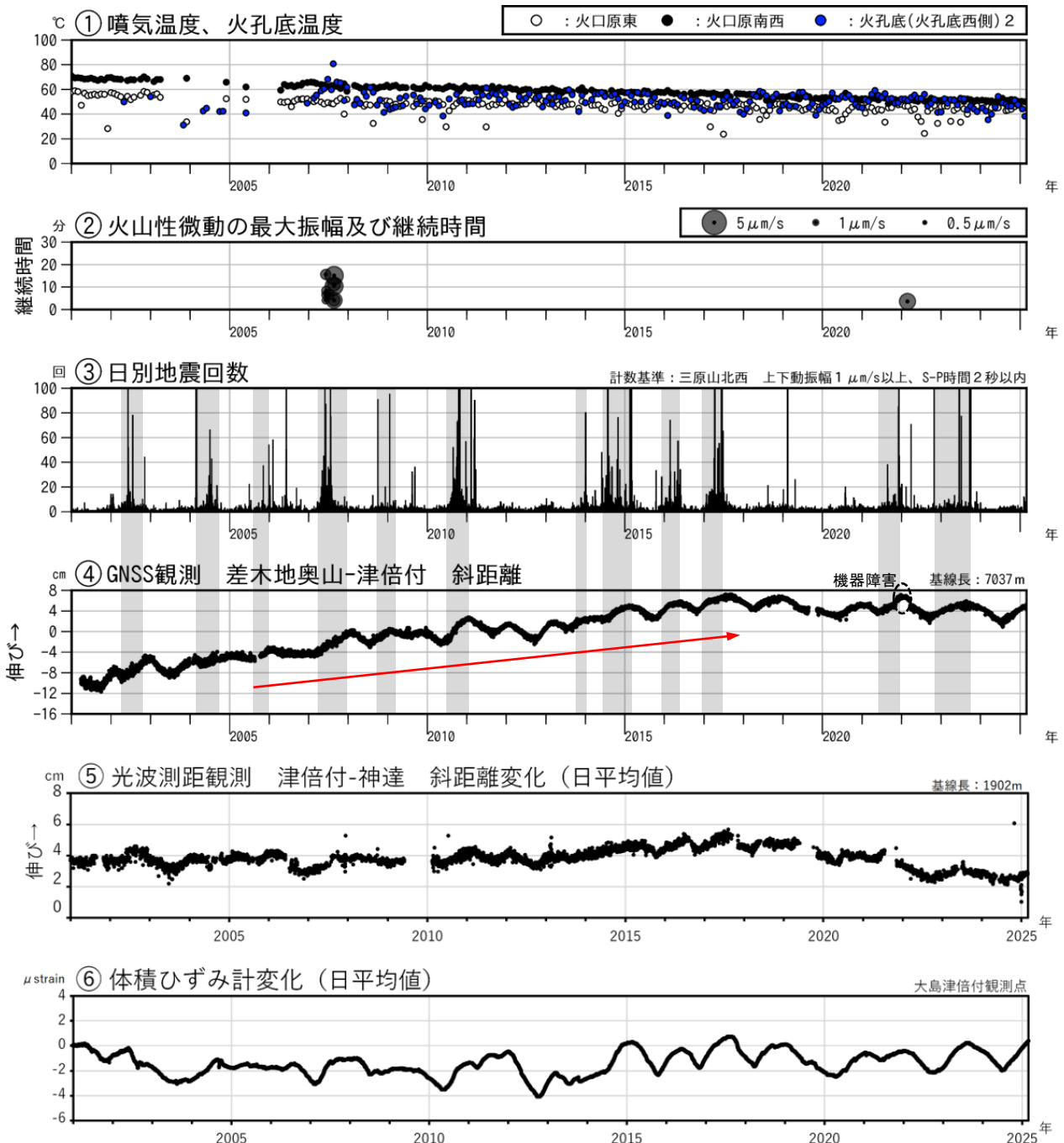
図2 伊豆大島 最近の火山活動経過図 (2001年1月～2025年2月28日)
