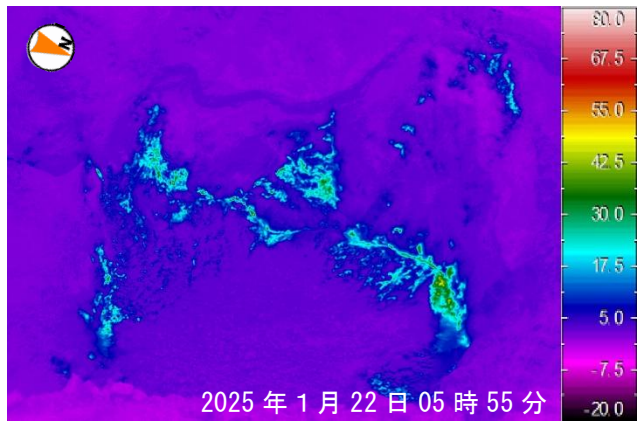
中央火孔東カメラ位置からの熱画像 （1月22日 現地調査時に撮影）
