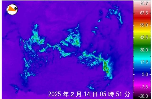
中央火孔東カメラ位置からの熱画像 （2月14日 現地調査時に撮影）
