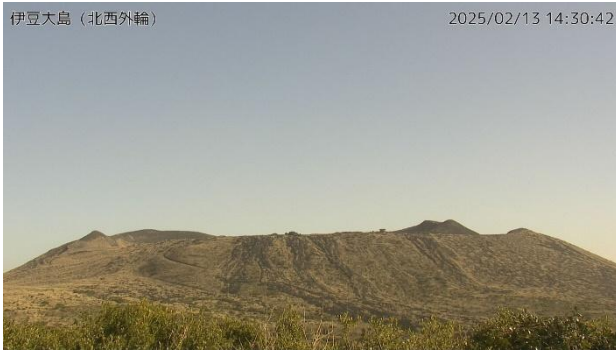
山頂部（2月13日、北西外輪監視カメラによる）
