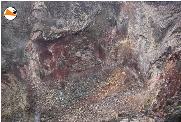
中央火孔東カメラ位置からの可視画像 （2024年2月19日 現地調査時に撮影）
