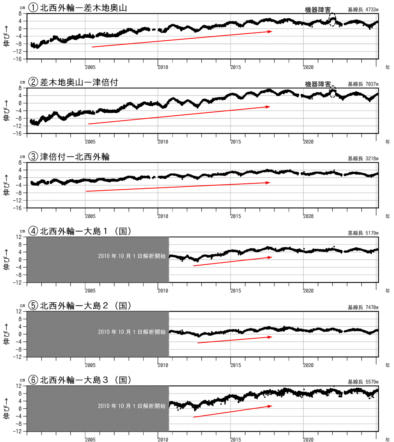
図 3-1 伊豆大島 GNSS 連続観測による基線長変化(2001 年 1 月～2025 年 2 月 28 日)
