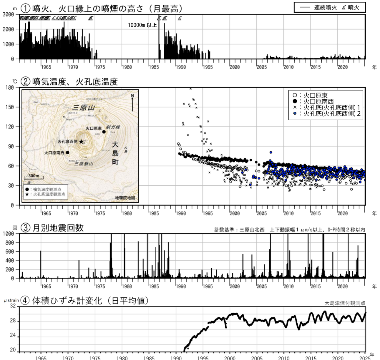
図1 伊豆大島 長期間の火山活動経過図（1961年1月～2025年2月28日）
