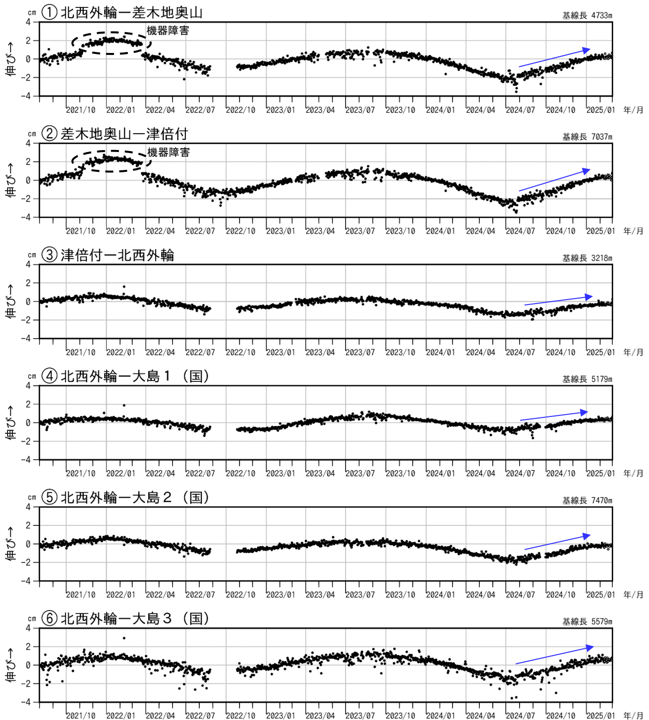
図 3-2 伊豆大島 GNSS 連続観測による基線長変化(2021 年 8 月～2025 年 2 月 28 日)
