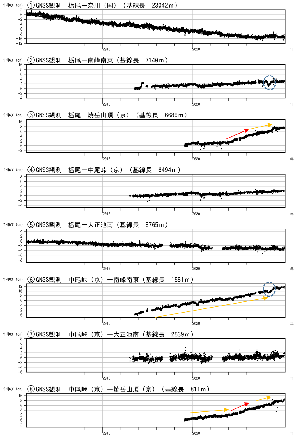
図5 焼岳 GNSS 連続観測による基線長変化 (2010年10月1日～2025年3月3日)
