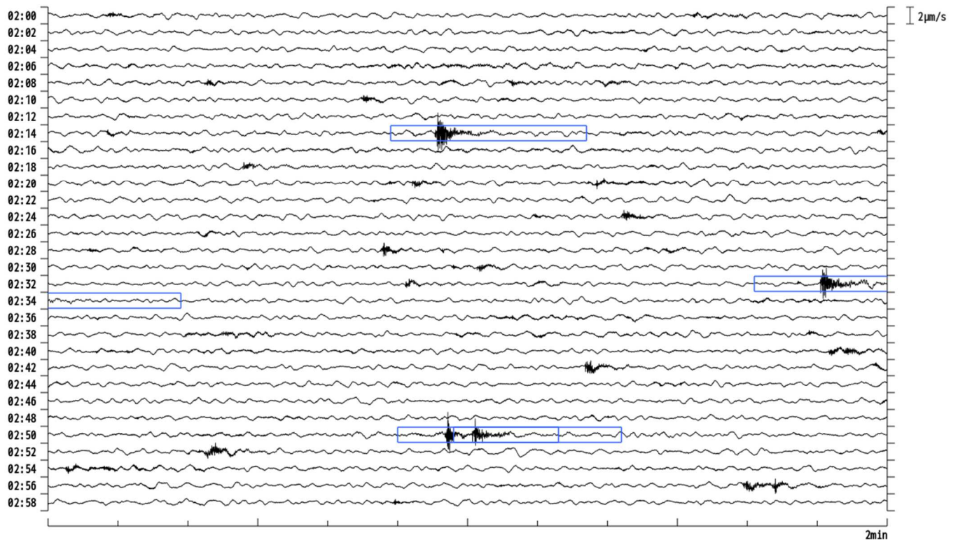
図3 焼岳 本日（4日）02時台に観測された火山性地震
