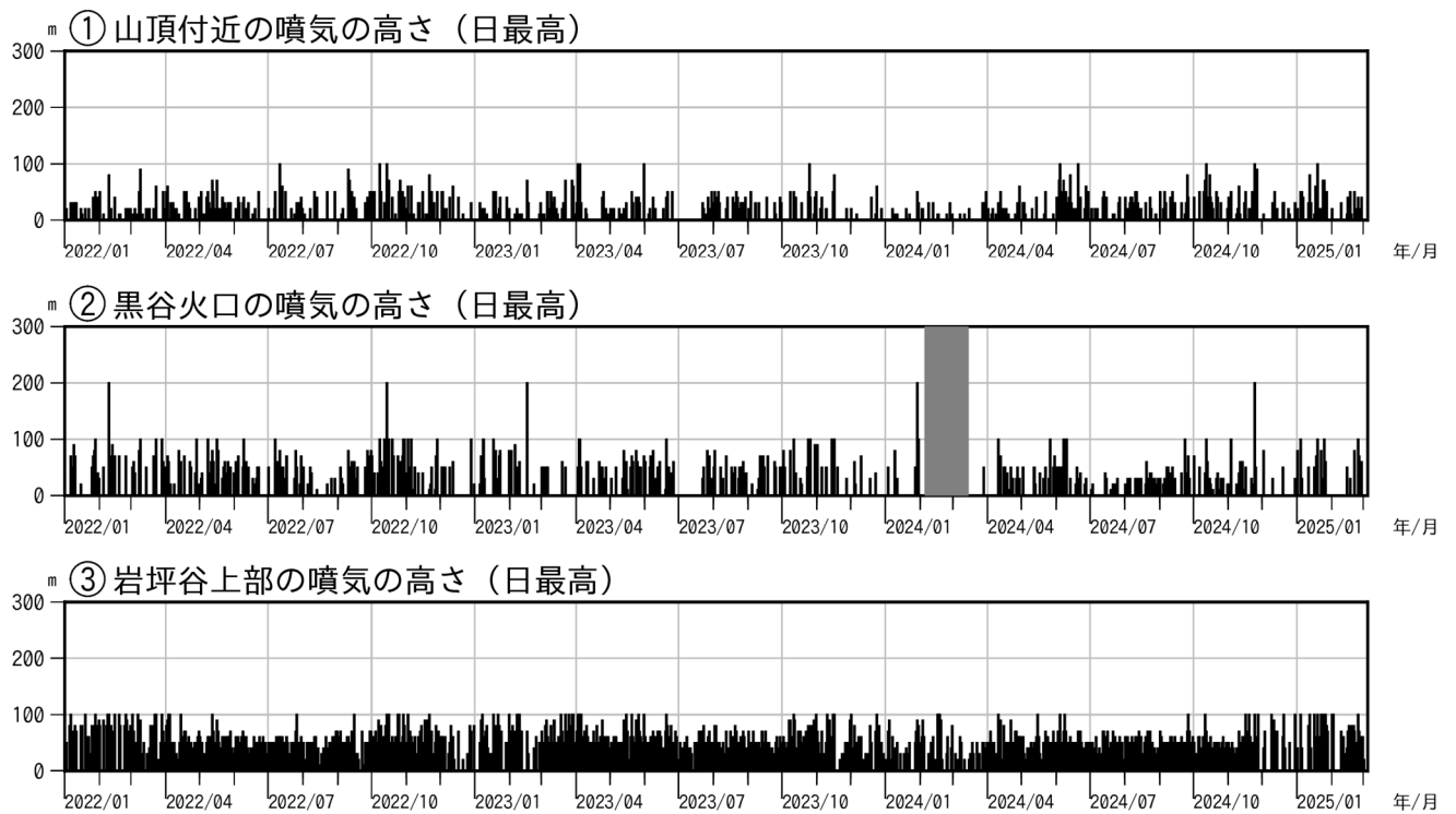
図4-1 焼岳 噴気の高さの推移（2022年1月1日～2025年3月3日）
