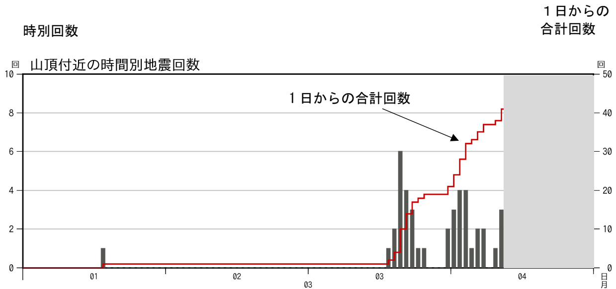
図2 焼岳 山頂付近の時別及び1日からの合計地震回数 (2025年3月1日～4日09時まで)
