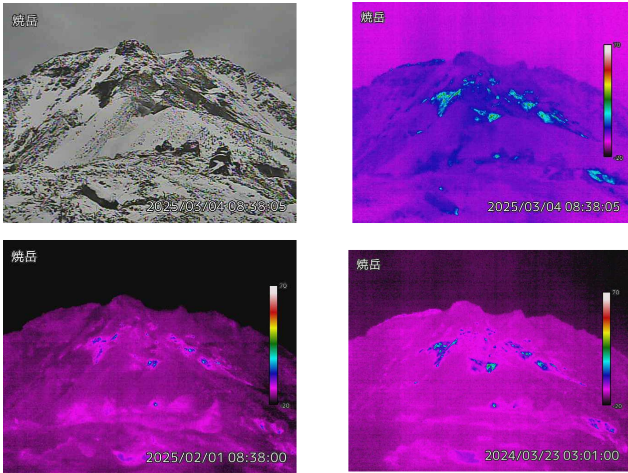
図4—2 焼岳 中尾峠赤外熱映像カメラによる焼岳の北側斜面の地表面温度分布と可視画像 ・前月（左下図）及び前年（右下図）と比較して、噴気の状態や地表面温度分布に明瞭な変化はありません。
