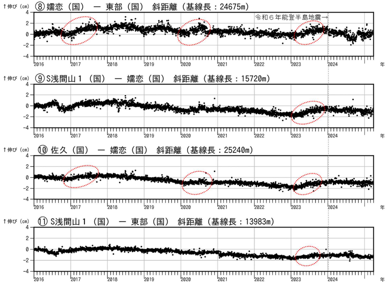
図7-2 浅間山 GNSS 連続観測結果 (2016年1月1日～2025年3月31日)
