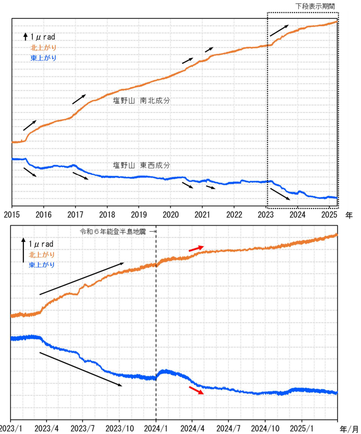
図6 浅間山 塩野山観測点における傾斜データ（2015年1月1日～2025年3月31日）
