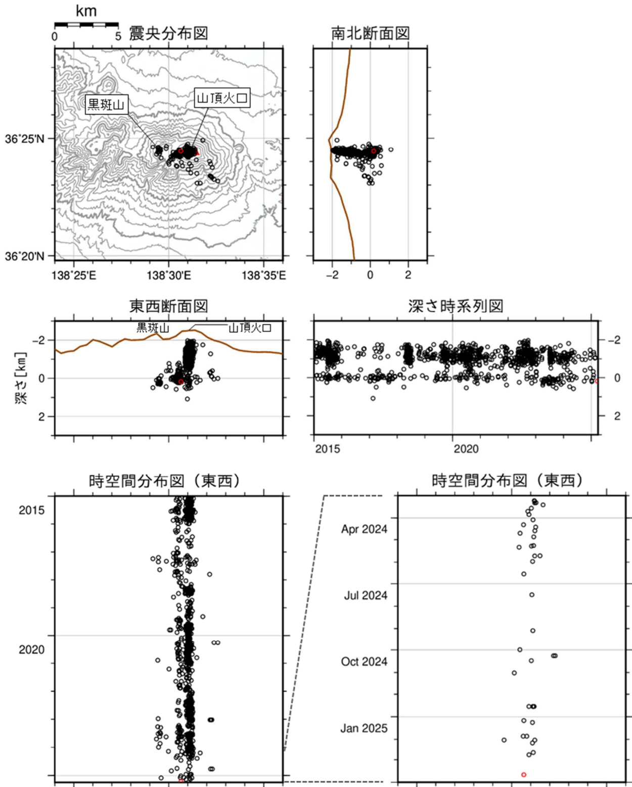
図5 浅間山 震源分布図（2015年1月1日～2025年3月31日）
