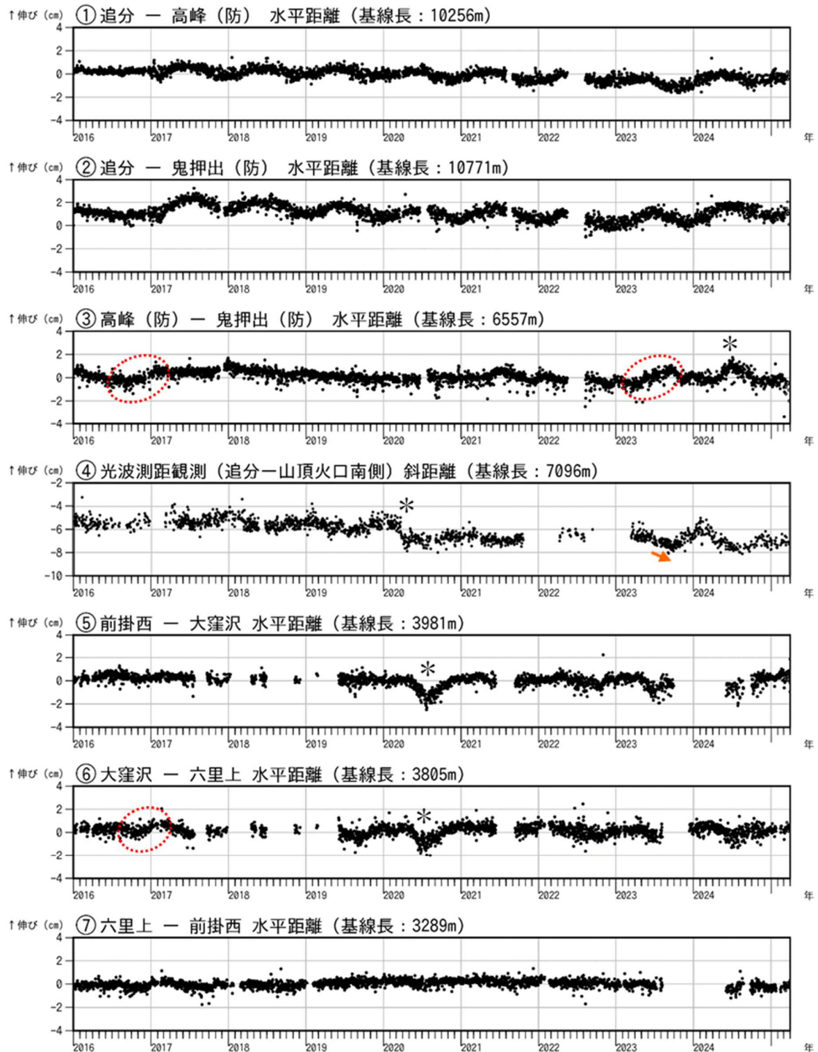
図7-1 浅間山 GNSS 連続観測及び光波測距観測結果(2016年1月1日～2025年3月31日)
