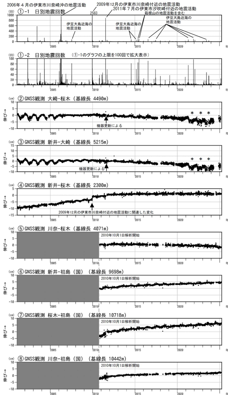
図3 伊豆東部火山群 火山活動経過図 (2001年2月1日～2025年3月31日)
