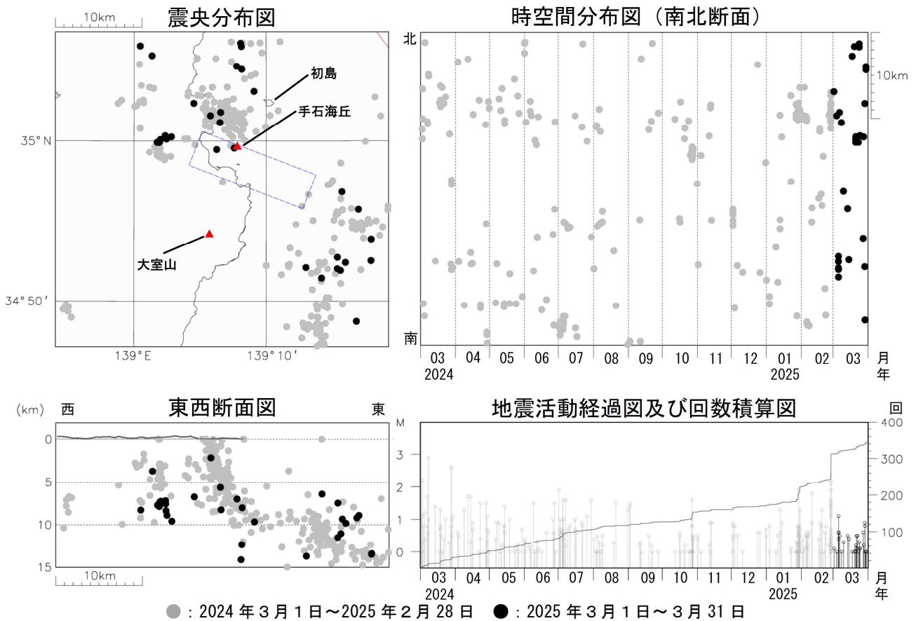
図2 伊豆東部火山群 広域地震観測網による震源分布図（2024 年 3 月 1 日～2025 年 3 月 31 日） □ の領域は群発地震活動の発生する可能性がある範囲（火口が出現する可能性のある範囲）を示しています。 https://www.data.jma.go.jp/vois/data/filing/level/PDF/level_316.pdf 広域地震観測網により震源決定したもので、深さは全て海面以下として決定しています。 M（マグニチュード）は地震の規模を表し、M0.0 以上を表示しています。 図中の震源要素は一部暫定値が含まれており、後日変更することがあります。 この図では、関係機関の地震波形を一元的に処理し、地震観測点の標高を考慮する等した手法で得られた震源を用いています。
