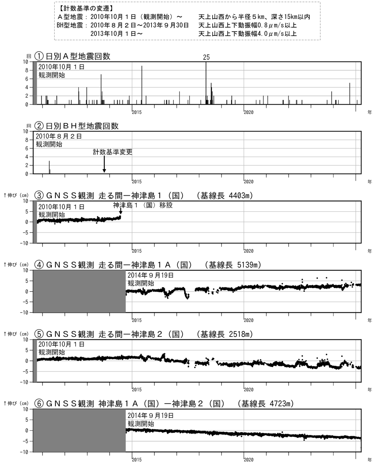
図2 神津島 火山活動経過図(2010年8月2日～2025年3月31日)
