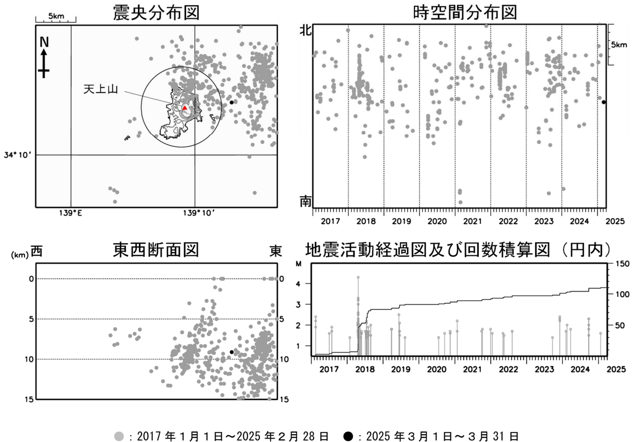
図3 神津島 広域地震観測網による山体・周辺の地震活動（2017年1月1日～2025年3月31日） 広域地震観測網により震源決定したもので、深さは全て海面以下として決定しています。なお、2020年9月以降については、地震観測点の標高を考慮する等、震源決定の手法を変更しております。 M（マグニチュード）は地震の規模を表し、M1.4以上の地震を示しています。 図中の震源要素は一部暫定値が含まれており、後日変更することがあります。 計数対象（天上山西から半径約5km、深さ約15km以内）以外の地震が含まれるため、図2－①の日別A型地震回数とは異なります。 震央分布図中の円は火山性地震の回数の計数対象（天上山西から半径5km、深さ15km以内）の範囲を示しています。 ・地震活動は低調に経過しました。
