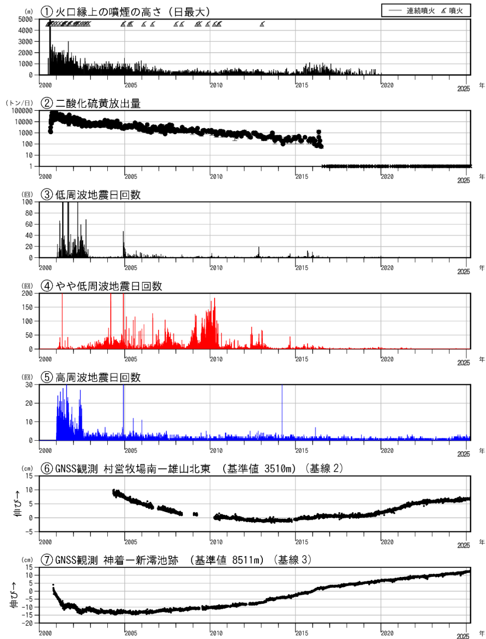
図7 三宅島 長期の火山活動経過図（2000年1月1日～2025年3月31日）
