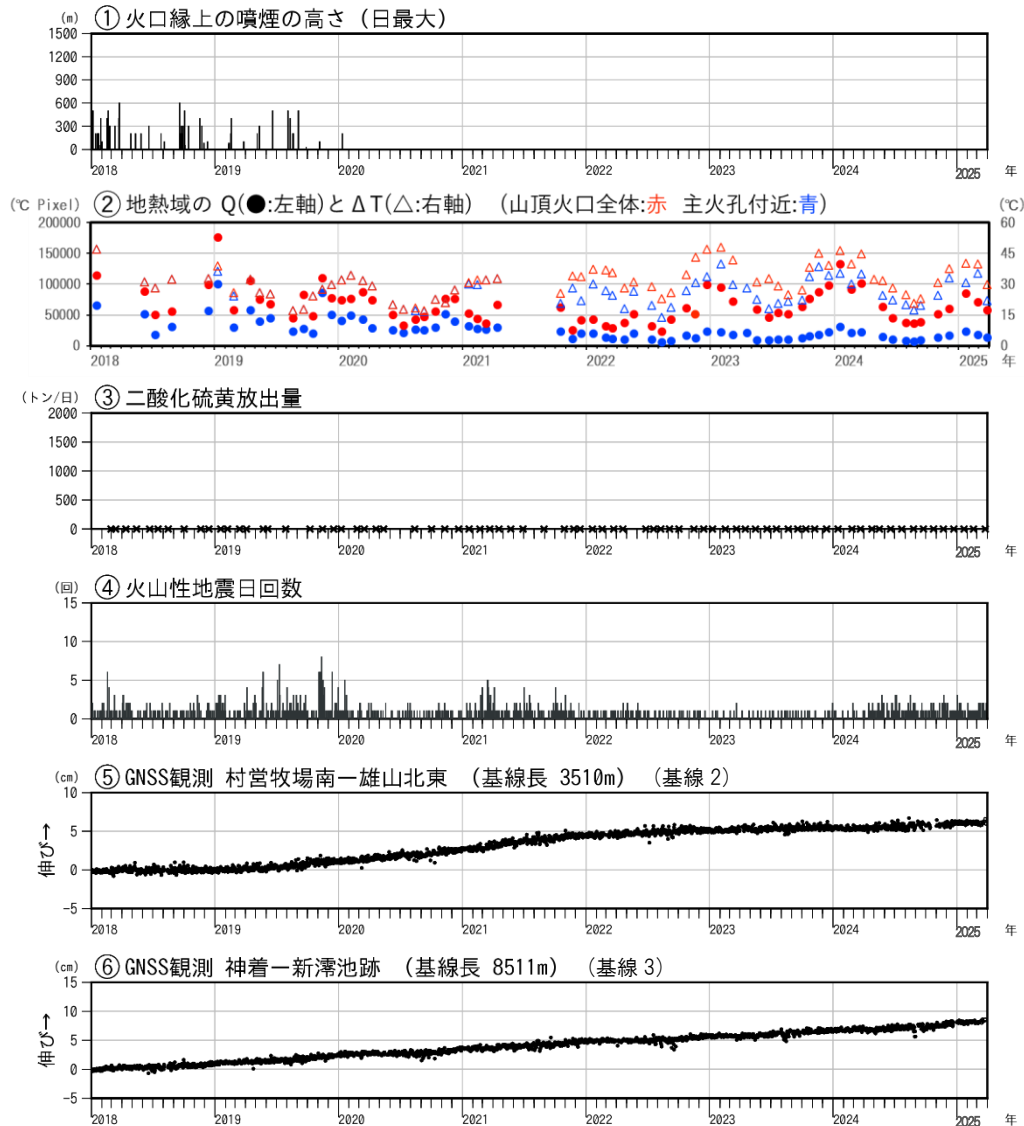
図6 三宅島 火山活動経過図（2018年1月1日～2025年3月31日）
