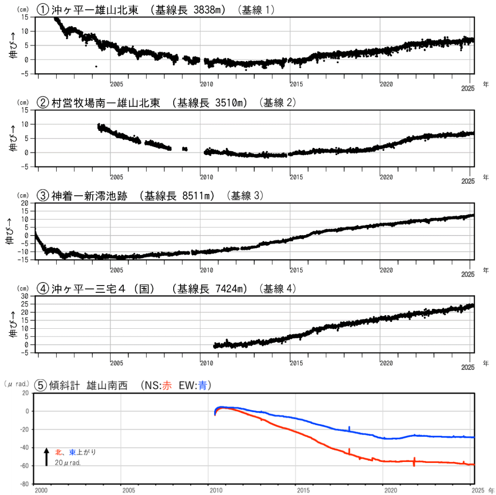
図8 三宅島 GNSS 連続観測及び傾斜計観測結果（2000年10月26日～2025年3月31日）
