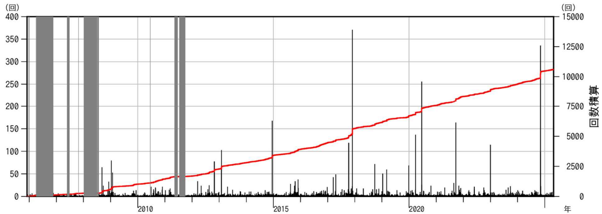
図3 白山 日別地震回数と積算回数（2005年12月1日～2025年4月30日）
