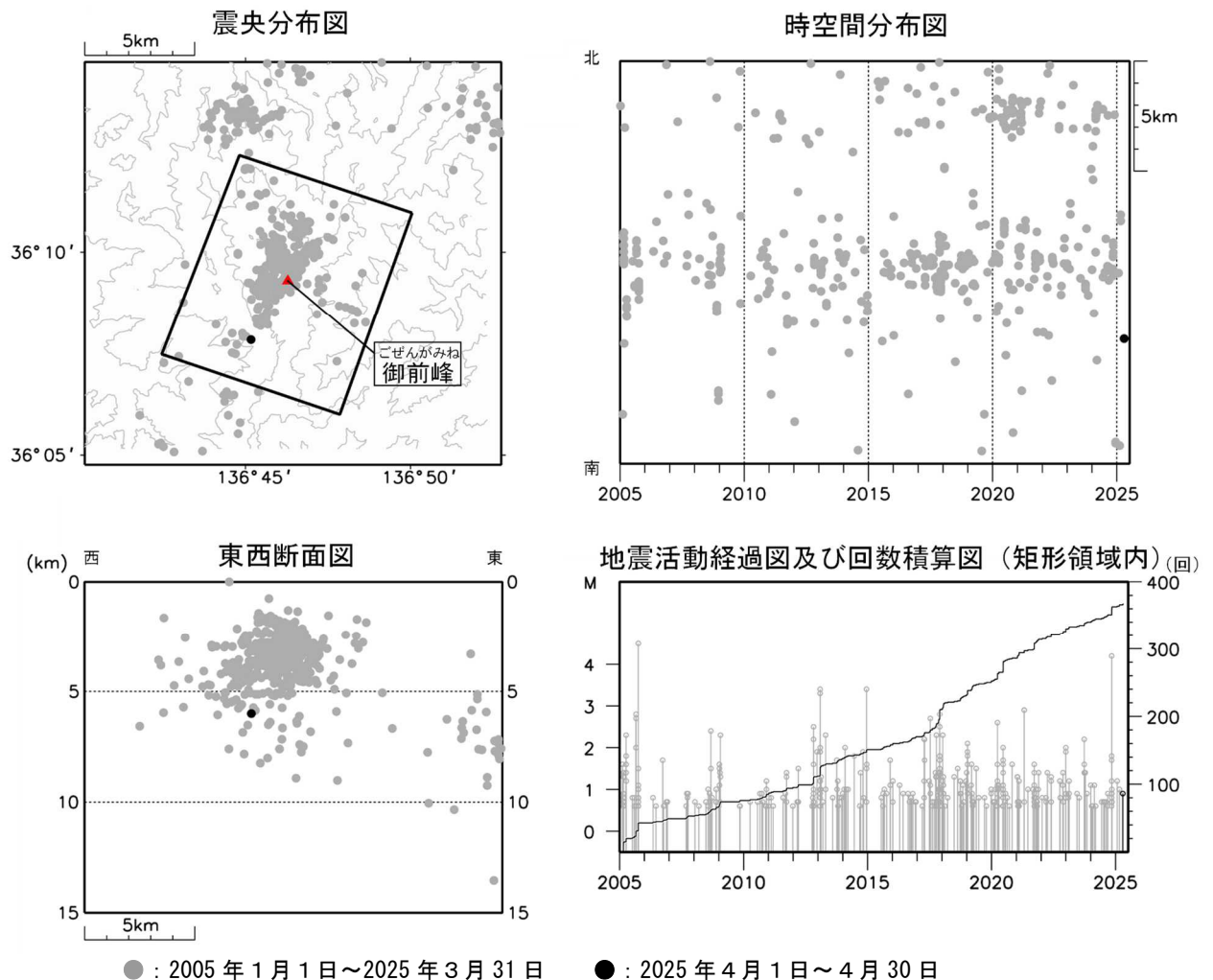
図4 白山 広域地震観測網による山体・周辺の地震活動（2005年1月1日～2025年4月30日）
