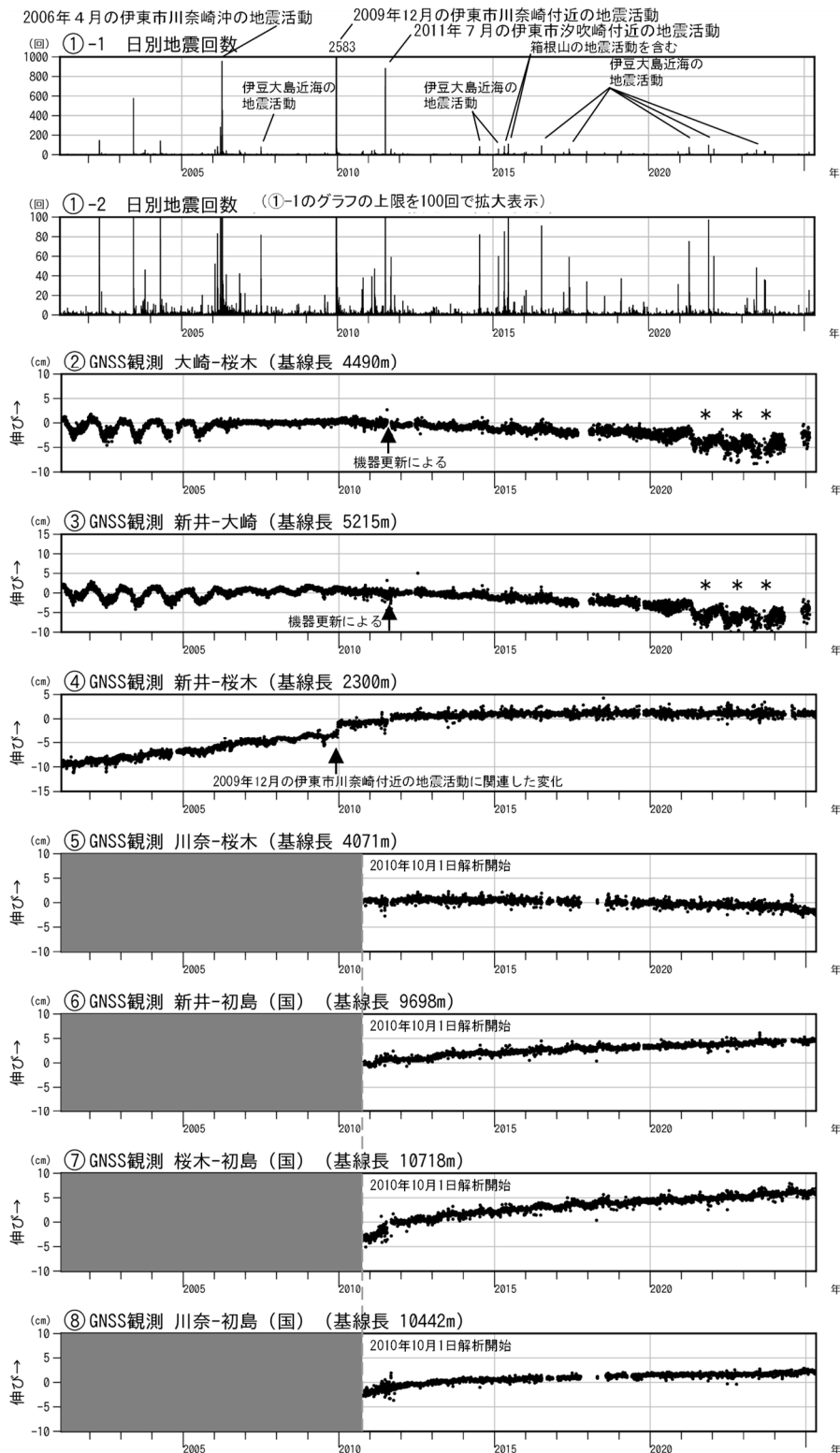
図3 伊豆東部火山群 火山活動経過図 (2001年2月1日~2025年4月30日)
