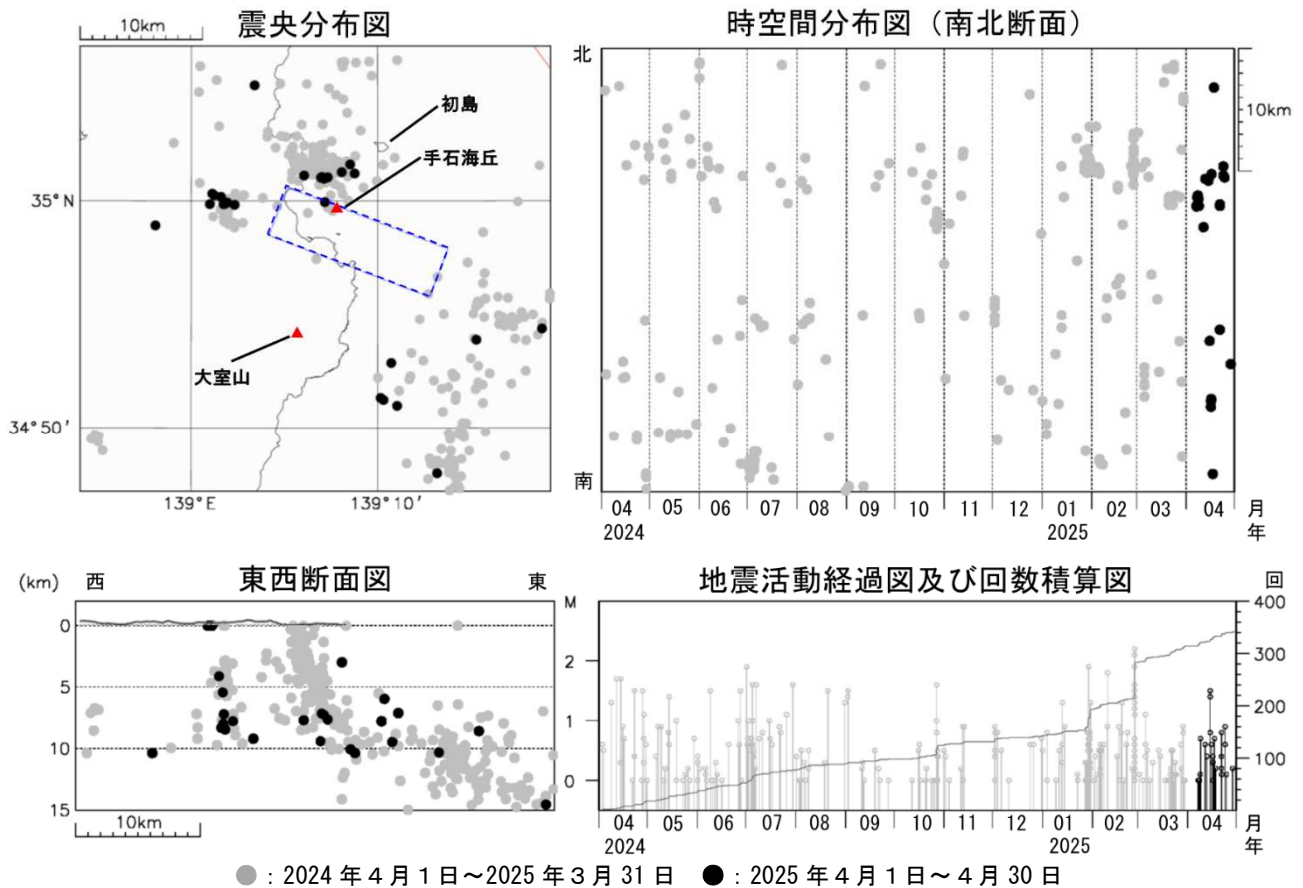
図2 伊豆東部火山群 広域地震観測網による震源分布図（2024 年 4 月 1 日～2025 年 4 月 30 日） □ の領域は群発地震活動の発生する可能性がある範囲（火口が出現する可能性のある範囲）を示しています。 https://www.data.jma.go.jp/vois/data/filing/level/PDF/level_316.pdf 広域地震観測網により震源決定したもので、深さは全て海面以下として決定しています。 M（マグニチュード）は地震の規模を表し、M0.0 以上を表示しています。 図中の震源要素は一部暫定値が含まれており、後日変更することがあります。 この図では、関係機関の地震波形を一元的に処理し、地震観測点の標高を考慮する等した手法で得られた震源を用いています。
