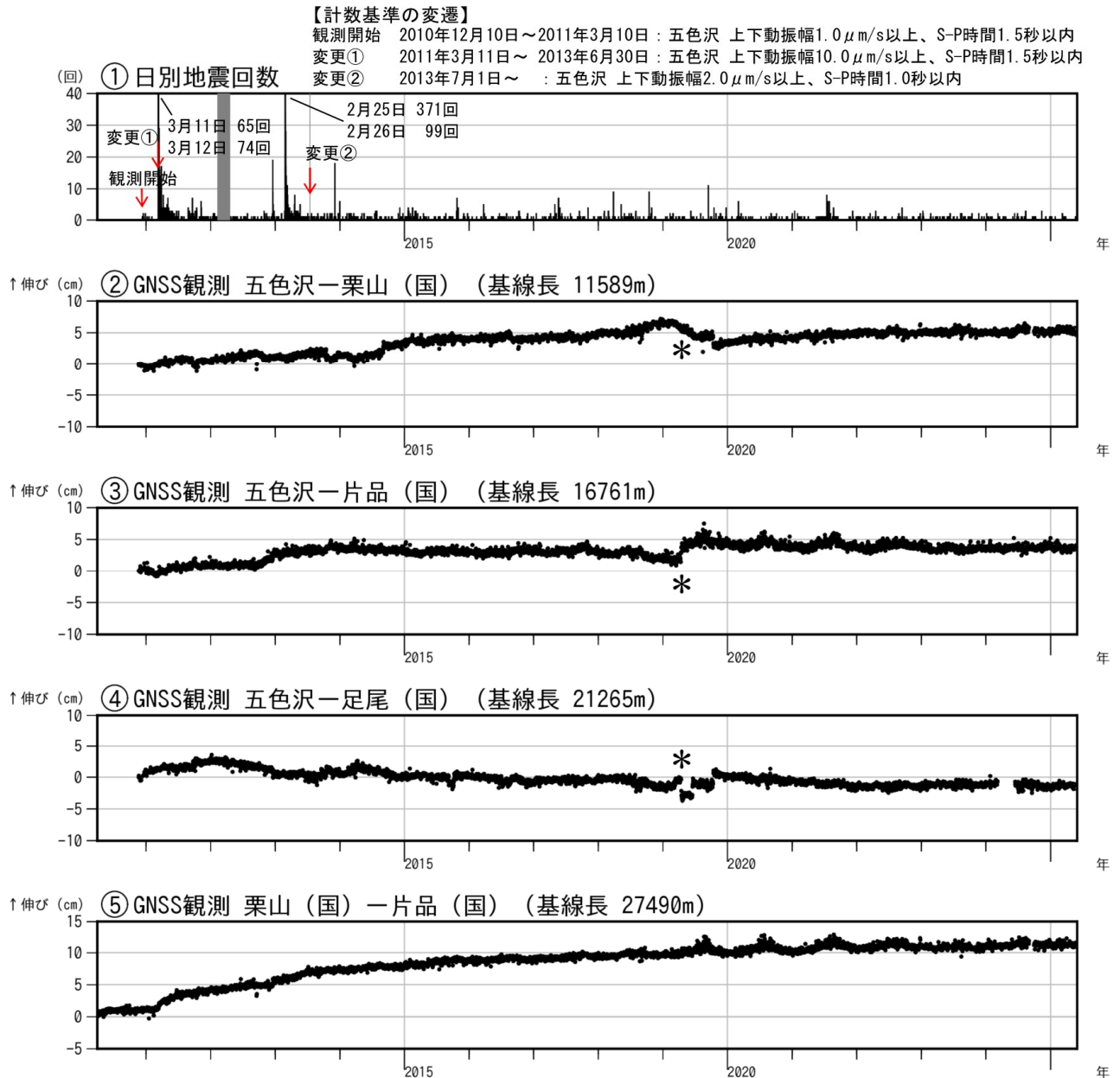
図 2 日光白根山 火山活動経過図（2010 年 4 月 1 日～2025 年 5 月 31 日）
