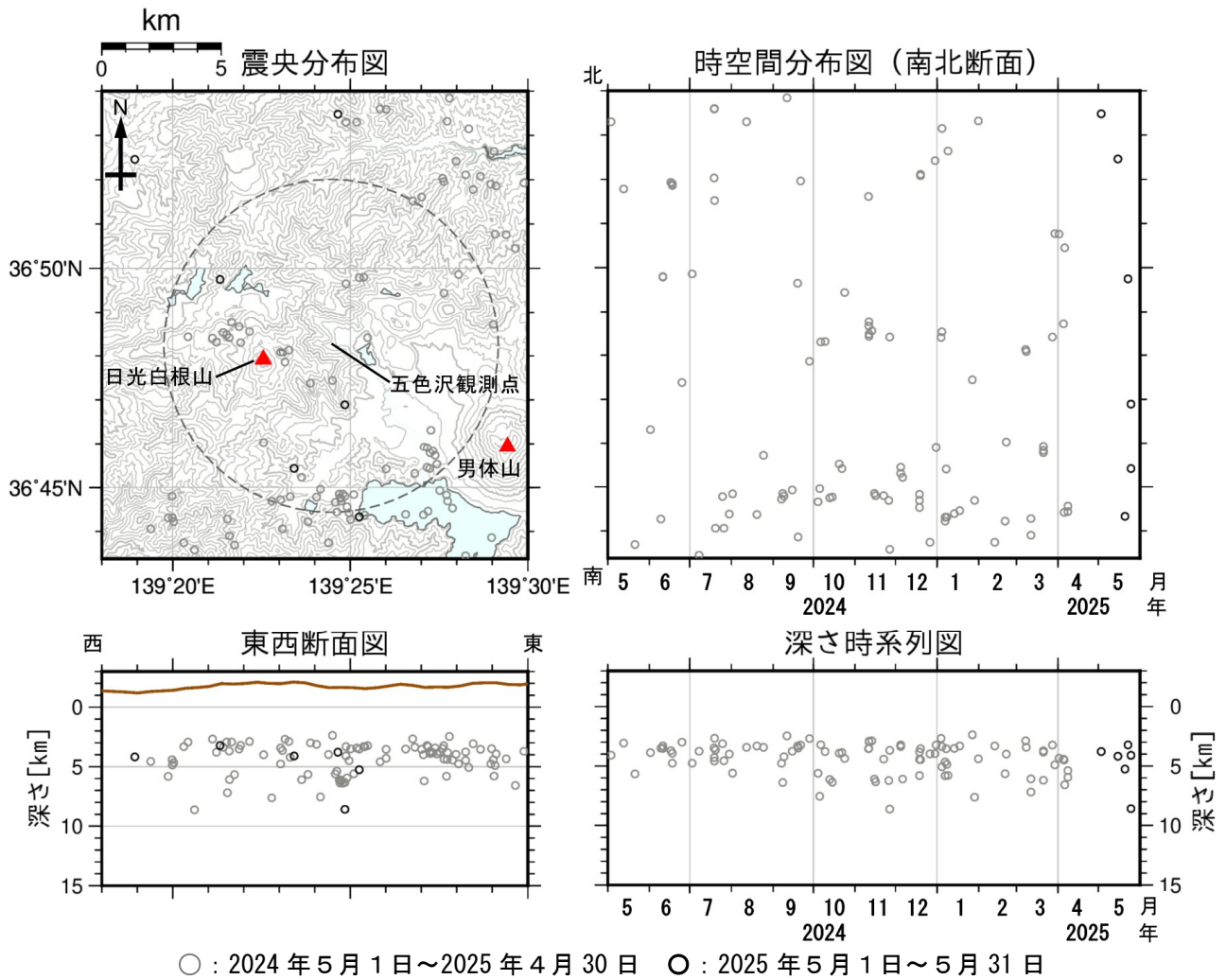
図3 日光白根山 広域地震観測網による山体周辺の地震活動 (2024 年 5 月 1 日～2025 年 5 月 31 日)
