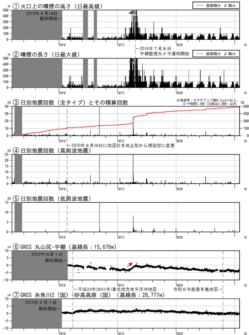
図2 新潟焼山 火山活動経過図（2006年1月1日～2025年5月31日）
