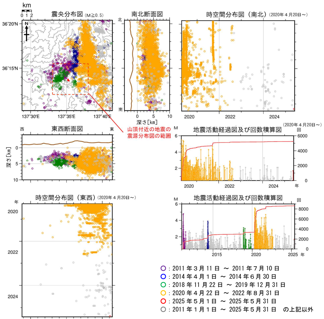
図9 焼岳 広域地震観測網による山体及び周辺の地震活動(2011年1月1日～2025年5月31日)
