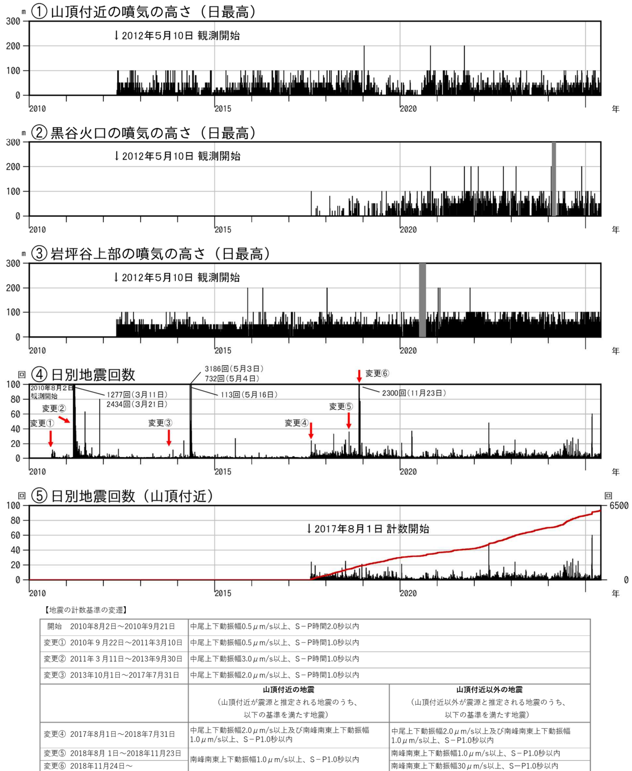
図5 焼岳 噴気の高さと地震回数の推移(2010年8月2日～2025年5月31日)
