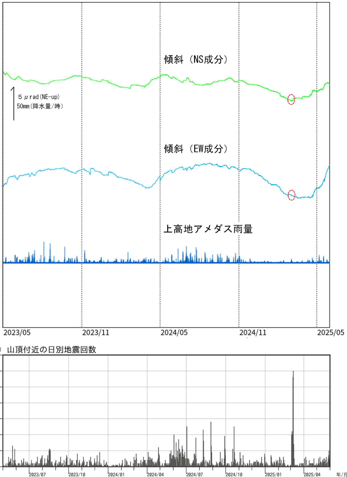
図8 焼岳 南峰南東観測点における傾斜データ（2023年5月1日～2025年5月31日）
