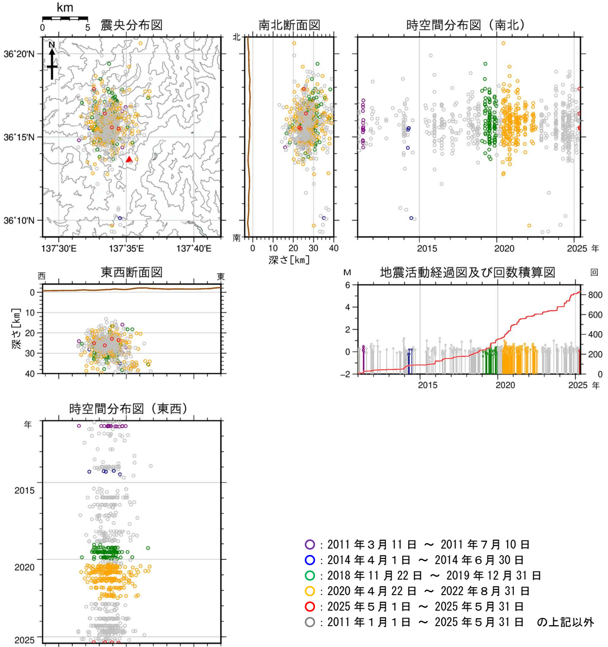
図10 焼岳 広域地震観測網による深部低周波地震の震源分布図（2011年1月1日～2025年5月31日） 広域地震観測網により震源決定したもので、深さは全て海面以下として決定しています。なお、2020年9月以降については、地震観測点の標高を考慮する等、震源決定の手法を変更しています。 M（マグニチュード）は地震の規模を表します。 図中の震源要素は一部暫定値が含まれており、後日変更することがあります。
