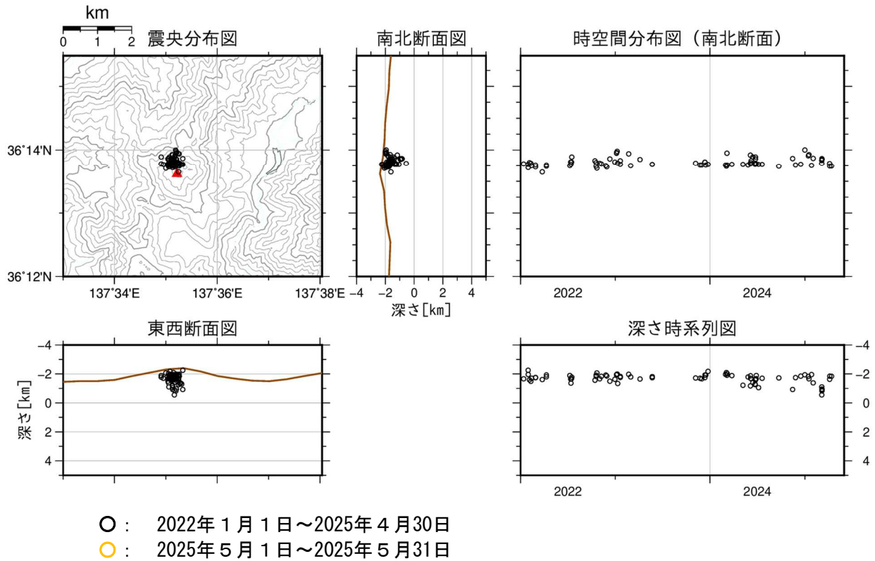
図2 焼岳 山頂付近の地震の震源分布図（2022年1月1日～2025年5月31日）
