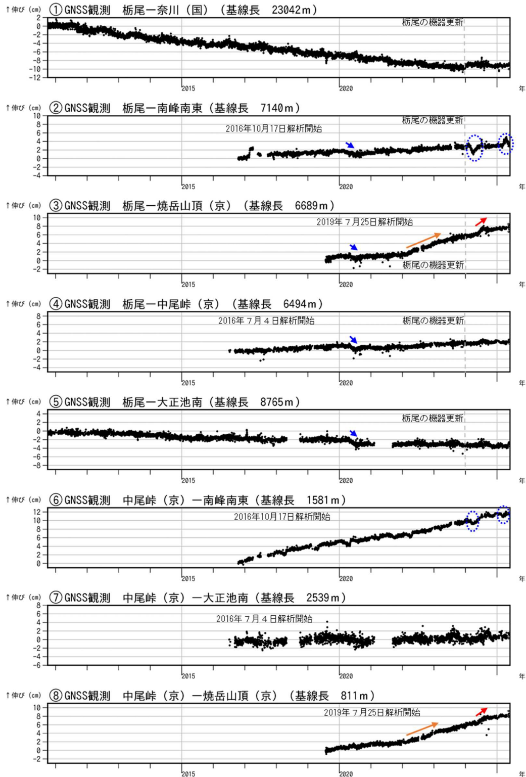
図6 焼岳 GNSS 連続観測による基線長変化（2010 年 10 月 1 日～2025 年 5 月 31 日）
