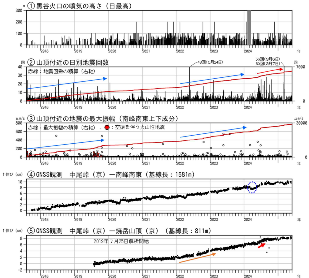
図1 焼岳 火山活動経過図（2017年8月1日～2025年5月31日）
