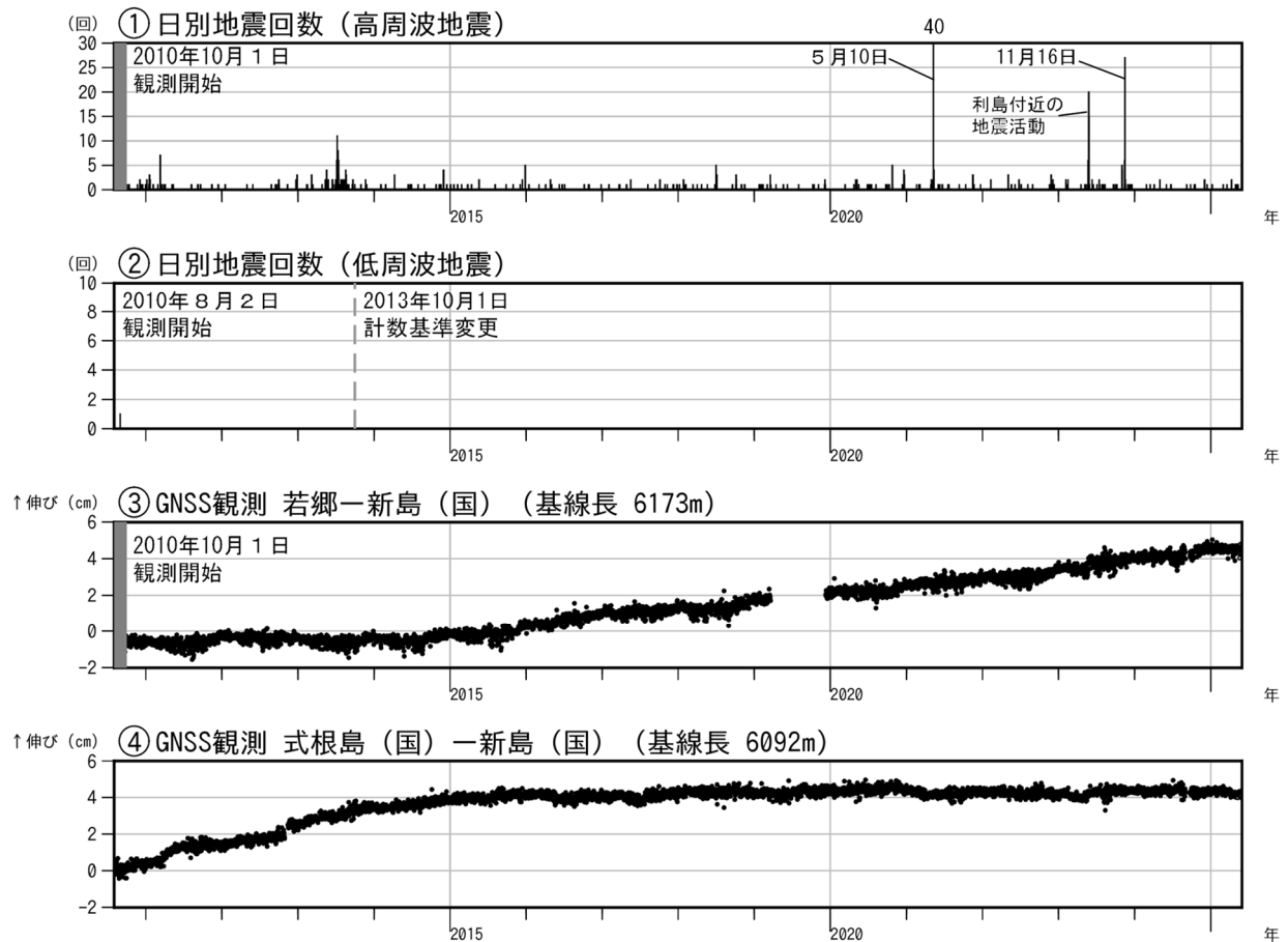
図2 新島 火山活動経過図(2010年8月2日～2025年5月31日)
