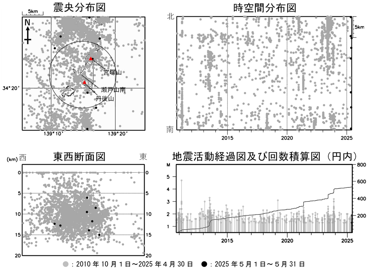
図3 新島 広域地震観測網による山体・周辺の地震活動（2010年10月1日～2025年5月31日） 広域地震観測網により震源決定したもので、深さは全て海面以下として決定しています。なお、2020年9月以降については、地震観測点の標高を考慮する等、震源決定の手法を変更しています。 M（マグニチュード）は地震の規模を表し、M1.3以上の地震を示しています。 図中の震源要素は一部暫定値が含まれており、後日変更することがあります。 計数対象（瀬戸山南から半径約8km、深さ約20km以内）以外の地震が含まれるため、図2-①の日別地震回数（高周波地震）とは異なります。 震央分布図中の円は火山性地震の回数の計数対象（瀬戸山南から半径8km、深さ20km以内）の範囲を示しています。 ・地震活動は低調に経過しました。
