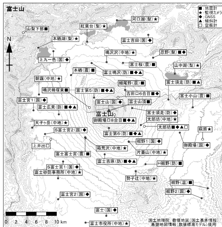
図6 富士山 観測点配置図
