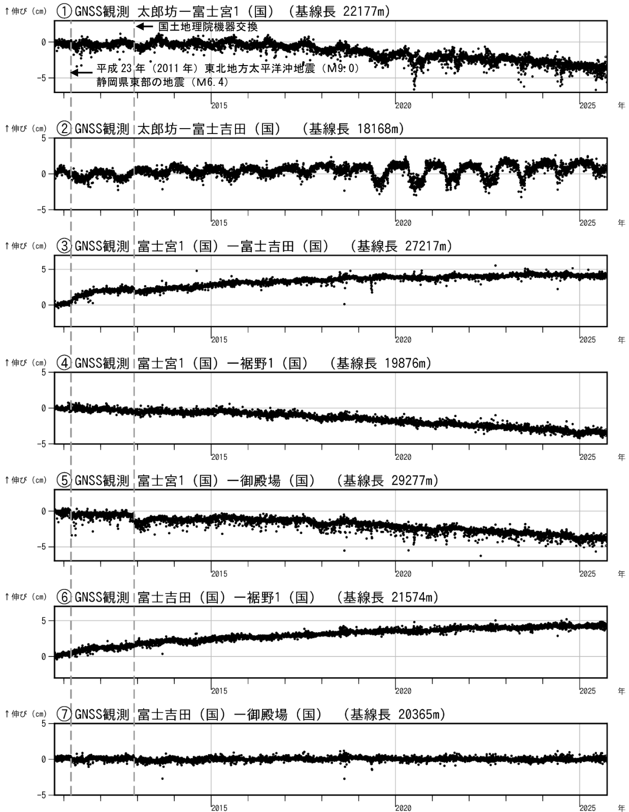
図4 富士山 GNSS 連続観測による基線長変化 (2010 年 10 月 1 日～2025 年 9 月 30 日)
