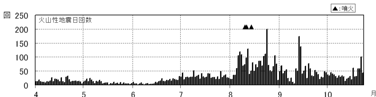
図3 浅間山 火山性地震の日別回数（2008年4月1日～2008年10月23日）
