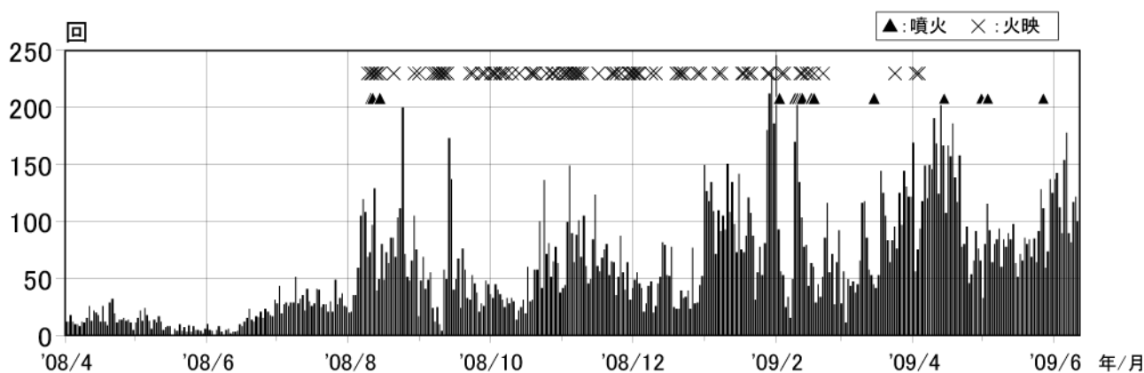
図2 浅間山 火山性地震の日別回数（2008年4月1日～2009年6月11日）
