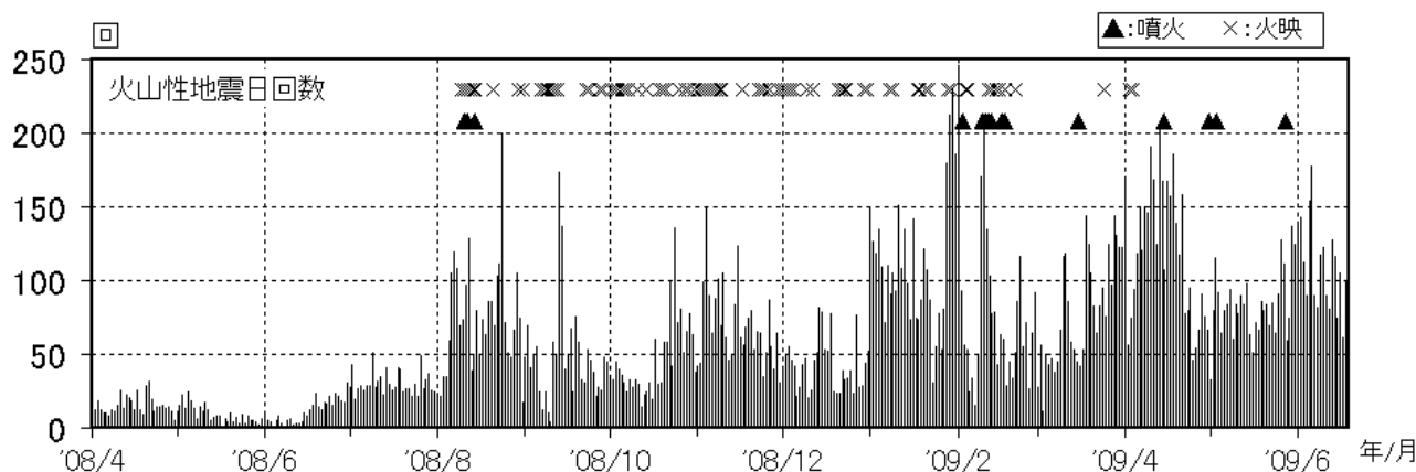
図2 浅間山 火山性地震の日別回数（2008 年4月1日～2009 年6月25日）
