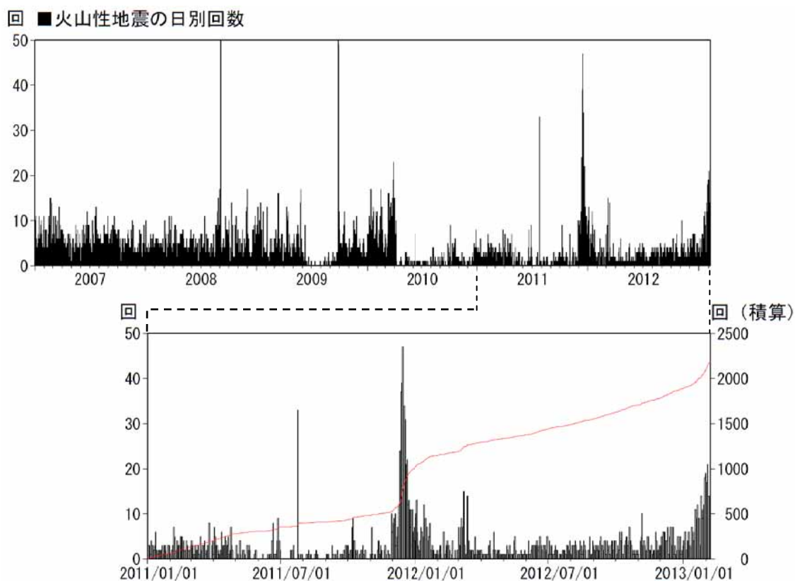
図2 口永良部島 火山性地震の発生回数（2007年1月1日～2013年2月7日）
