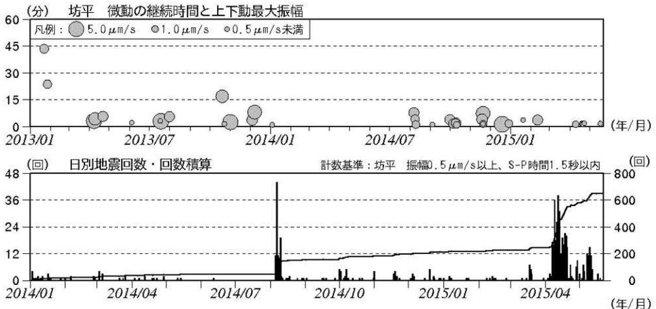
図2 蔵王山 火山性地震の発生状況（2014年1月1日～2015年5月21日）
