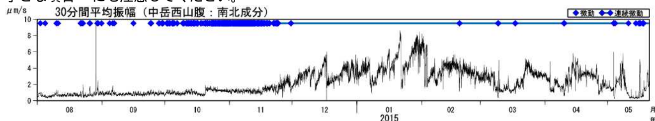
図7 阿蘇山 火山性微動の30分間平均振幅（2014年8月1日～2015年5月21日）
