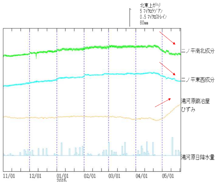
図5 箱根山 湯河原鍛冶屋観測点におけるひずみ変化と箱根山地震活動の推移 (2014年11月1日～2015年5月21日)
