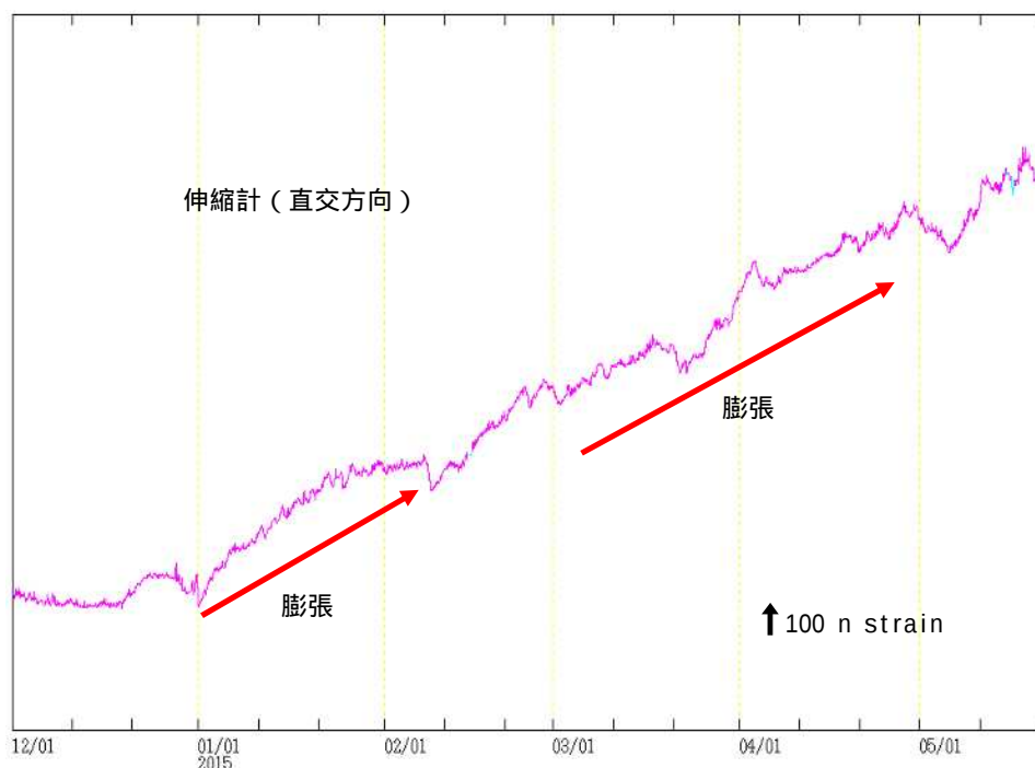
図 8 桜島 有村観測坑道の伸縮変動（2014 年 12 月 1 日～2015 年 5 月 21 日）
