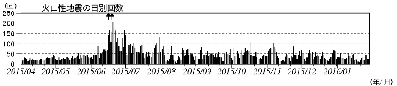
図2 浅間山 火山性地震の日別回数(2015年4月1日～2016年1月28日)(矢印はごく小規模な噴火を示す)
