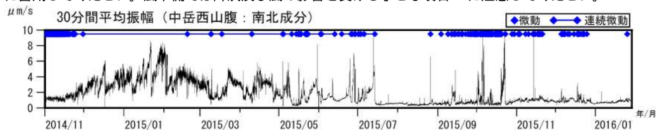
図3 阿蘇山 火山性微動の30分間平均振幅（2014年11月1日～2016年1月28日）
