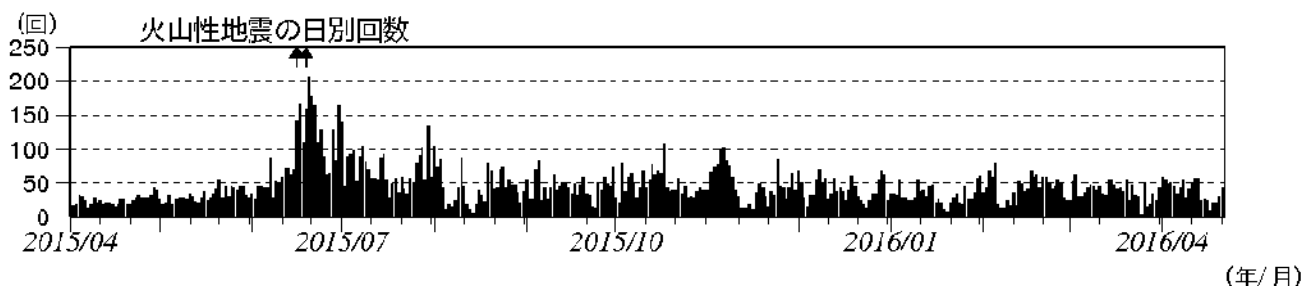
図2 浅間山 火山性地震の日別回数（2015年4月1日～2016年4月21日）（矢印はごく小規模な噴火を示す）
