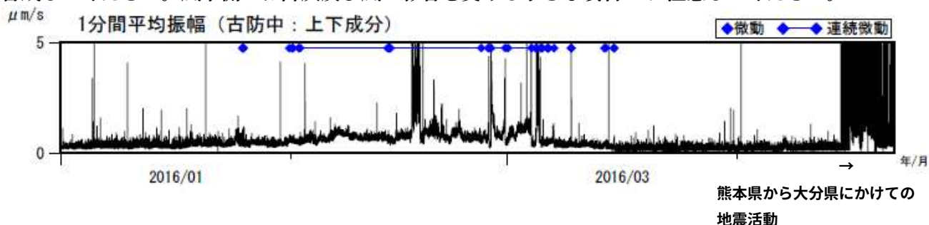
図3 阿蘇山 古防中観測点上下成分の1分間平均振幅（2016年1月1日～2016年4月21日）
