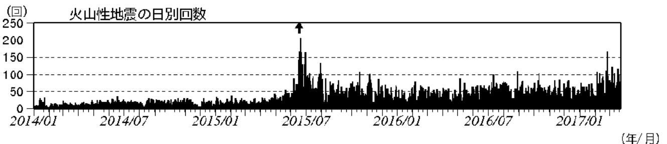
図2 浅間山 火山性地震の日別回数（2014年1月1日～2017年3月23日） （矢印はごく小規模な噴火を示す）
