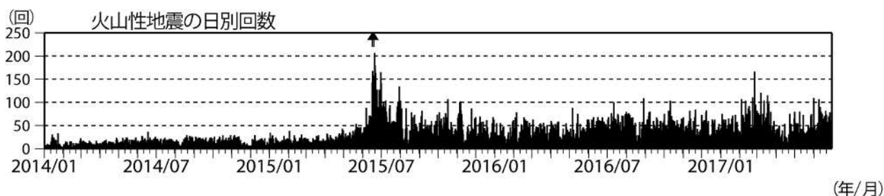
図2 浅間山 火山性地震の日別回数（2014年1月1日～2017年6月29日） （矢印はごく小規模な噴火を示す）
