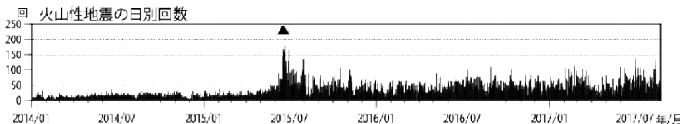
図2 浅間山 火山性地震の日別回数（2014年1月1日～2017年8月24日）
