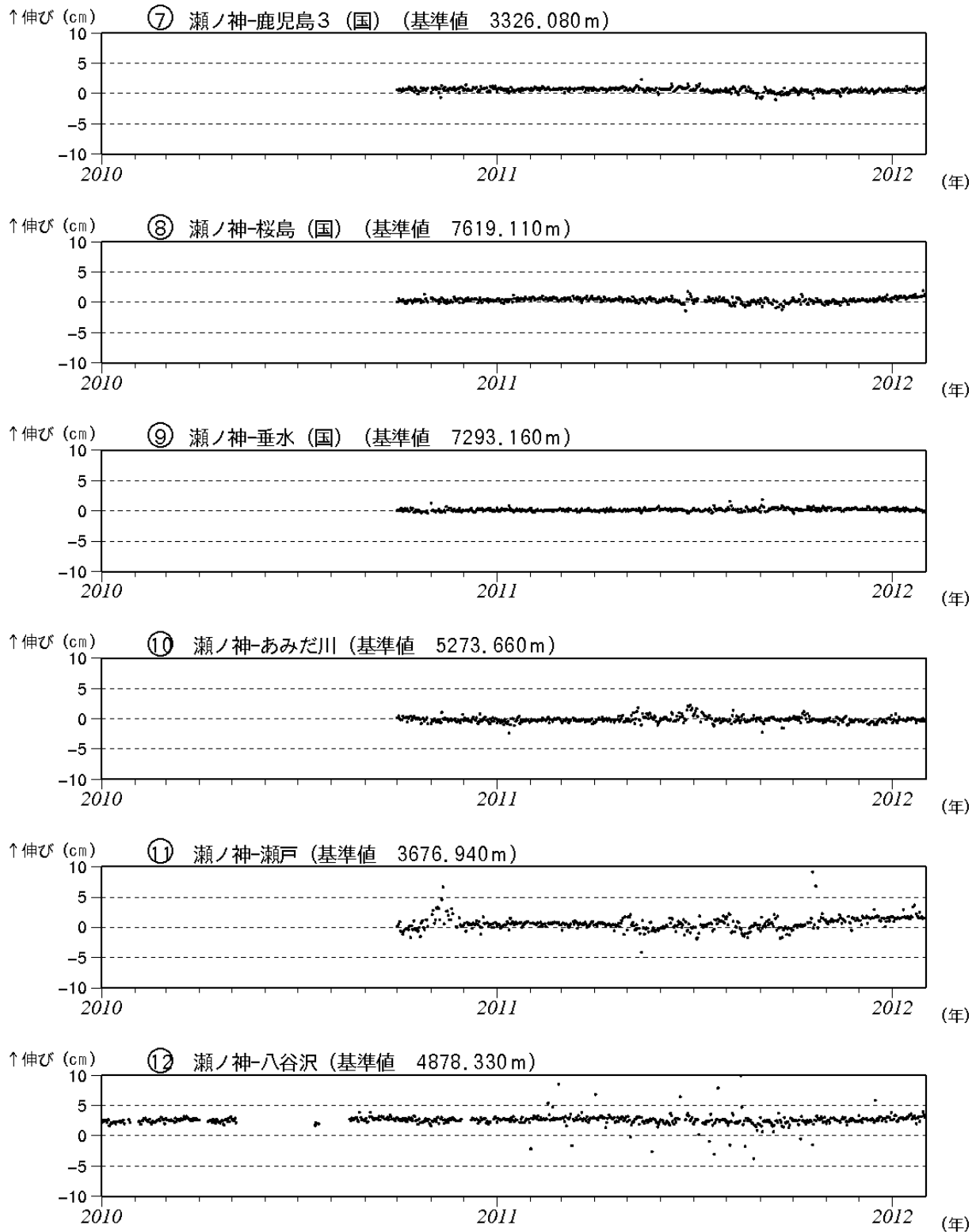
図9※ 桜島 GPS 連続観測による長期の基線長変化（2010 年 10 月～2012 年 1 月）
