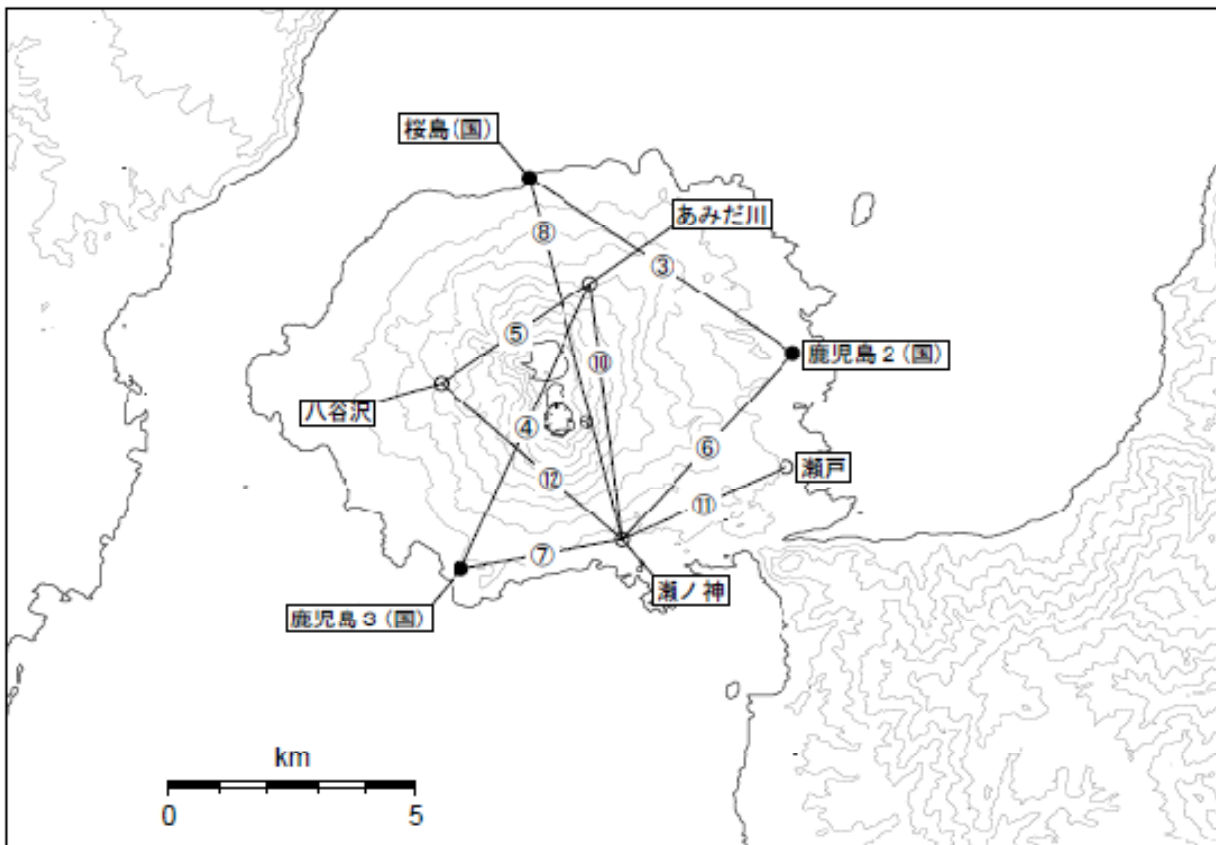
図 10 桜島 GPS 連続観測点と基線番号
