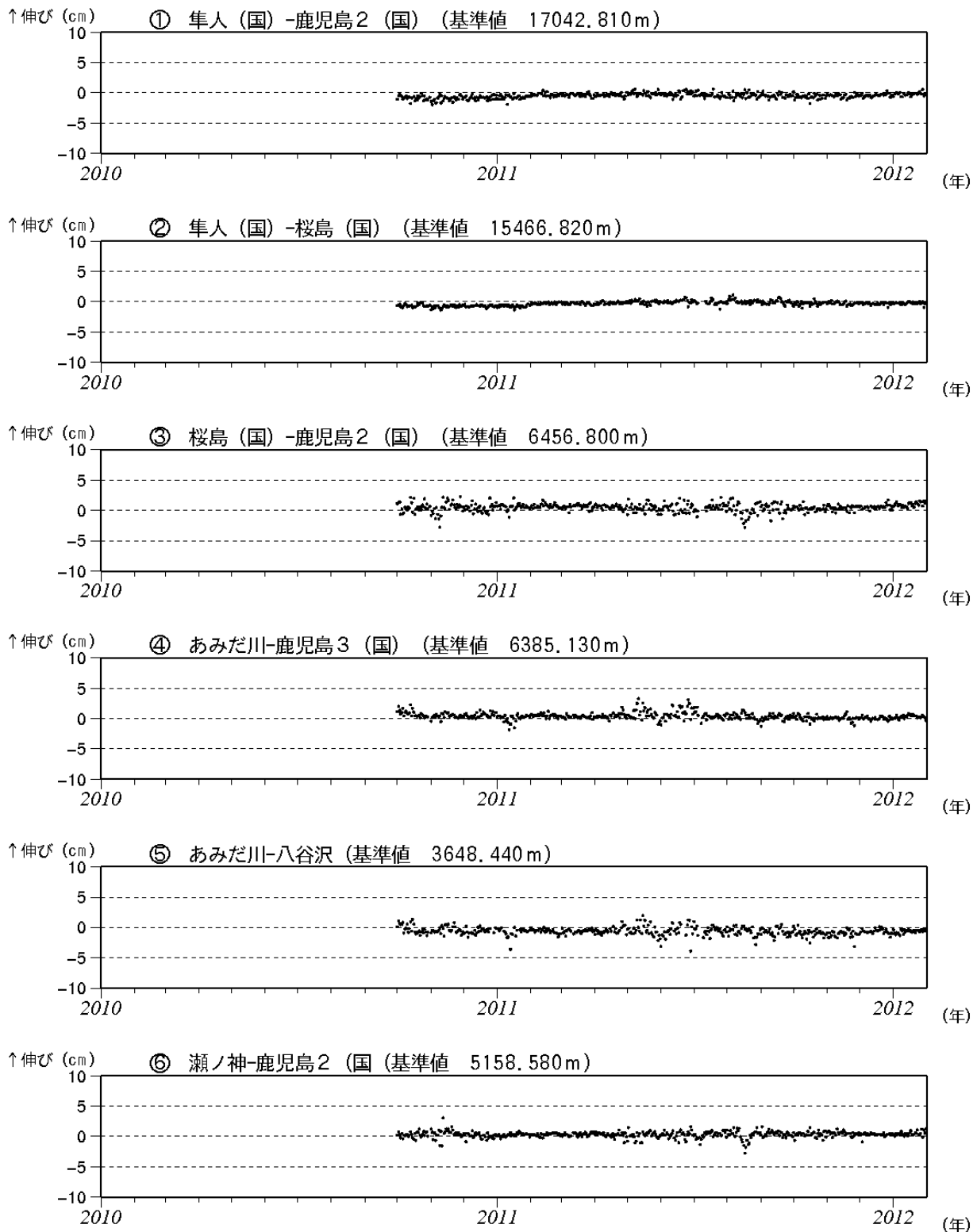
図 8※ 桜島 GPS 連続観測による長期の基線長変化（2010 年 10 月～2012 年 1 月） GPS 連続観測では、2011 年 9 月頃からわずかな伸びの傾向が続いています。
