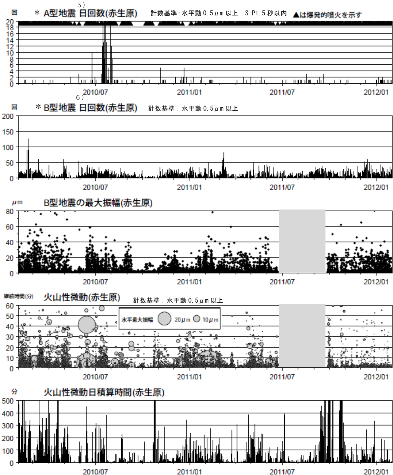
図5 桜島 最近2年間の火山性地震、火山性微動（2010年2月～2012年1月）
