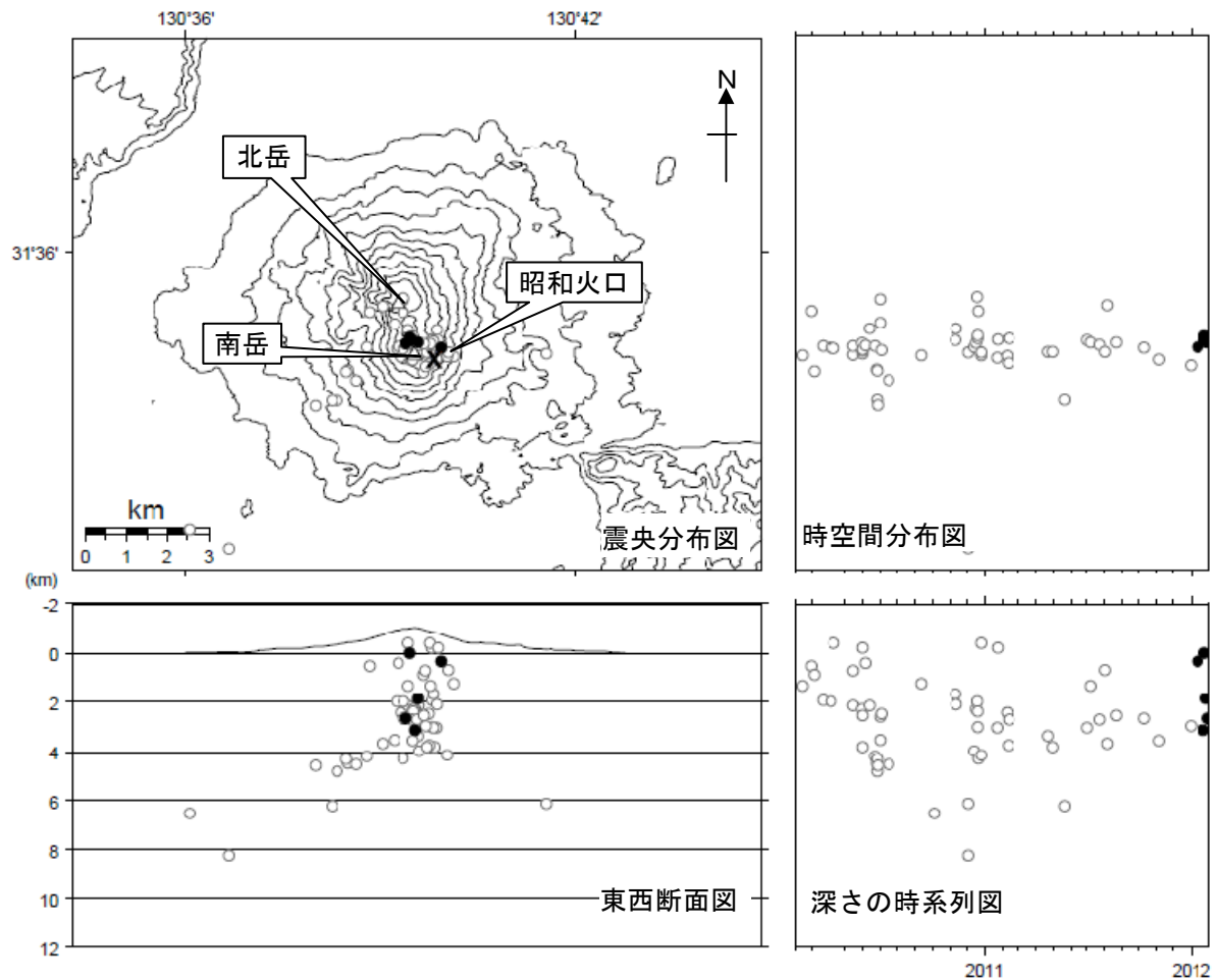
● : 2012 年 1 月の震源 ○ : 2010 年 2 月～2011 年 12 月の震源 図 6※ 桜島 震源分布図（2010 年 2 月～2012 年 1 月）
