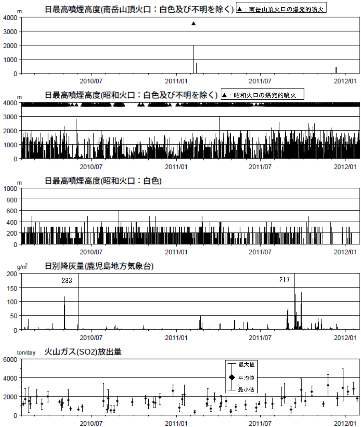
図 4 桜島 最近 2 年間の噴煙、降灰、火山ガス（2010 年 2 月～2012 年 1 月）
