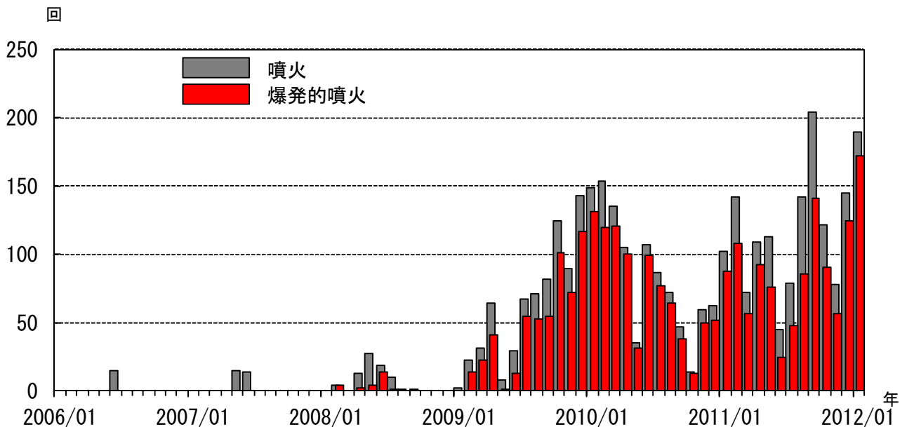
図 3 桜島 昭和火口月別噴火回数（灰色）と昭和火口月別爆発回数（赤色） （2006 年 1 月～2012 年 1 月）
