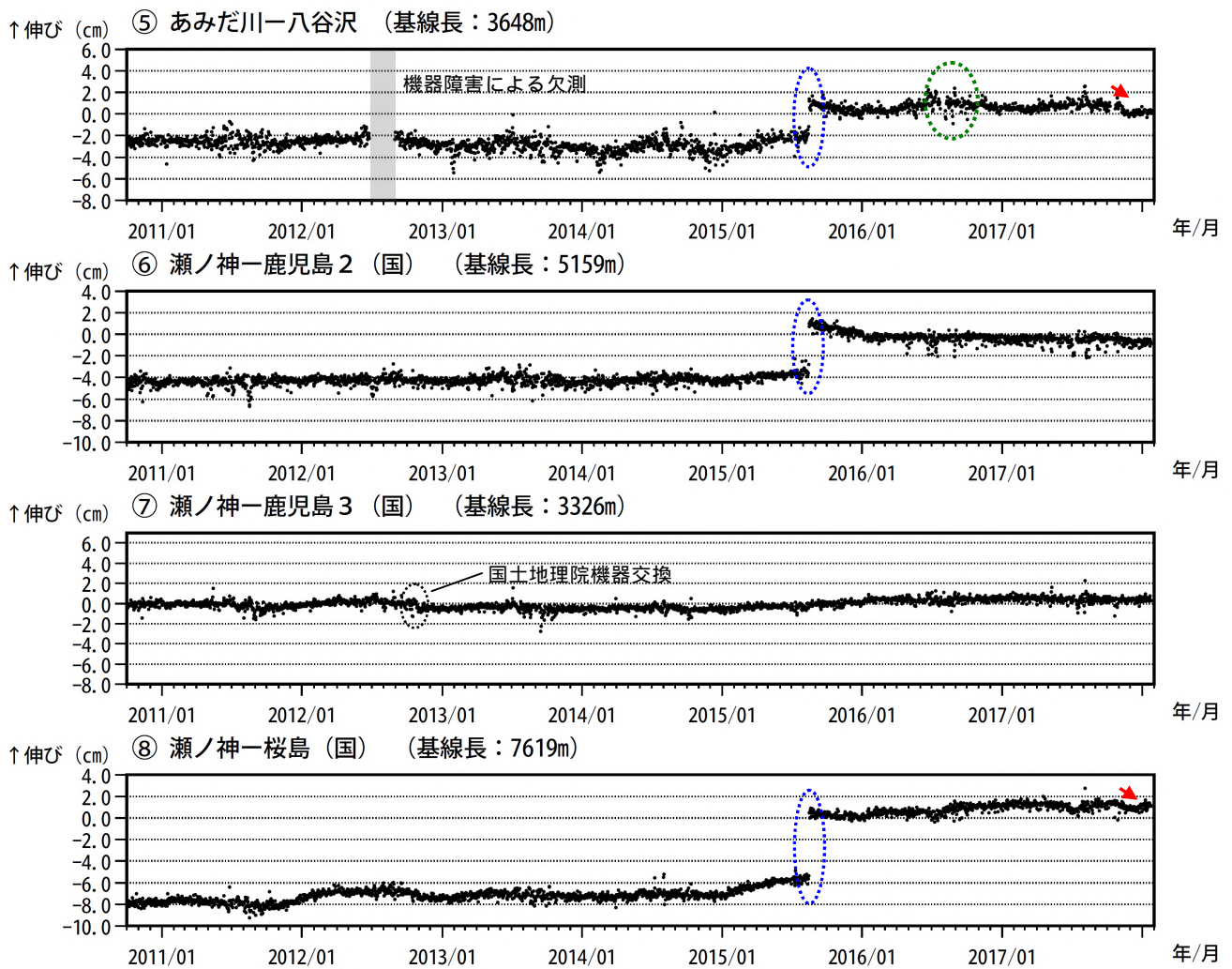
図 7-2 桜島 GNSS 連続観測による基線長変化 (2010 年 10 月 ~ 2018 年 1 月)
