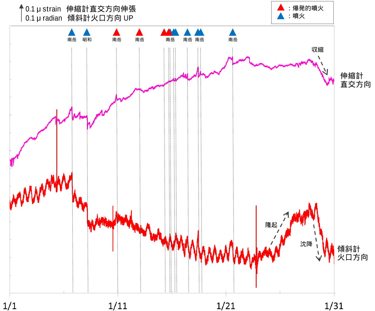
図 6 桜島 有村観測坑道の地殻変動の状況（2018 年 1 月 1 日～ 1 月 31 日）
