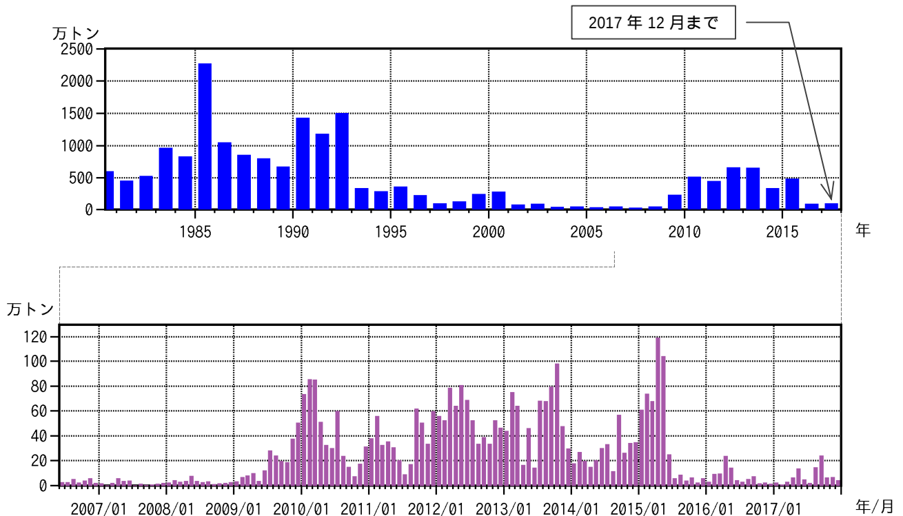
図9 桜島 鹿児島県が実施している降灰の観測データから推定した火山灰の総噴出量 （上段：1980年1月～2017年12月の年別値、下段：2006年6月～2017年12月の月別値）
