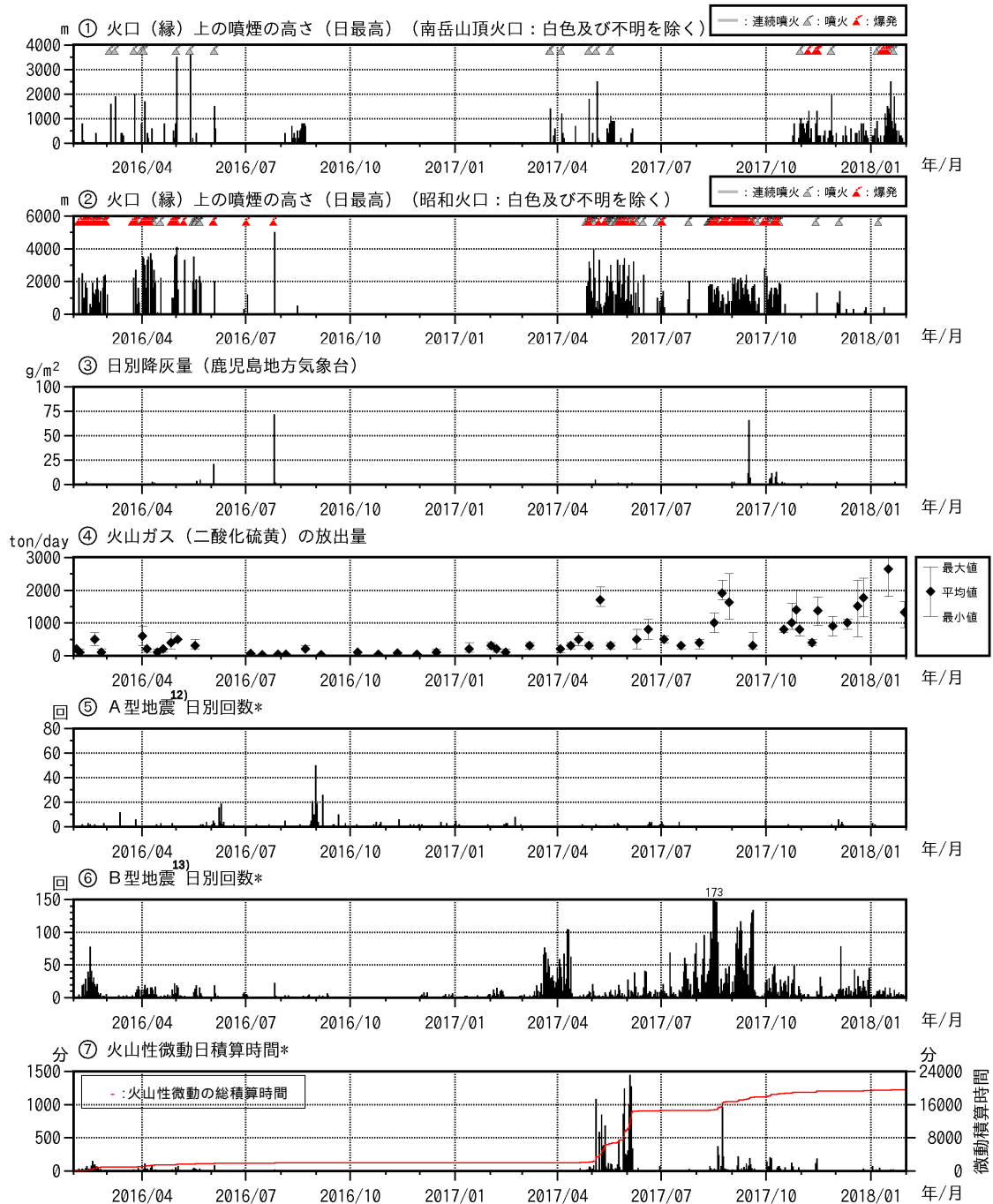
図 3 桜島 最近 2 年間の活動経過図（2016 年 2 月～2018 年 1 月）
