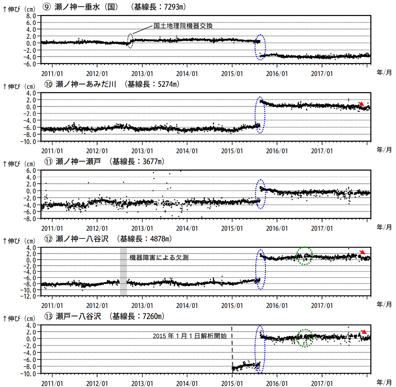
図 7-3 桜島 GNSS 連続観測による基線長変化（2010 年 10 月～2018 年 1 月）
