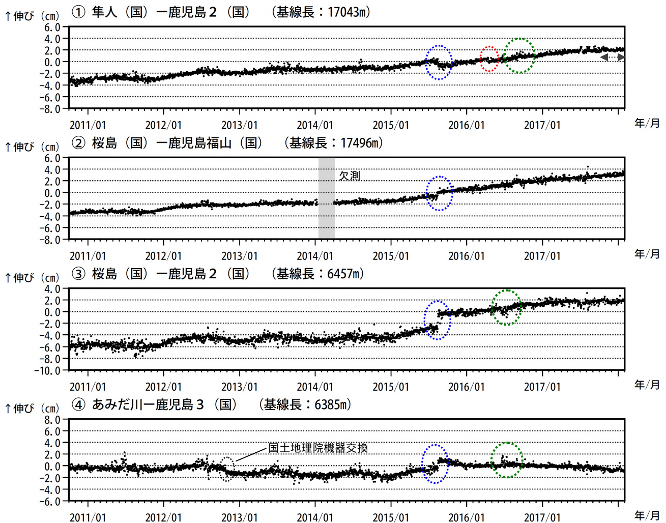
図 7-1 桜島 GNSS 連続観測による基線長変化（2010 年 10 月～2018 年 1 月）
