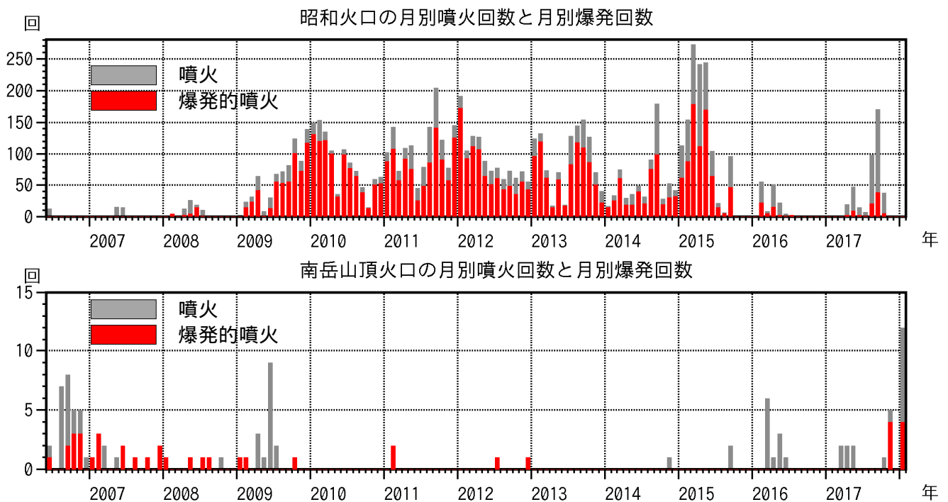
図 2 桜島 昭和火口（上図）と南岳山頂火口（下図）の月別噴火回数と月別爆発回数 （2006 年 6 月～2018 年 1 月）
