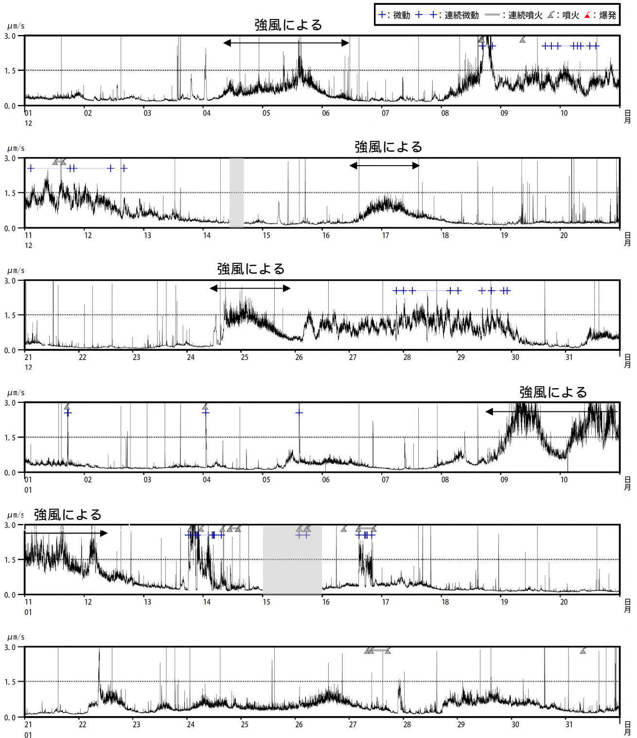
図 4 諏訪之瀬島 1 分間平均振幅の時間変化(トンガマ南西観測点上下動成分、2017 年 12 月～2018 年 1 月)
