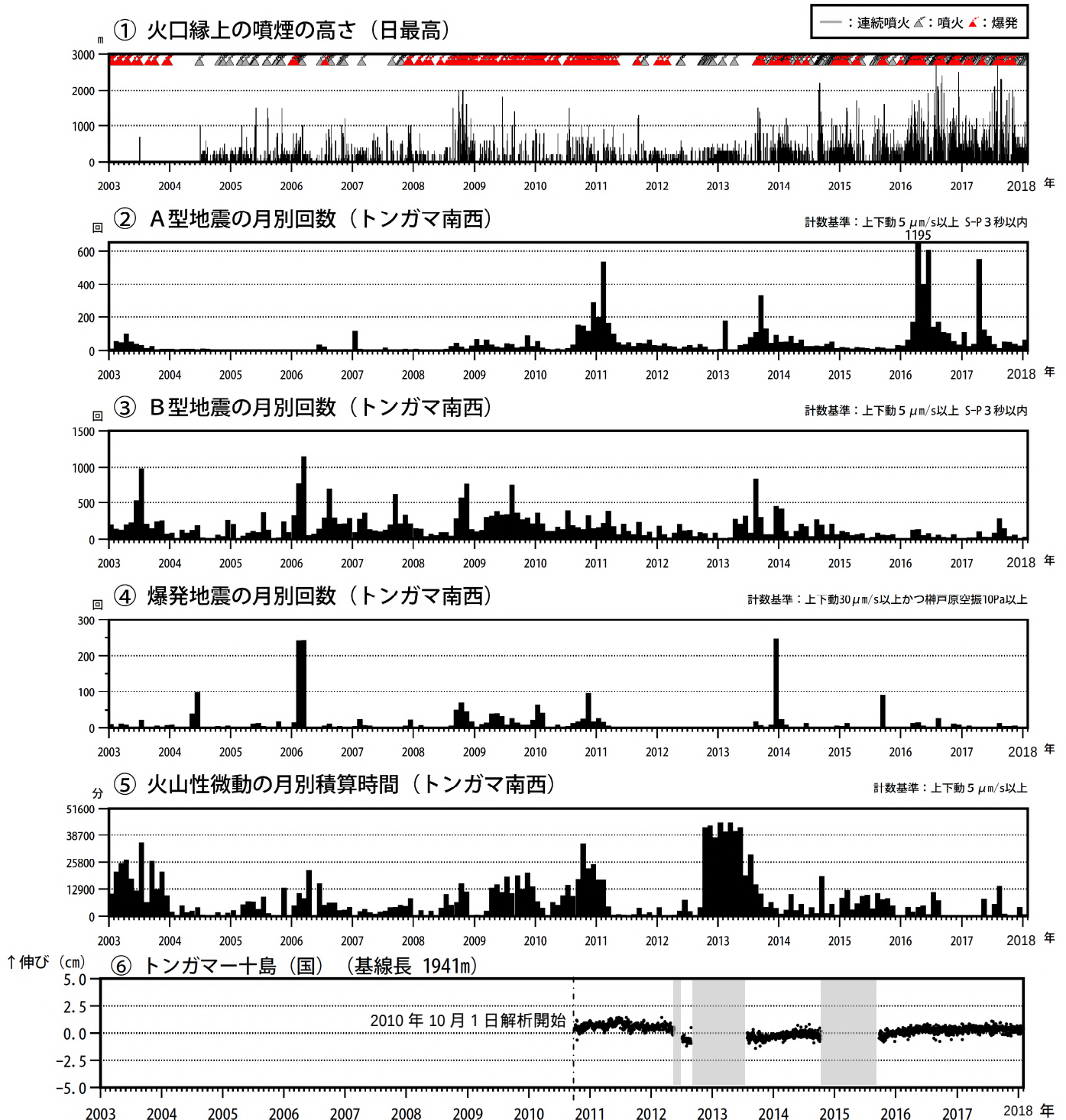
図 2 諏訪之瀬島 長期の火山活動経過図（2003 年 1 月～2018 年 1 月）
