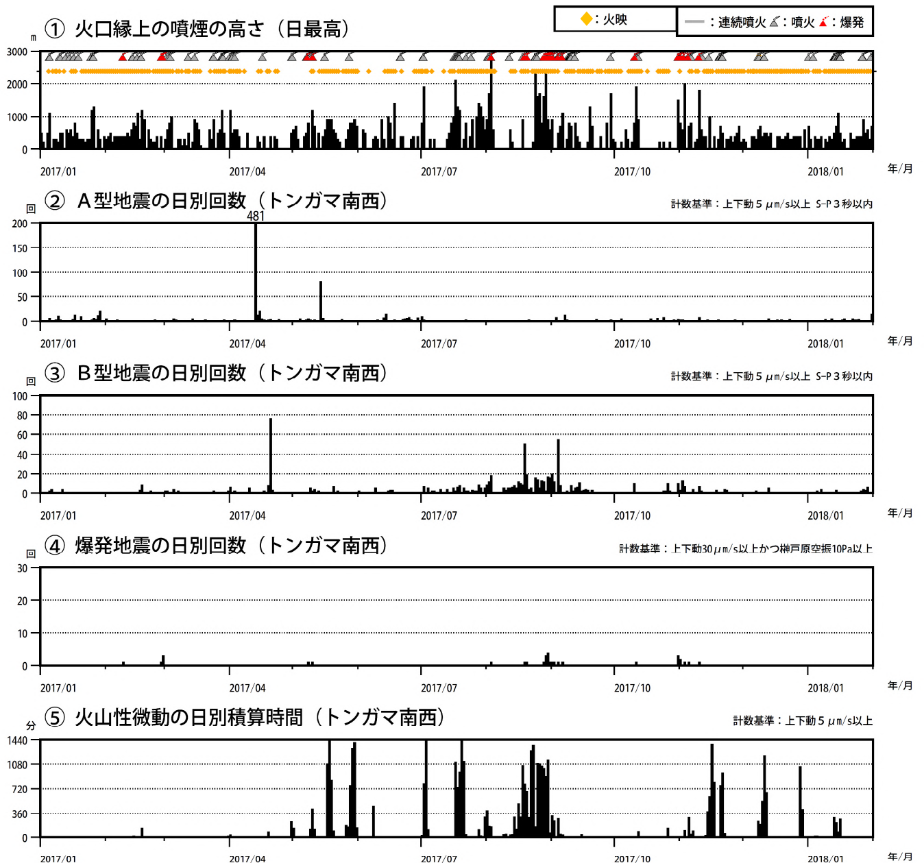
図 3 諏訪之瀬島 最近の火山活動経過図（2017 年 1 月～2018 年 1 月）
