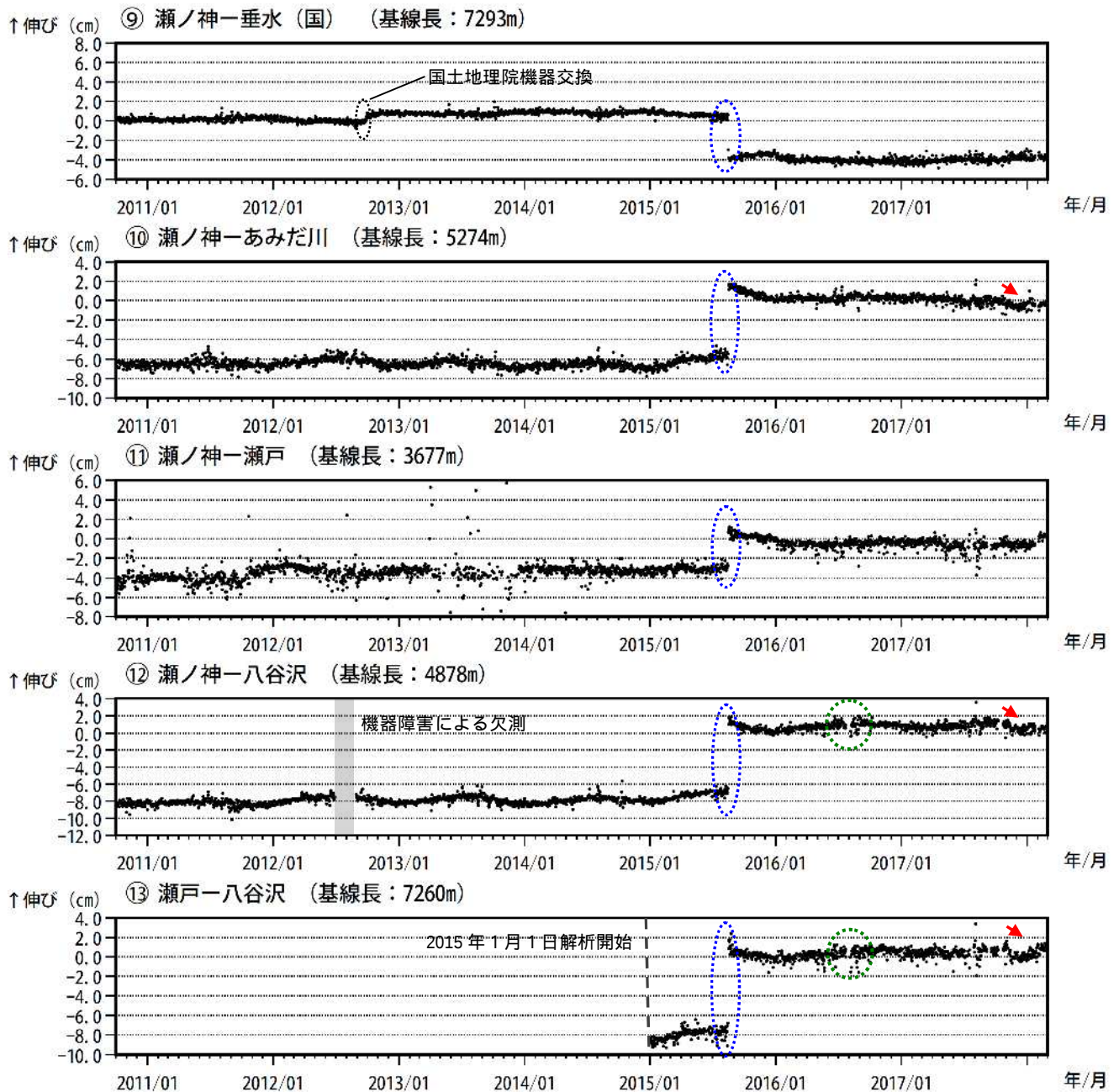
図 7-3 桜島 GNSS 連続観測による基線長変化 (2010 年 10 月 ~ 2018 年 2 月)
