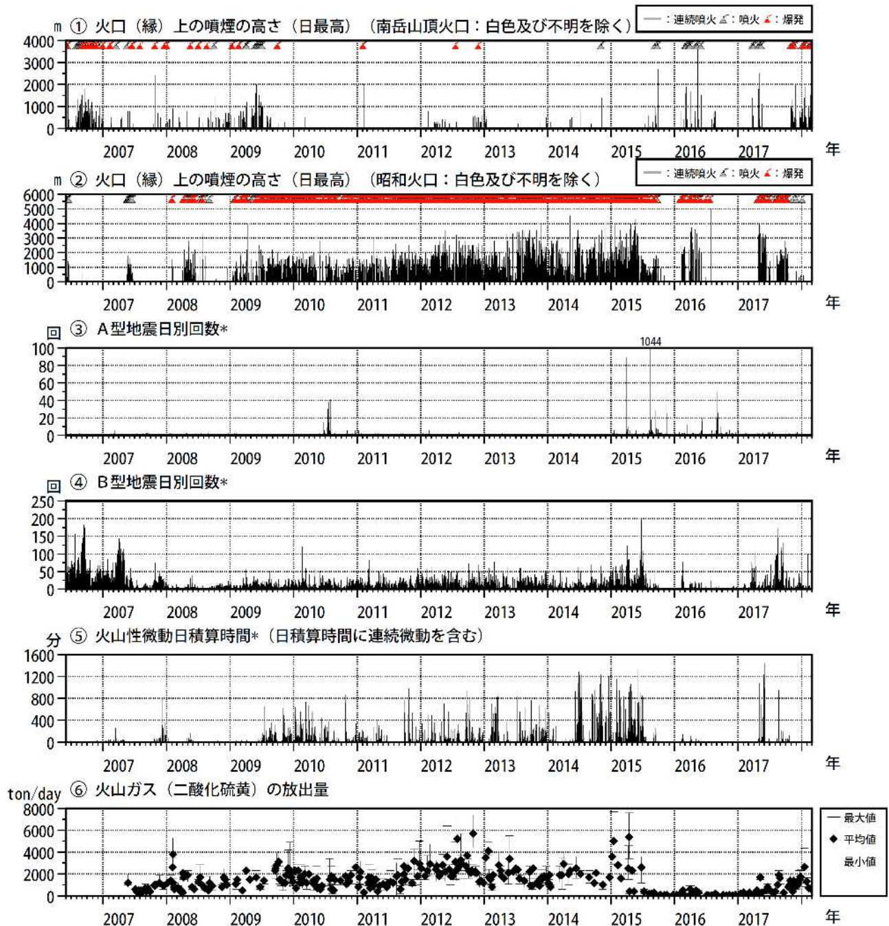
図4 桜島 昭和火口噴火活動再開（2006年6月）以降の活動経過図
