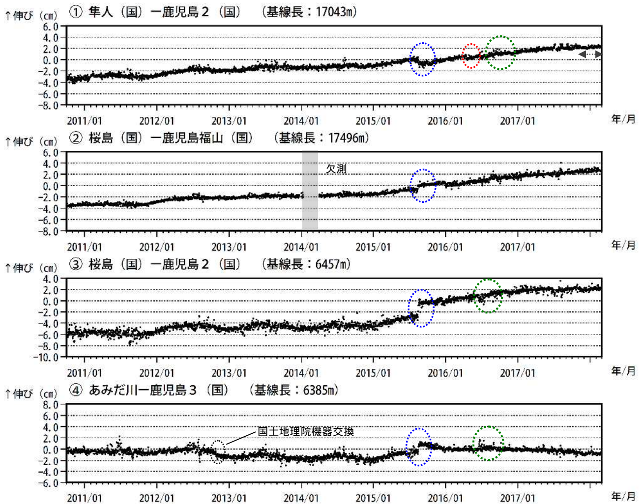
図 7-1 桜島 GNSS 連続観測による基線長変化（2010 年 10 月～2018 年 2 月）
