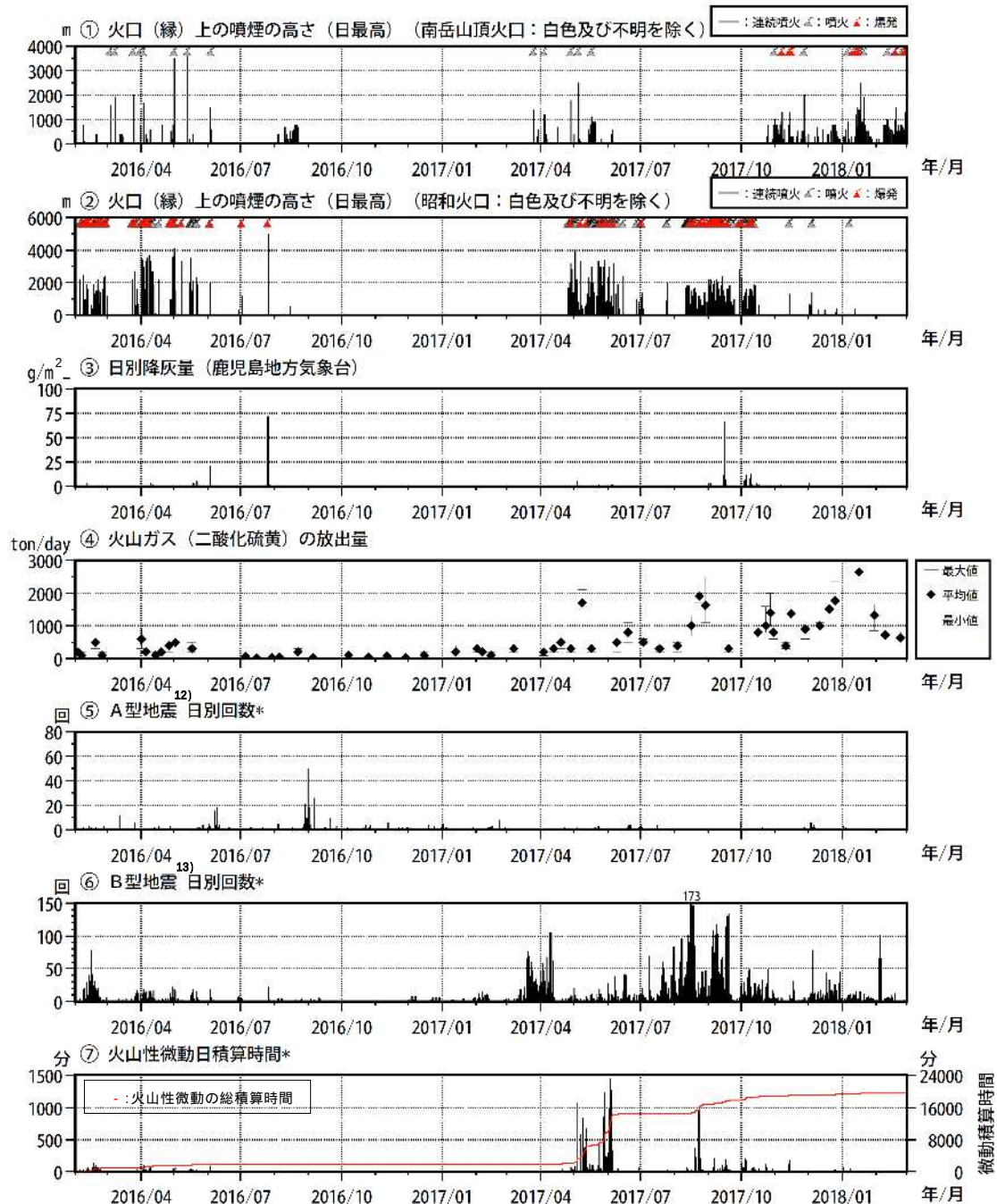
図3 桜島 最近2年間の活動経過図（2016年2月～2018年2月）
