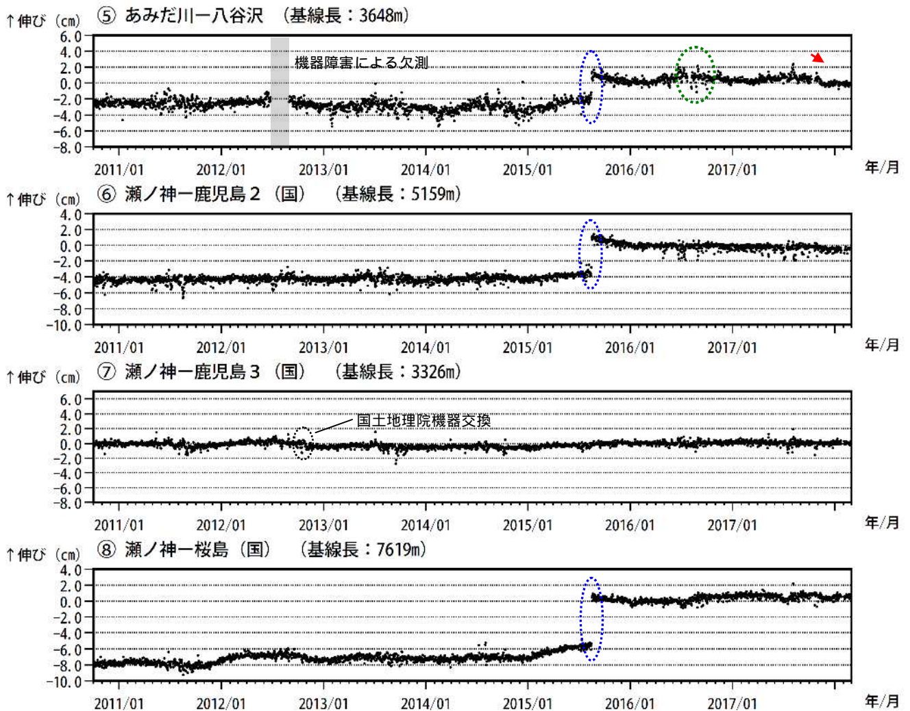
図 7-2 桜島 GNSS 連続観測による基線長変化 (2010 年 10 月 ~ 2018 年 2 月)
