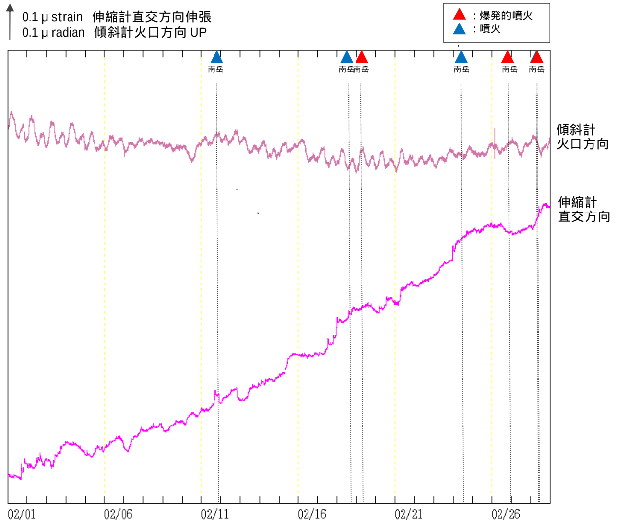
図 6 桜島 有村観測坑道の地殻変動の状況（2018 年 2 月 1 日～2 月 28 日）
