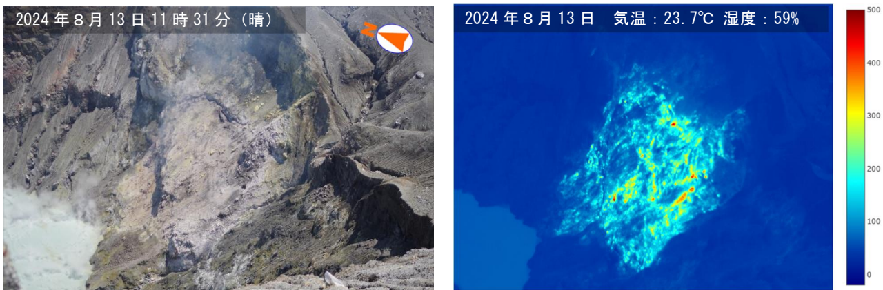
図 2-2 阿蘇山 中岳第一火口 南側火口壁の状況（8月13日、火口南西側観測定点から撮影）
