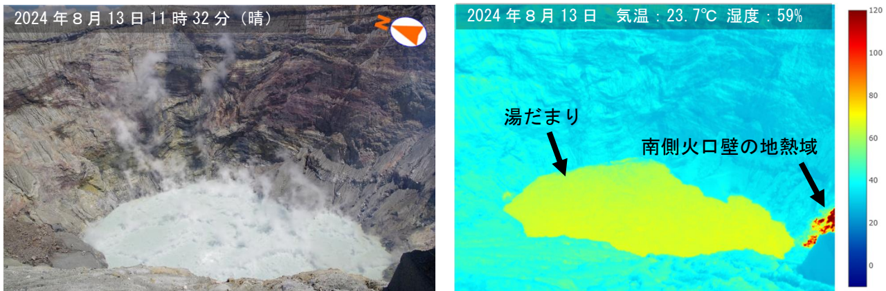
図 2-1 阿蘇山 中岳第一火口底の状況（8月13日、火口南西側観測定点から撮影）
