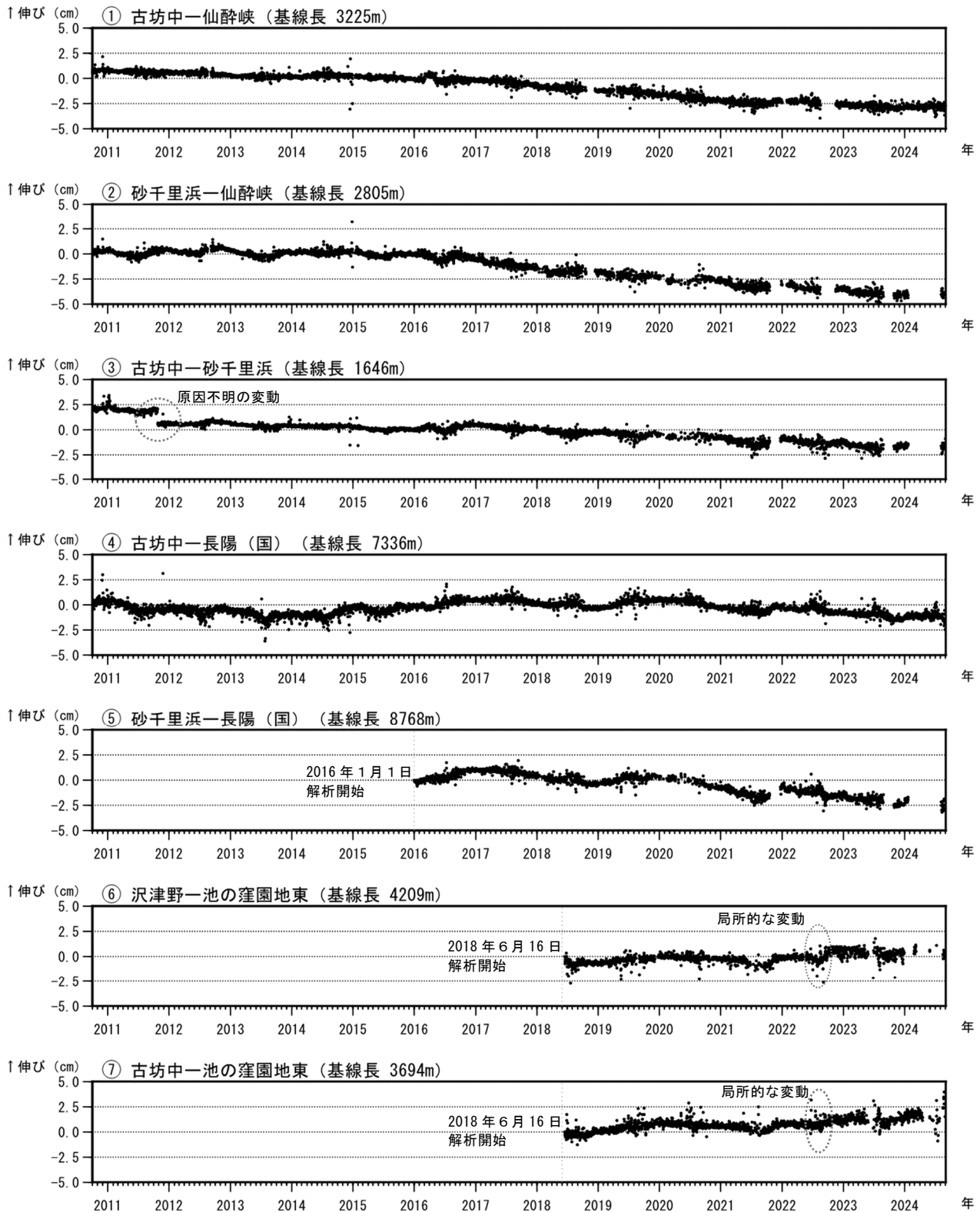
図5 阿蘇山 GNSS 連続観測による基線長変化（2010年10月～2024年8月）
