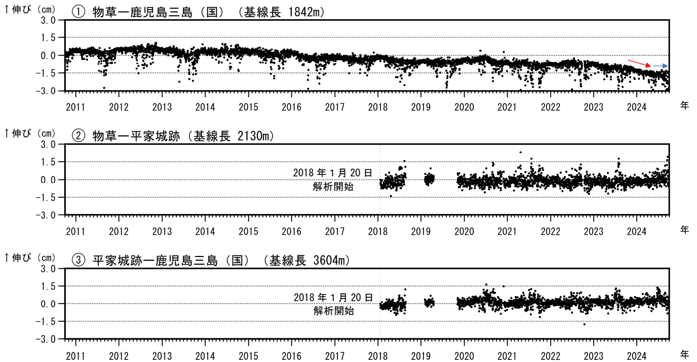
図5 薩摩硫黄島 GNSS連続観測による基線長変化（2010年10月～2024年9月）
