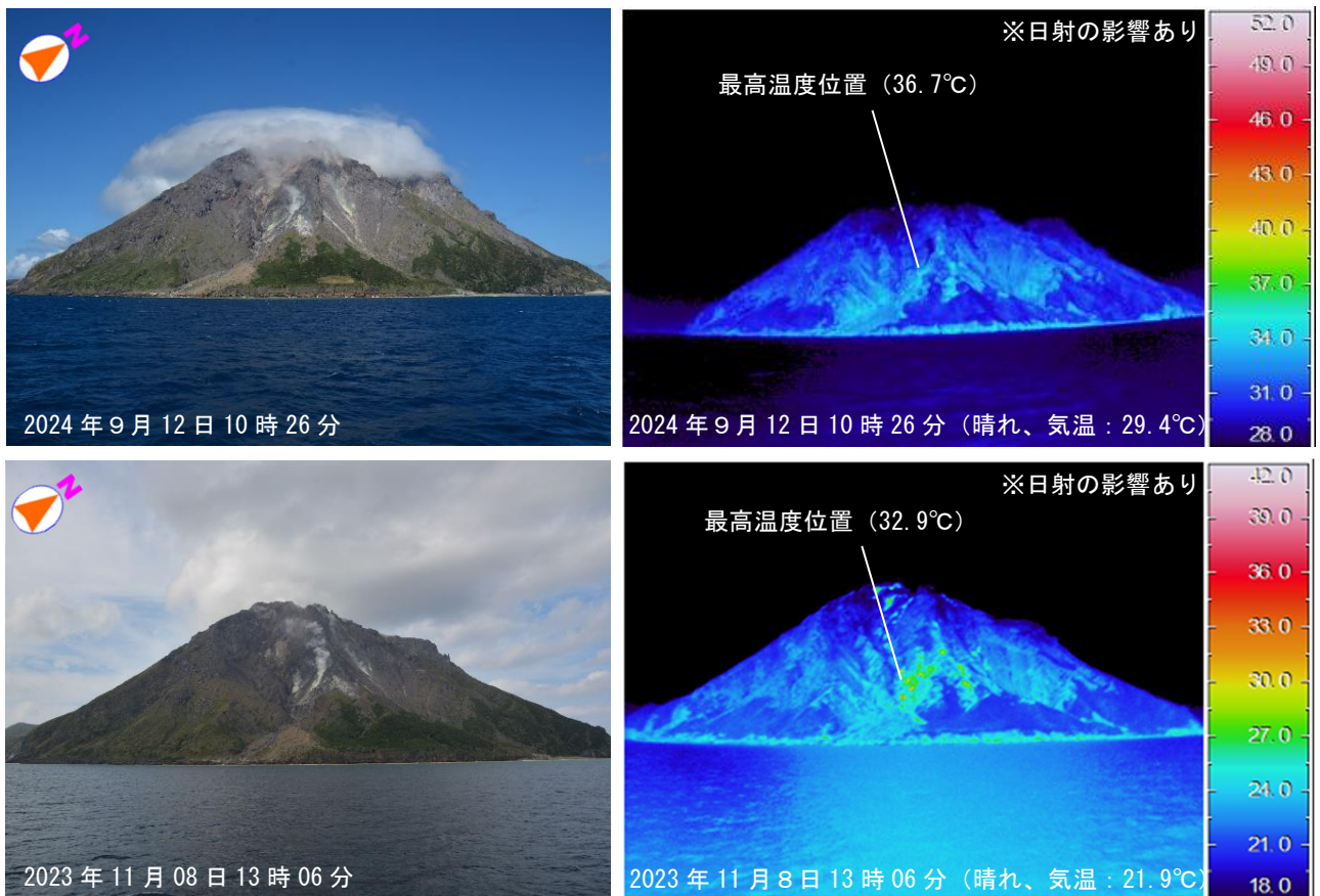
図 2-2 薩摩硫黄島 硫黄岳の状況（薩摩硫黄島の南東海上から観測）
