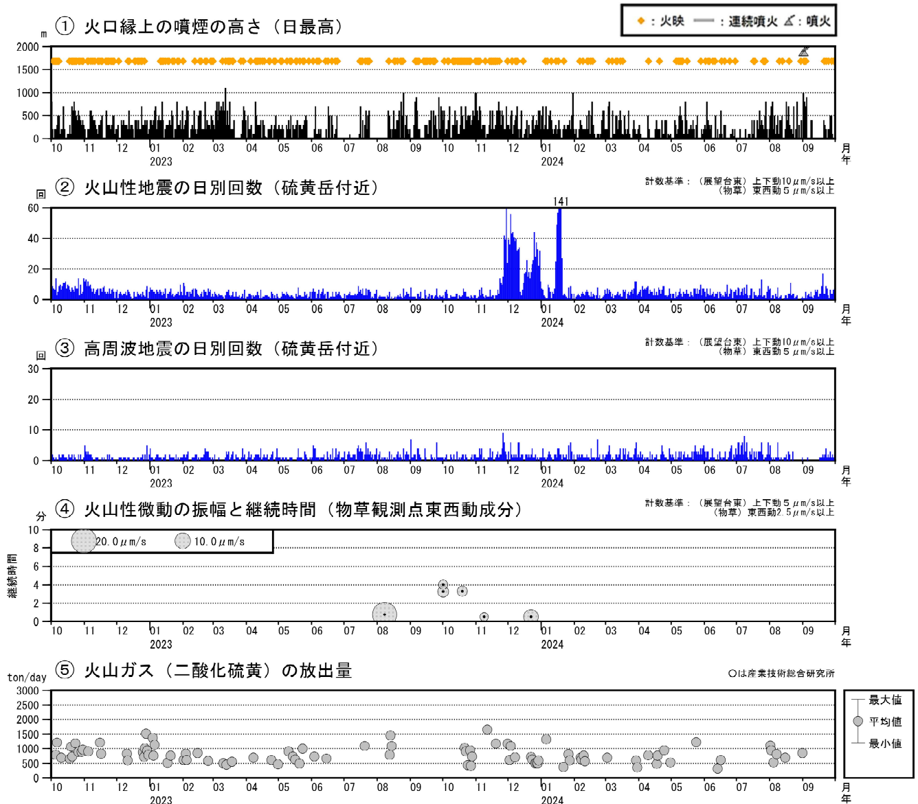
図4 薩摩硫黄島 火山活動経過図（2022年10月～2024年9月）
