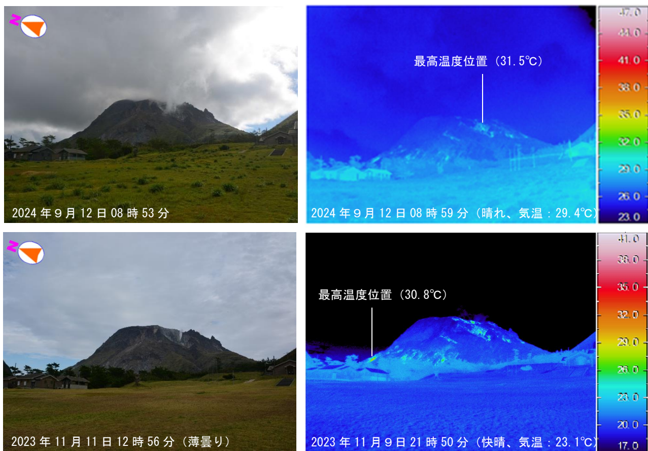
図 2-3 薩摩硫黄島 硫黄岳の状況（冒険ランドいおうじまから観測）
