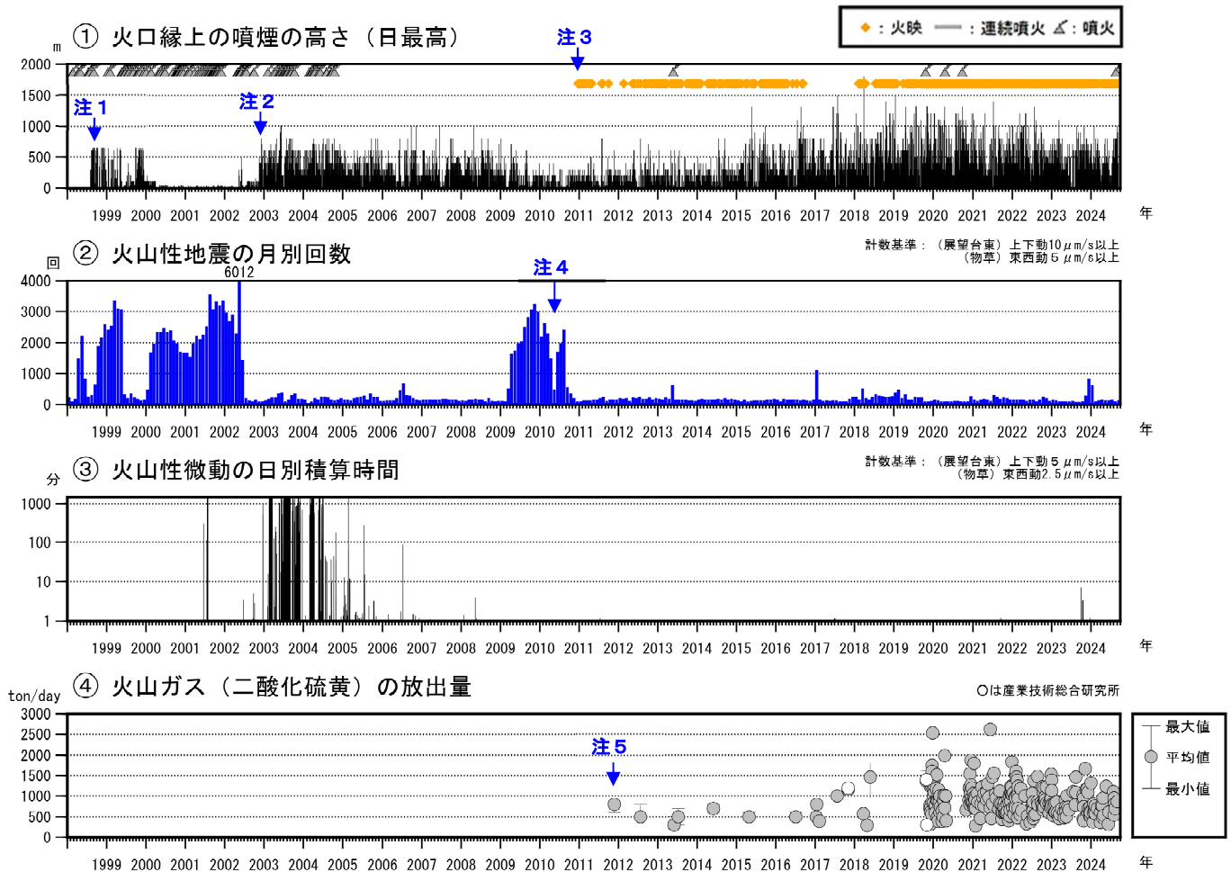
図3 薩摩硫黄島 火山活動経過図（1998年1月～2024年9月）
