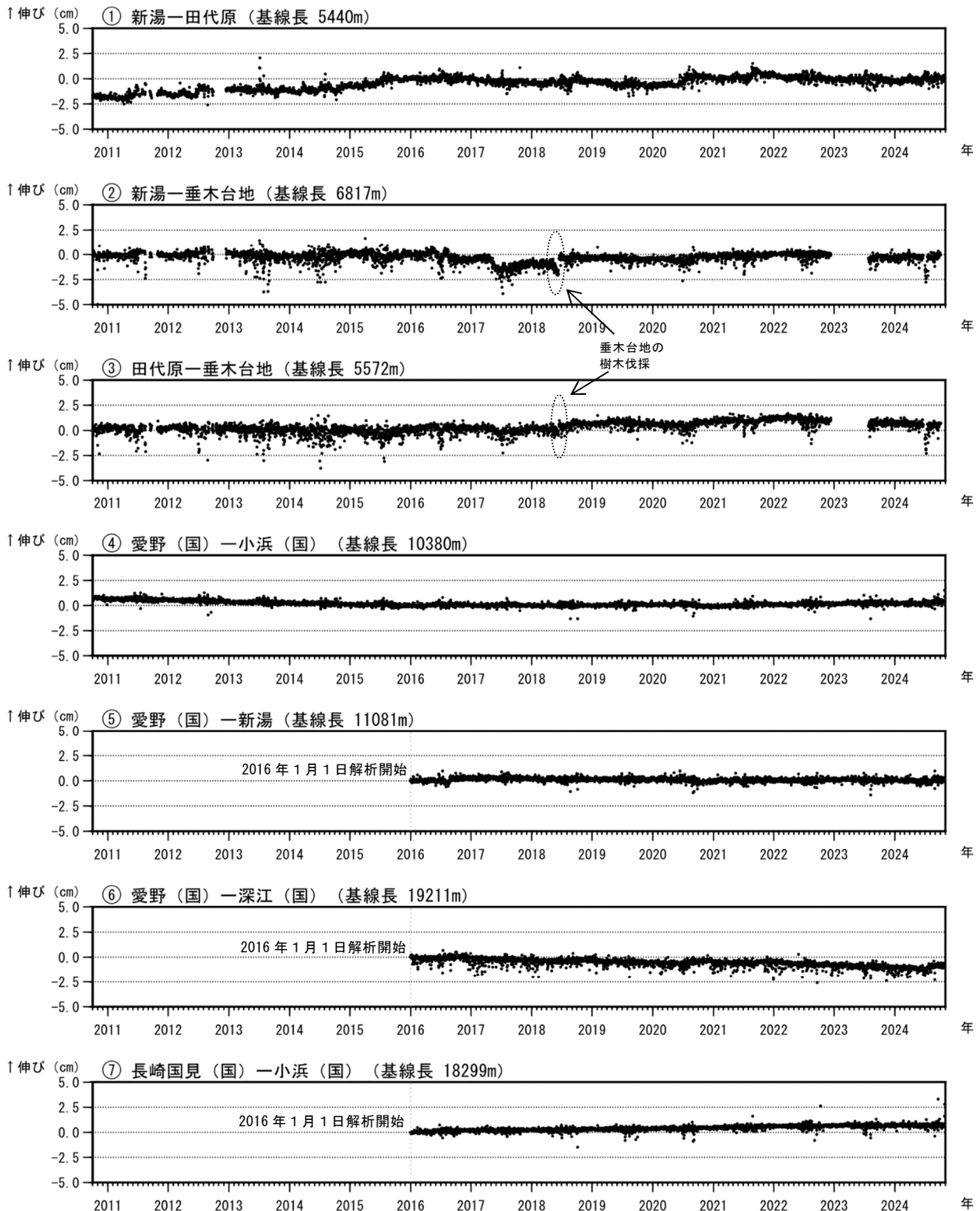
図5 雲仙岳 GNSS連続観測による基線長変化（2010年10月～2024年10月）
