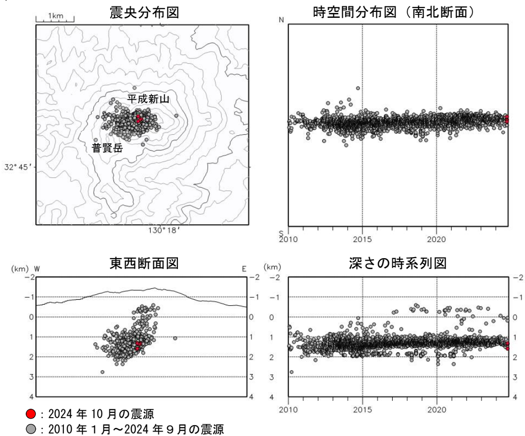
図4 雲仙岳 震源分布図 ①広域図 ②狭域図（2010年1月～2024年10月）
