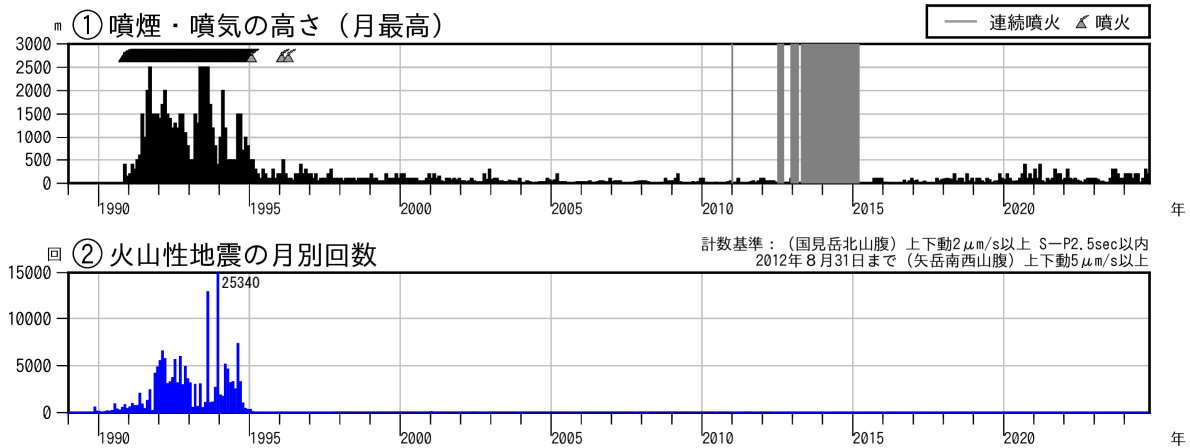
図2 雲仙岳 長期の火山活動経過図（1989年1月～2024年10月）
