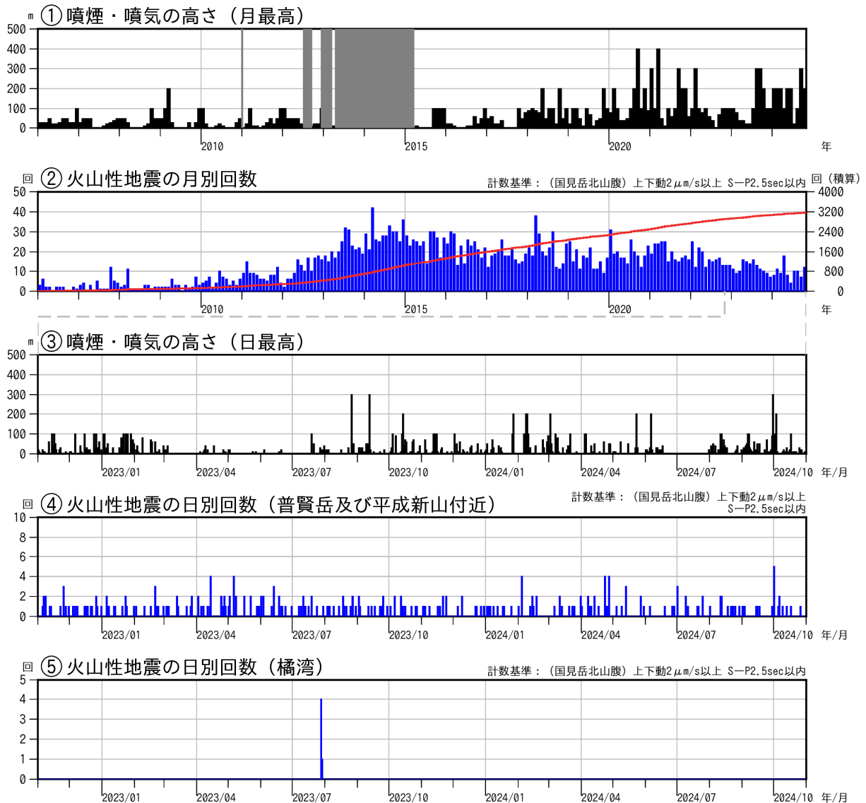
図3 雲仙岳 火山活動経過図（2006年1月～2024年10月）
