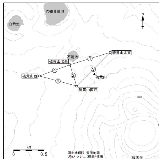
図3 霧島山（えびの高原（硫黄山）周辺） 図2及び図5のGNSS連続観測点と基線番号 白丸（○）は気象庁の観測点位置を示しています。
