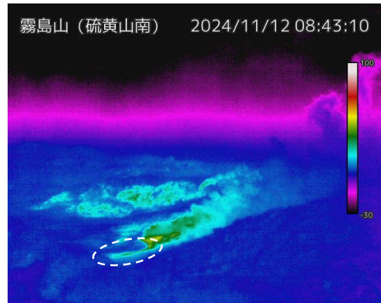
図 1-2 霧島山（えびの高原（硫黄山）周辺） 硫黄山南側の状況 （11月12日、硫黄山南監視カメラ）
