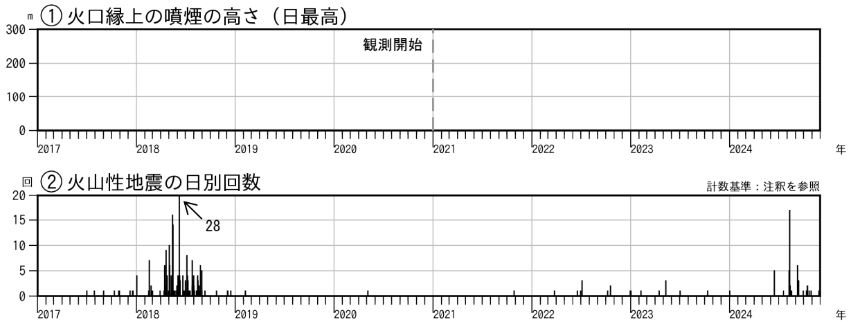
図2 霧島山（大幡池） 火山活動経過図（2017年1月～2024年11月）
