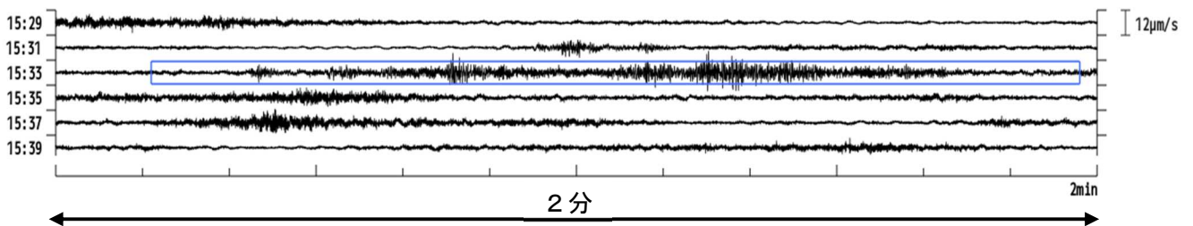
図5 霧島山（新燃岳） 15日15時33分に発生した火山性微動の状況 (新燃西(震)地震計：速度波形南北動成分)
