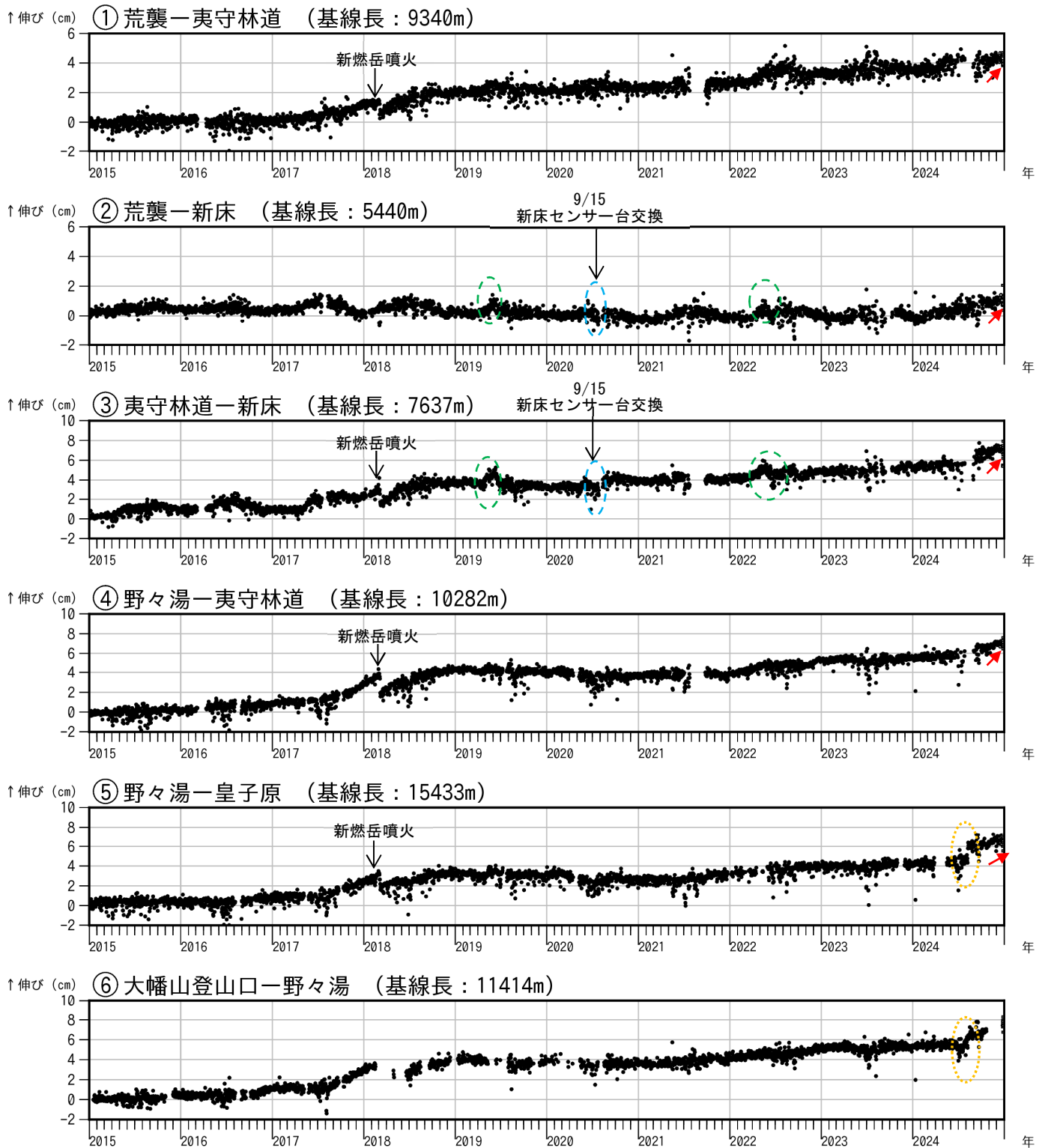
図8 霧島山（新燃岳） GNSS 連続観測による基線長変化（2015年1月～2024年12月）
