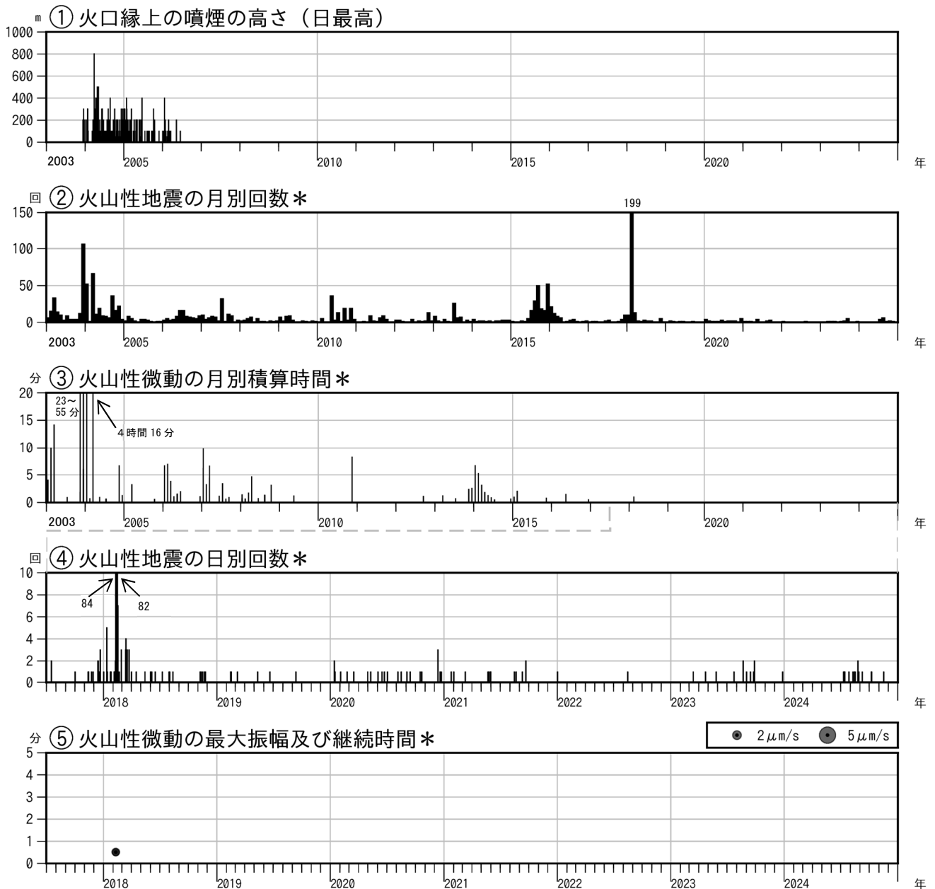
図3 霧島山（御鉢） 火山活動経過図（2003年1月～2024年12月）
