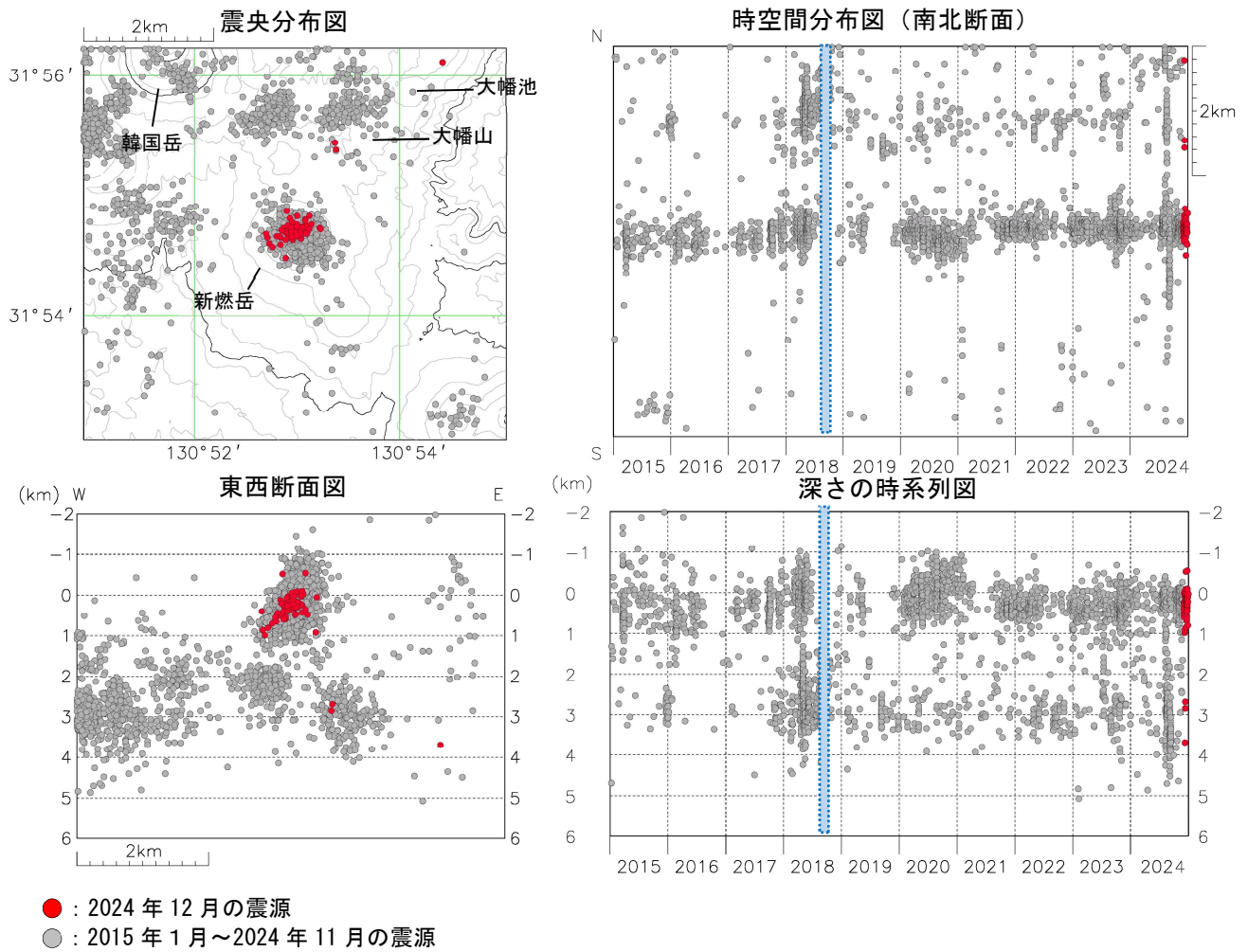
図7 霧島山（新燃岳） 震源分布図（2015 年 1 月～2024 年 12 月）
