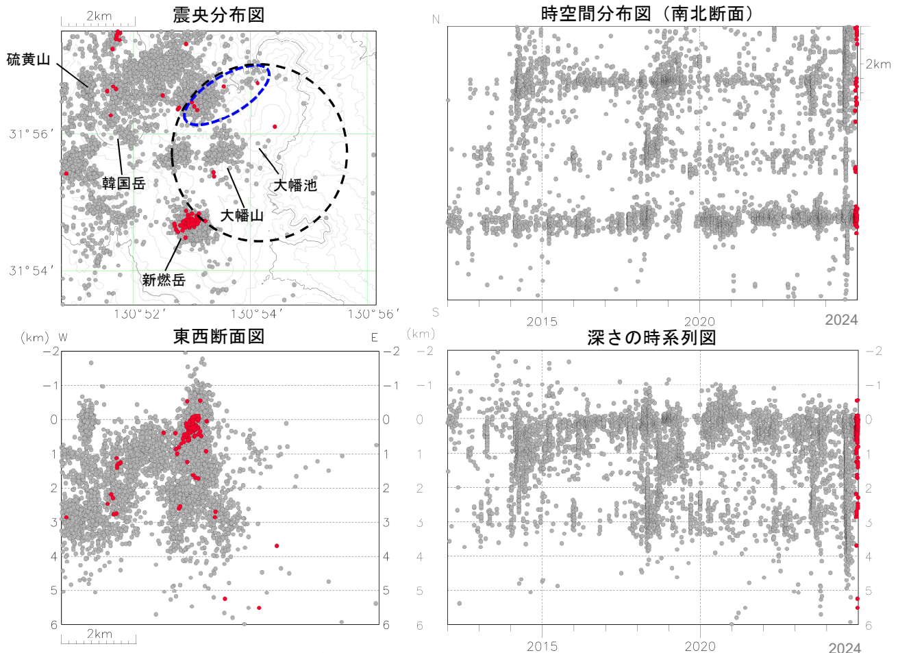
図3 霧島山（大幡池） 震源分布図（2012年1月～2024年12月） ●：2024年12月の震源 ●：2012年1月～2024年11月の震源
