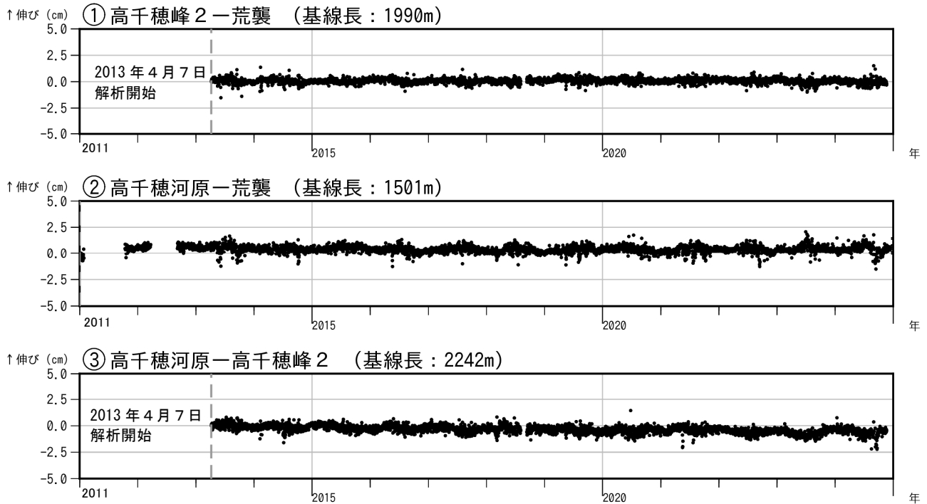
図4 霧島山（御鉢） GNSS 連続観測による基線長変化（2011年1月～2024年12月）
