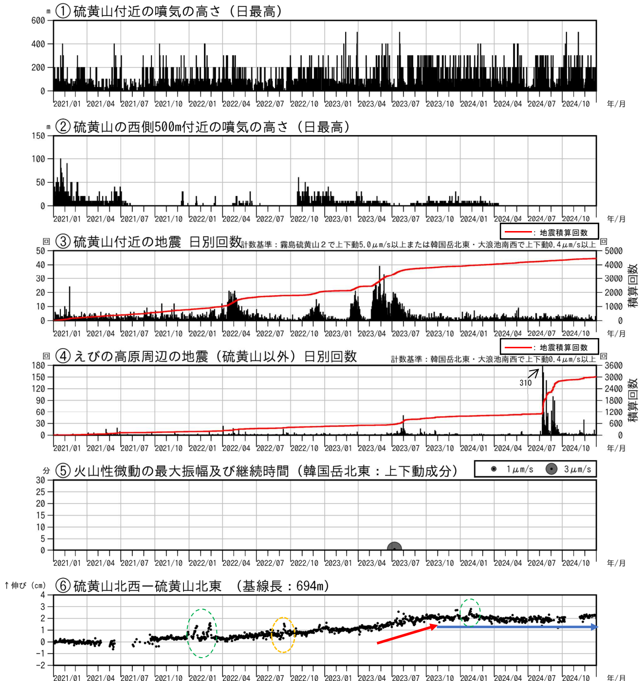
図2 霧島山（えびの高原（硫黄山）周辺） 火山活動経過図（2021年1月～2024年12月）
