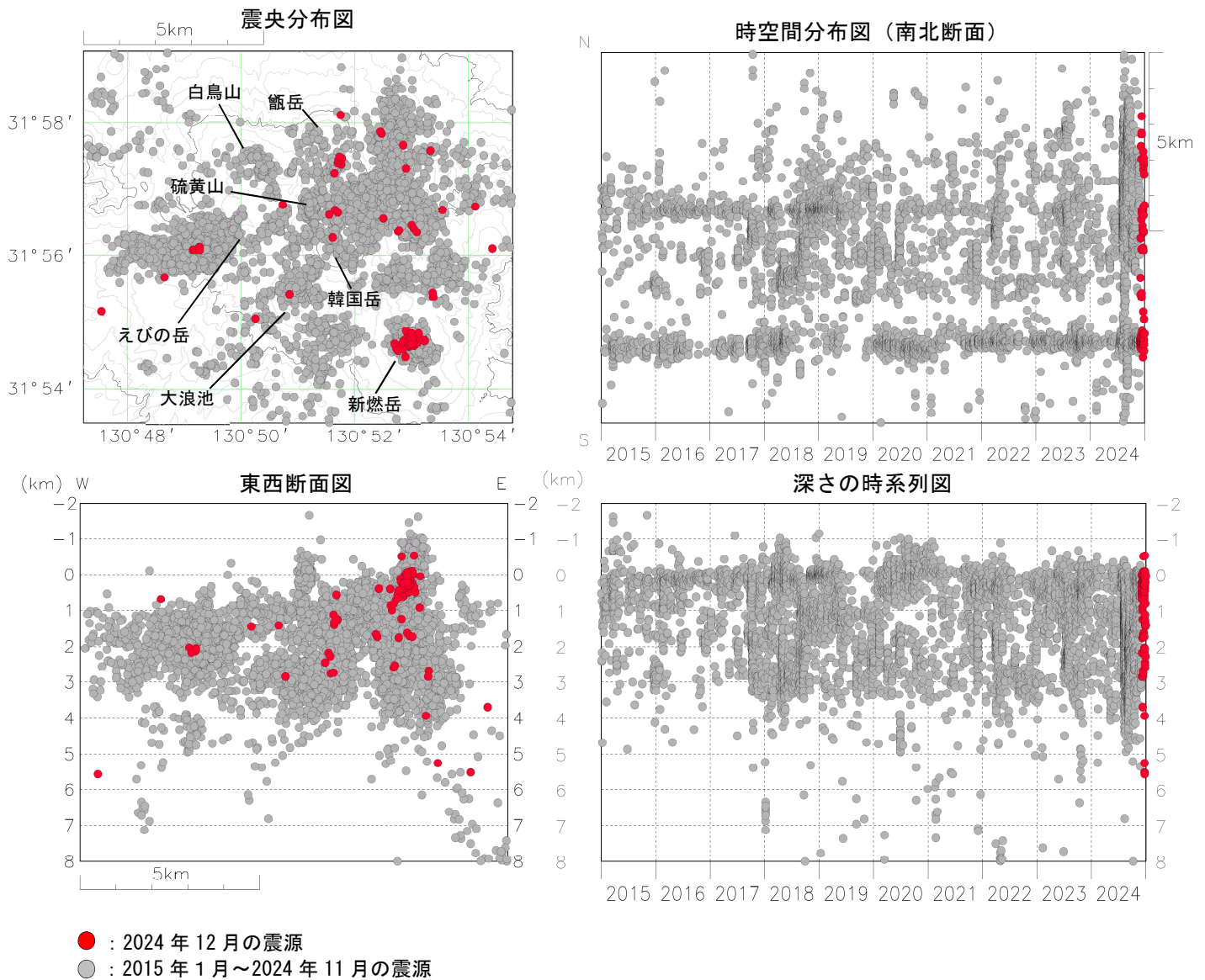
図3 霧島山（えびの高原（硫黄山）周辺） 震源分布図（2015 年 1 月～2024 年 12 月）
