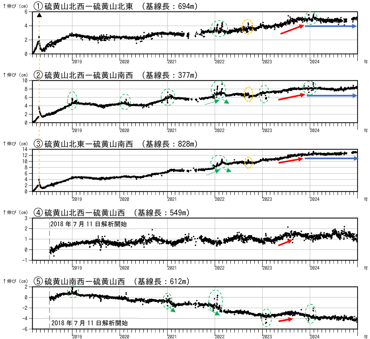
図4 霧島山（えびの高原（硫黄山）周辺） GNSS 連続観測による基線長変化（2018年3月～2024年12月）
