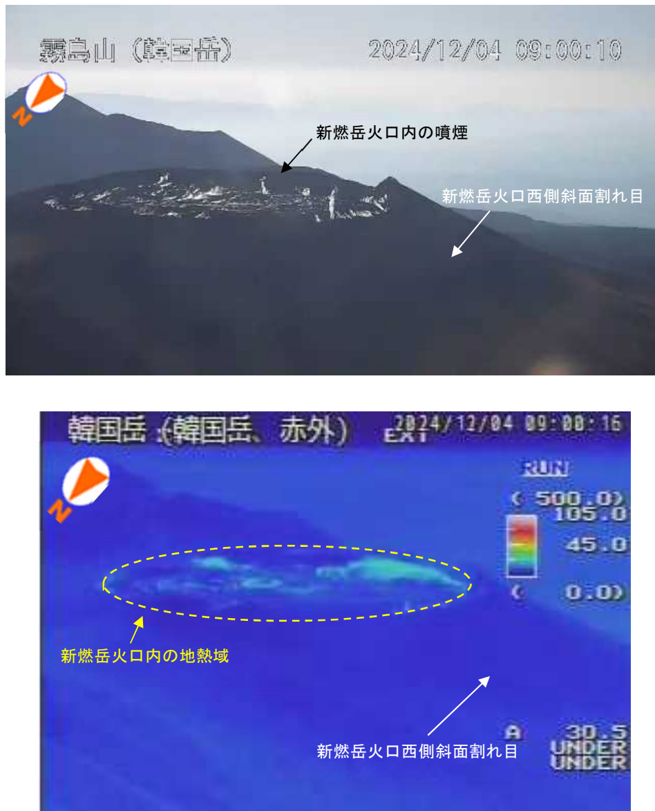
図1 霧島山（新燃岳） 噴煙及び地熱域の状況（12月4日、韓国岳監視カメラ）
