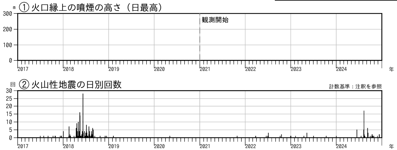
図2 霧島山（大幡池） 火山活動経過図（2017年1月～2024年12月）
