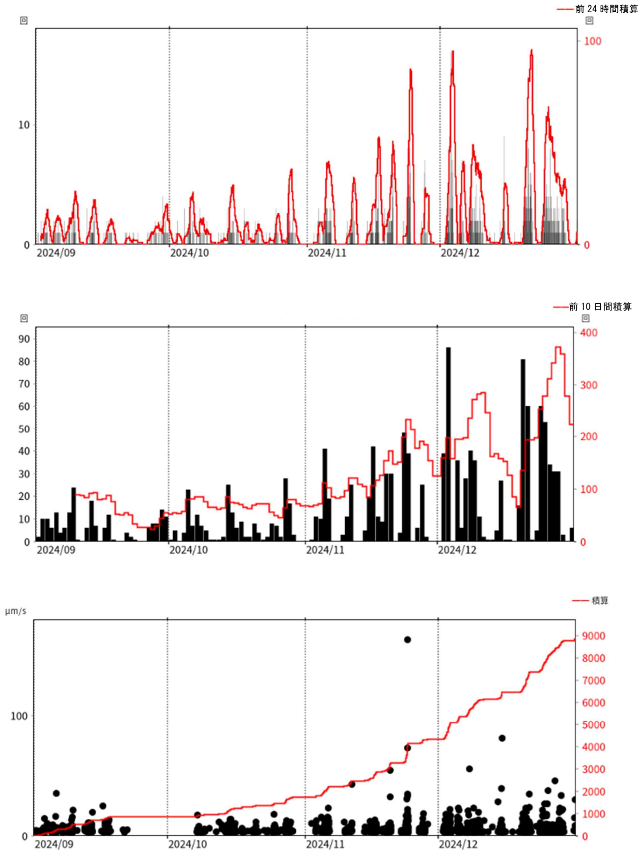
図2 霧島山（新燃岳） 火山性地震の発生状況（2024年9月1日～12月31日） （上段：特別回数、中段：日別回数、下段：火山性地震の最大振幅（新燃西（震）観測点南北動成分）） 新燃岳では、10月下旬頃から火口直下を震源とする振幅の小さな火山性地震が増減を繰り返しながら発生しています。
