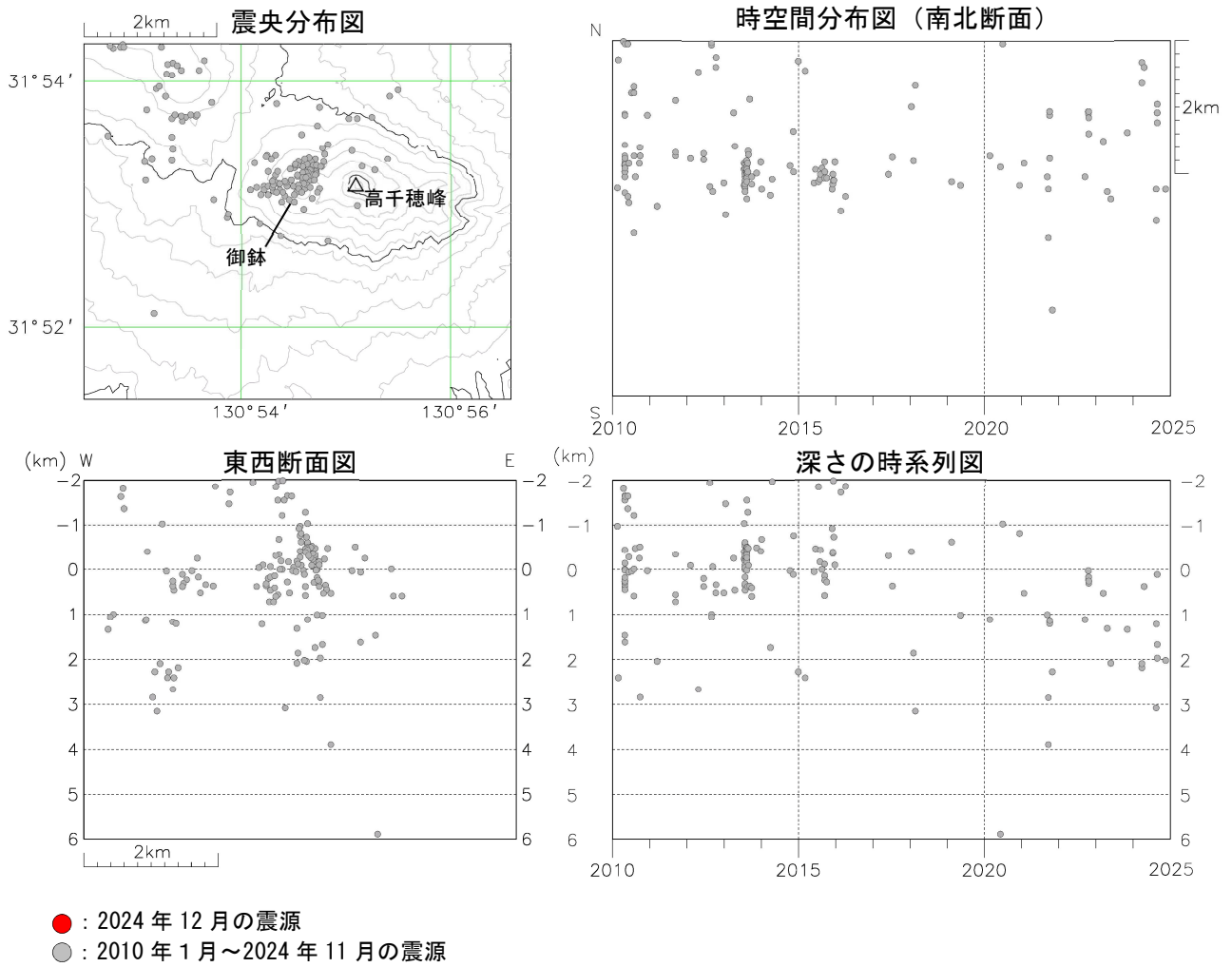
図2 霧島山（御鉢） 震源分布図（2010年1月～2024年12月）
