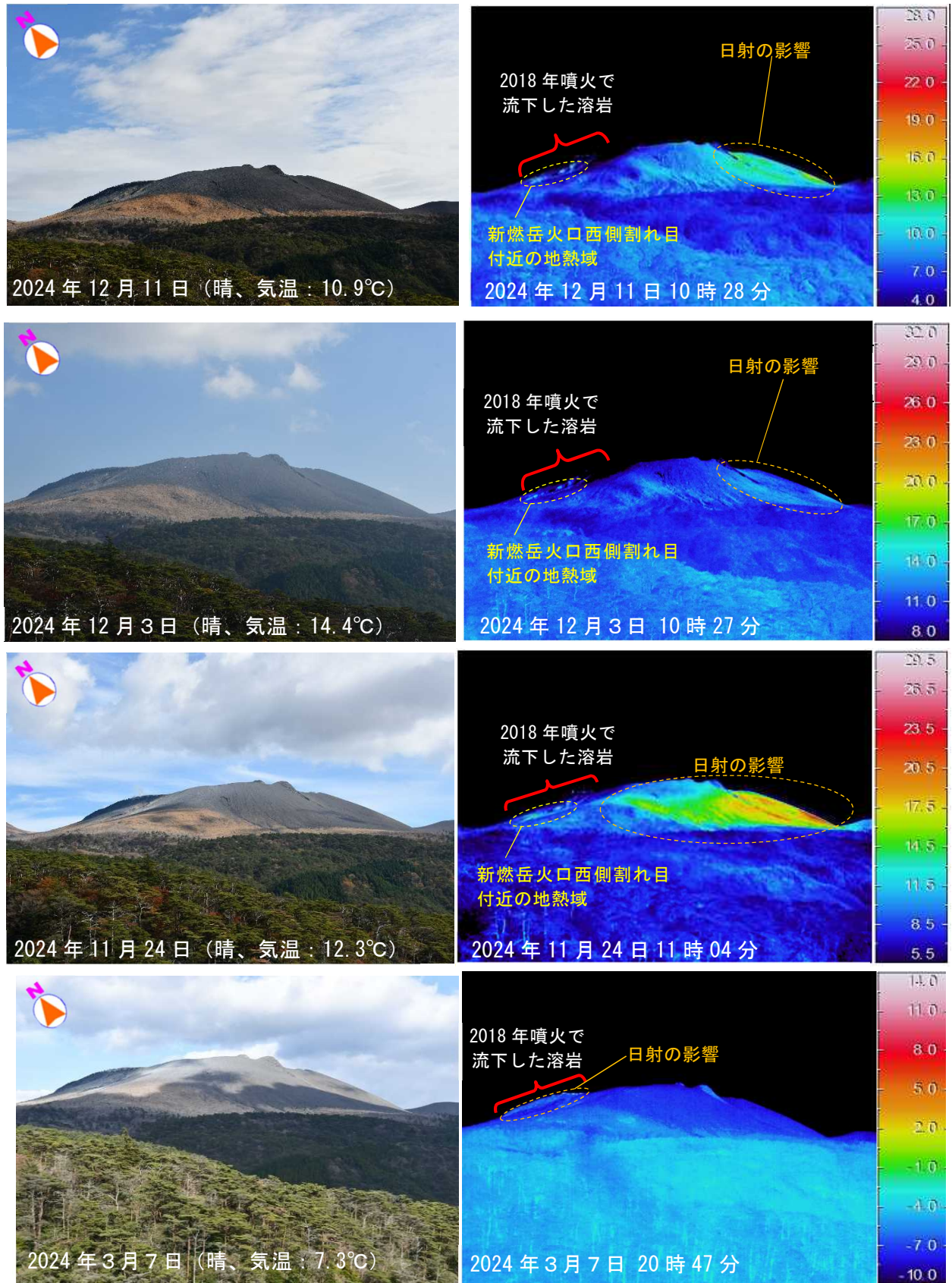
図3 霧島山（新燃岳） 新燃岳南西側の状況（新湯温泉付近からの観測）
