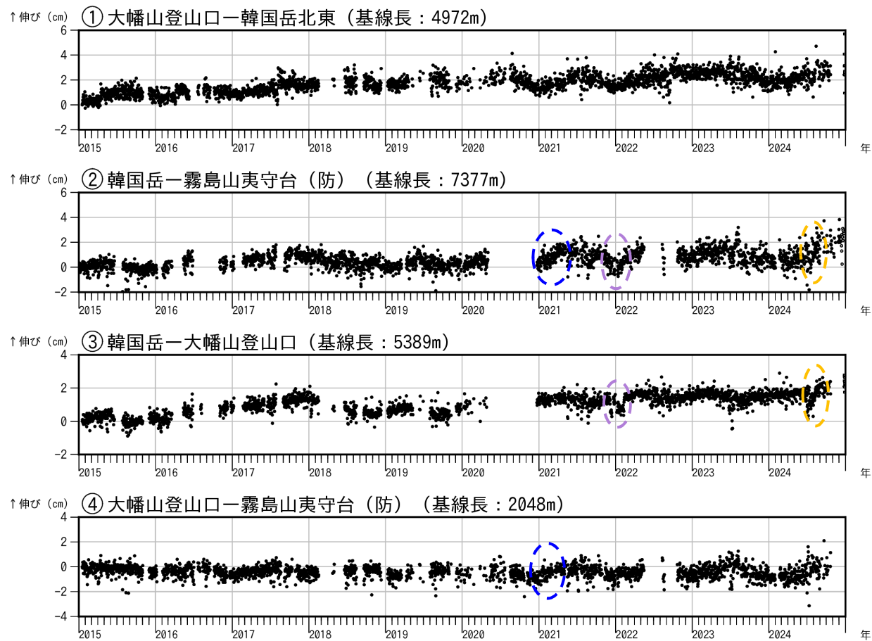
図4 霧島山（大幡池） GNSS 連続観測による基線長変化（2015年1月～2024年12月）
