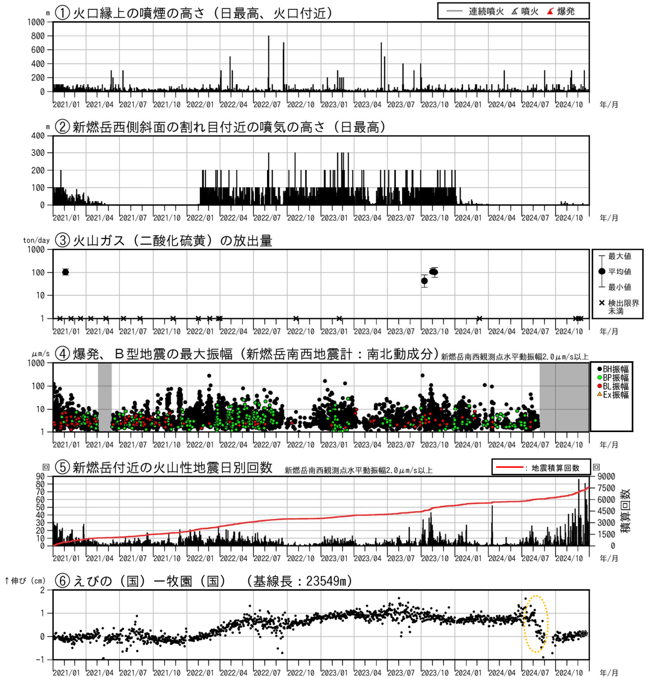
図6 霧島山（新燃岳） 火山活動経過図（2021年1月～2024年12月31日）
