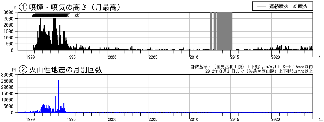
図2 雲仙岳 長期の火山活動経過図（1989年1月～2025年1月）
