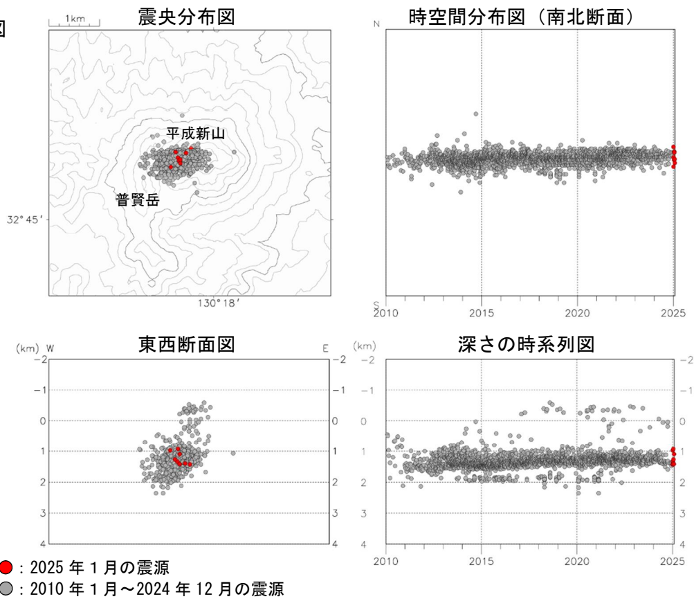
図4 雲仙岳 震源分布図 ①広域図 ②狭域図（2010年1月～2025年1月）
