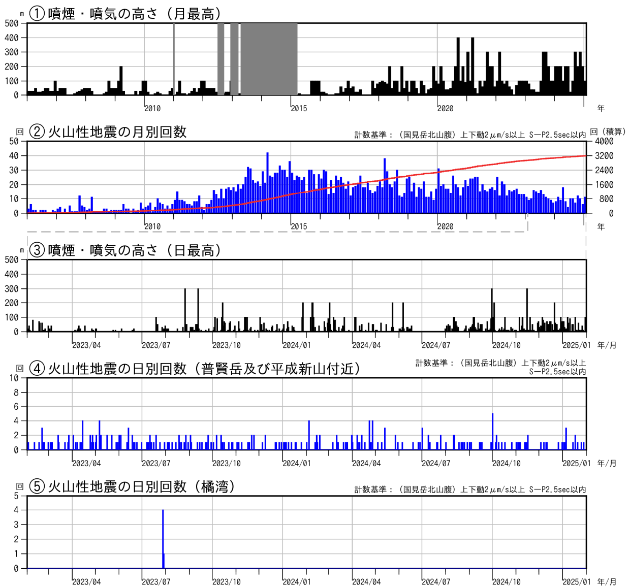
図3 雲仙岳 火山活動経過図（2006年1月～2025年1月）
