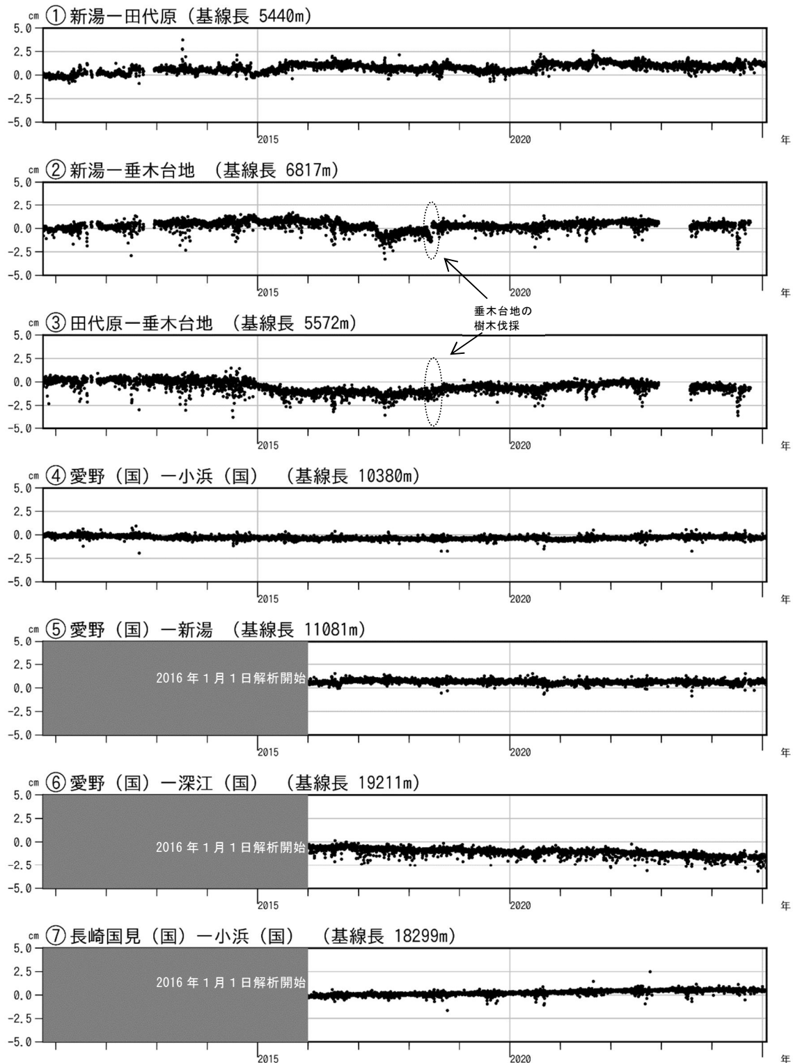
図5 雲仙岳 GNSS連続観測による基線長変化（2010年10月～2025年1月）
