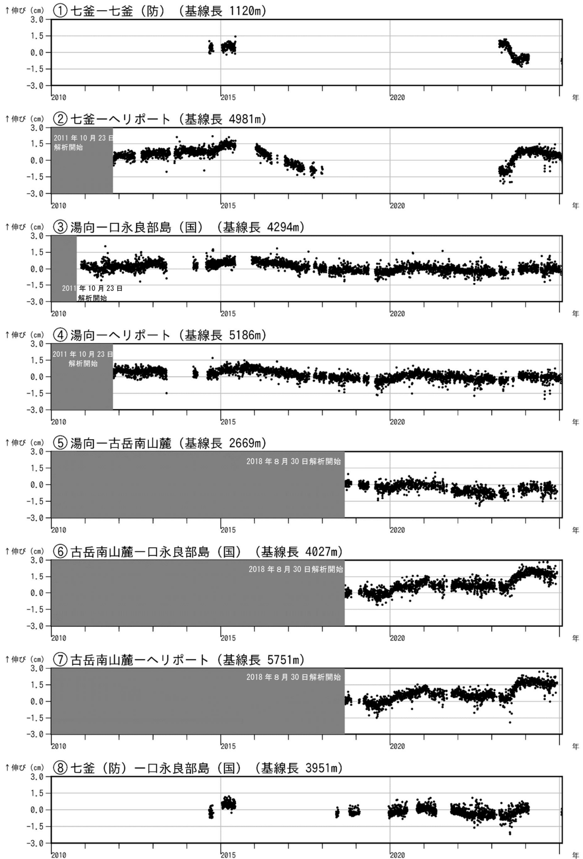
図 6-2 口永良部島 GNSS 連続観測による基線長変化（2010 年 1 月～2025 年 1 月）
