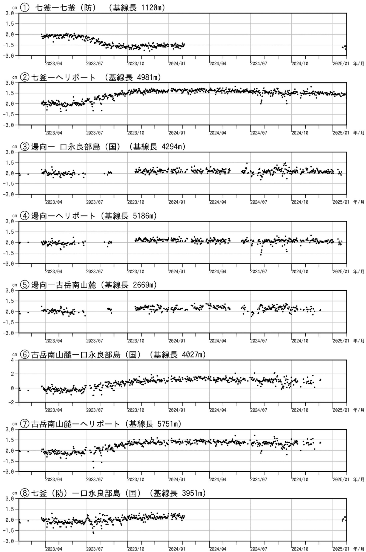
図 6-1 口永良部島 GNSS 連続観測による基線長変化（2023 年 2 月～2025 年 1 月）
