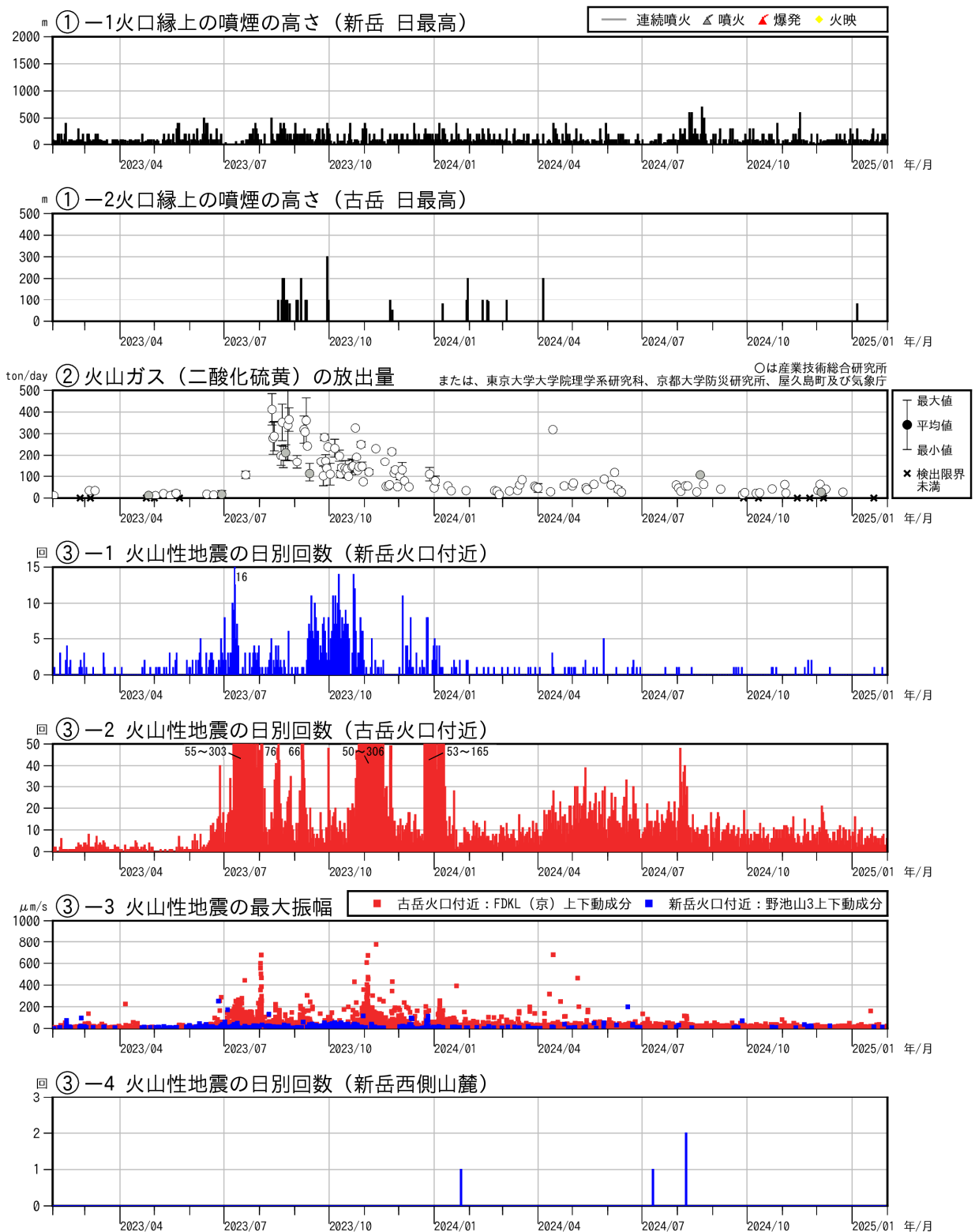
図 4-2 ロ永良部島 最近の火山活動経過図（2023 年 2 月～2025 年 1 月）
