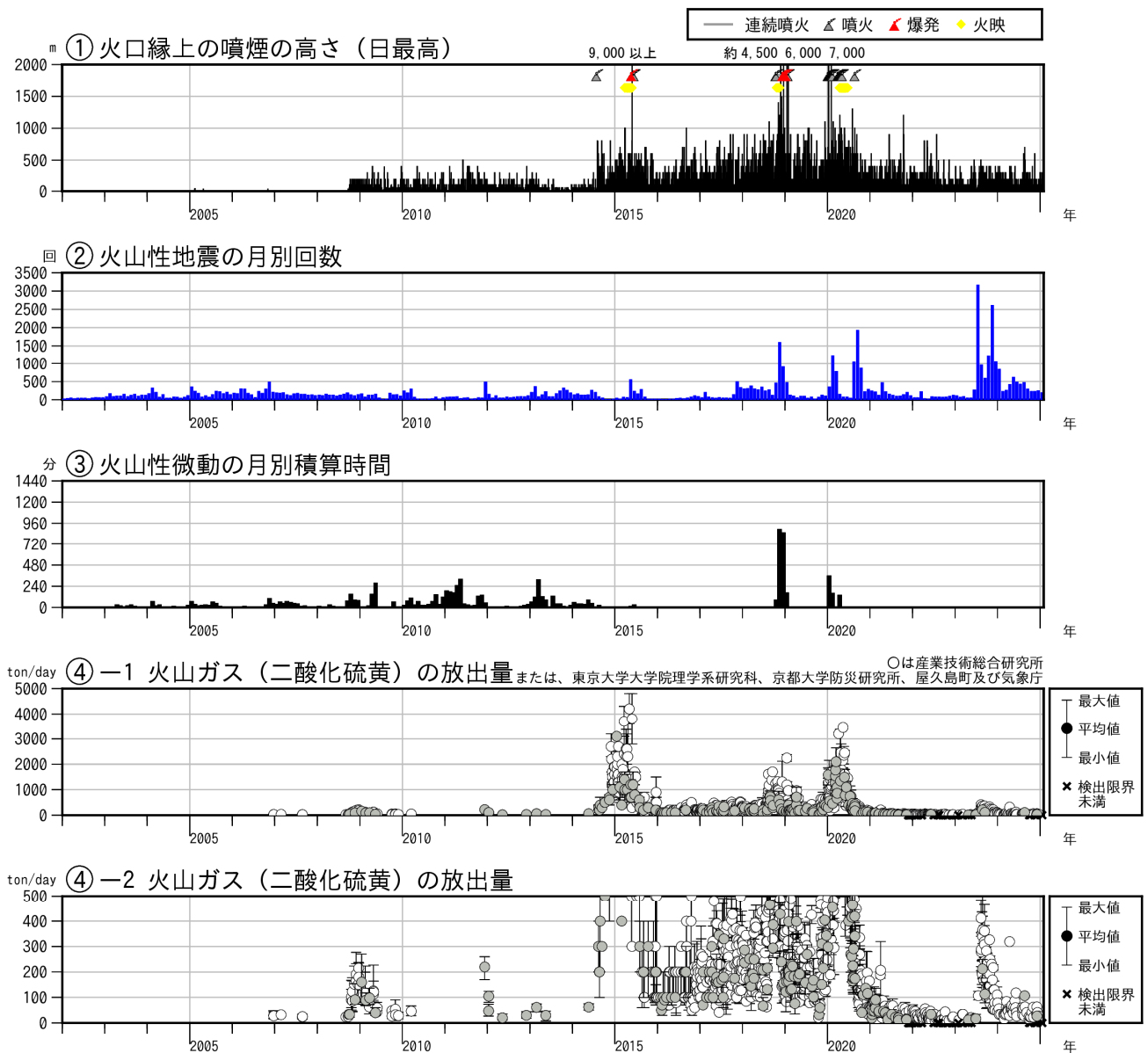
図 4-1 口永良部島 火山活動経過図（2002 年 1 月～2025 年 1 月）
