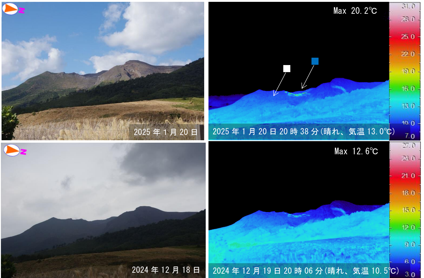
図 3-1 口永良部島 古岳周辺の地熱域の状況（湯向から観測）
