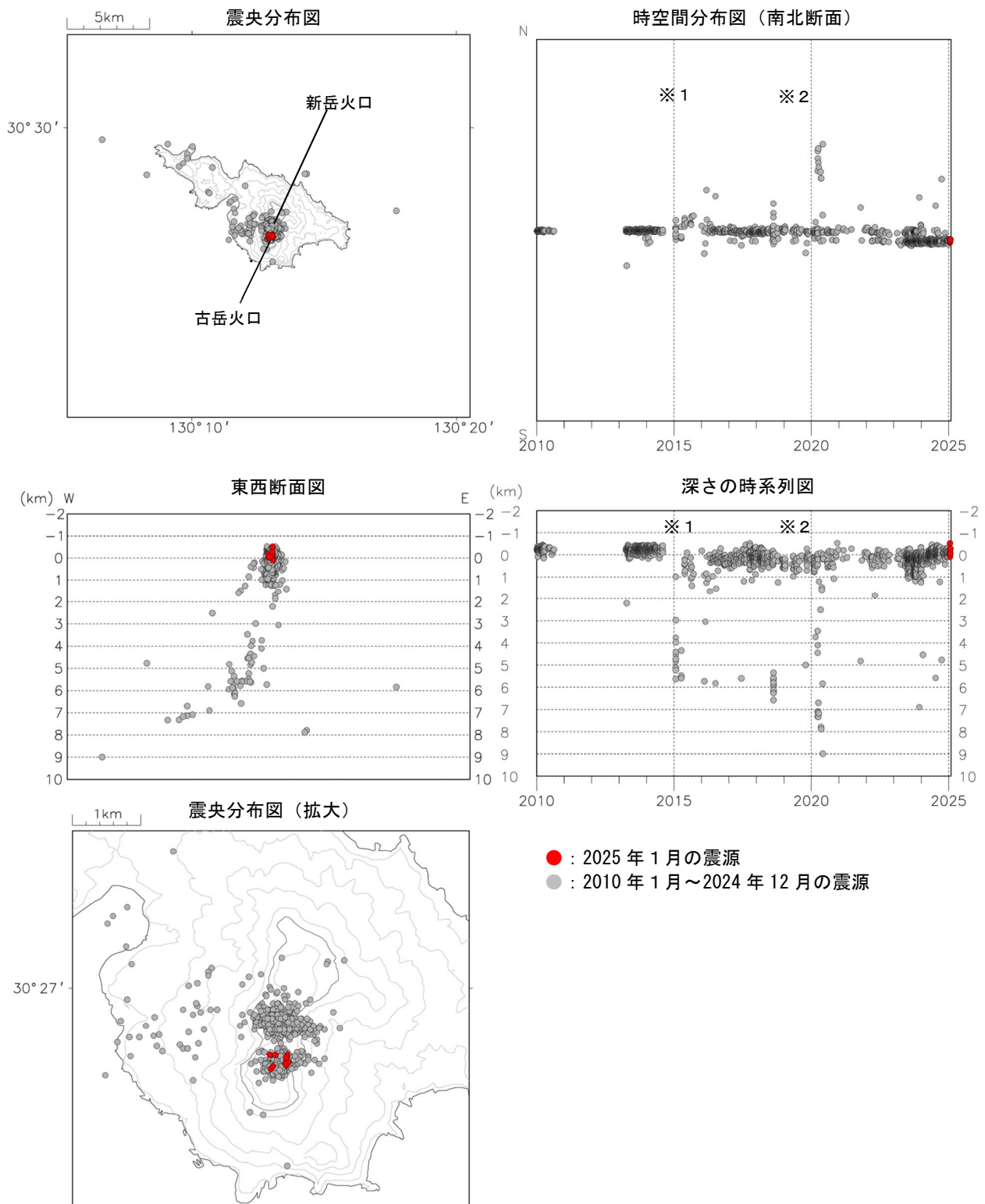
図5 口永良部島 震源分布図（2010年1月～2025年1月）
