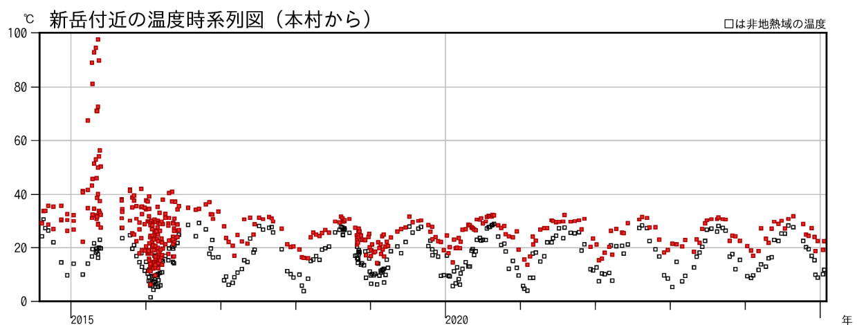
図 3-4 口永良部島 新岳火口西側割れ目付近の地熱域の温度時系列
