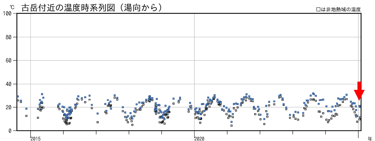
図 3-2 古岳火口付近の地熱域の温度時系列（2014 年 9 月～2025 年 1 月、湯向から観測）
