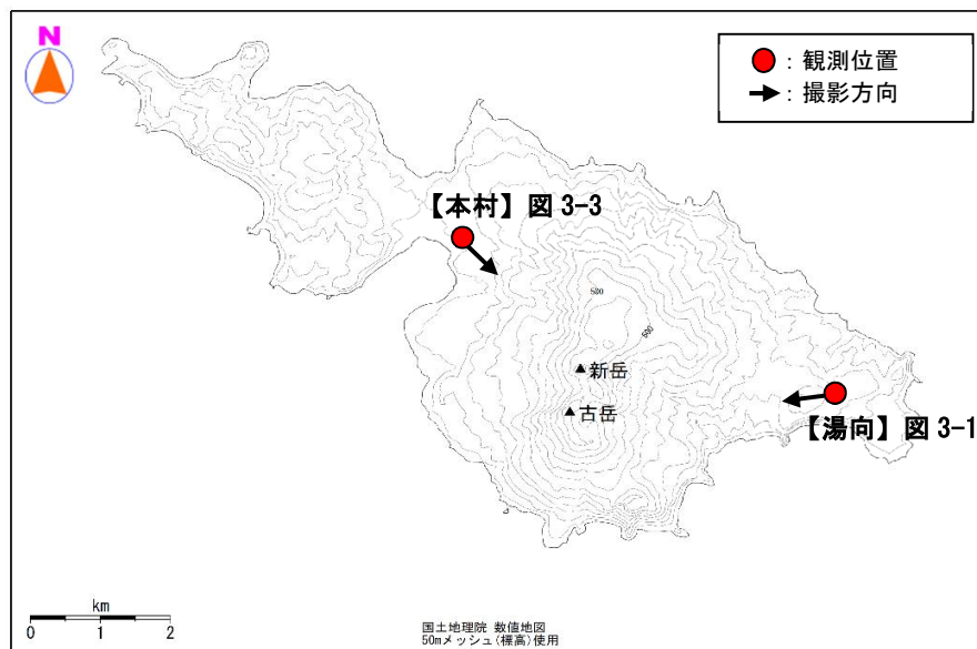
図2 口永良部島 観測位置及び撮影方向
